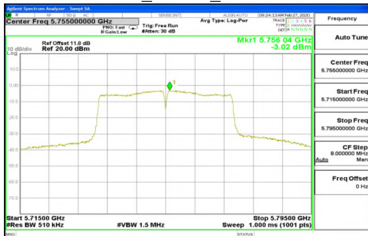
802.11n_40MHz_5755MHz
