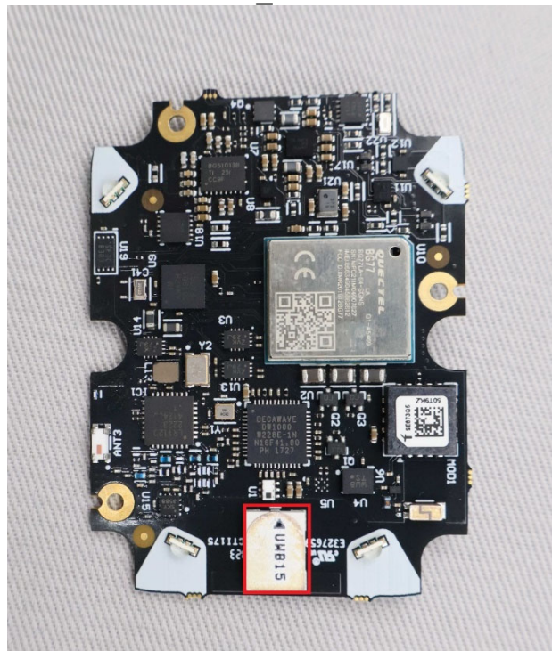
UWB_Antenna
