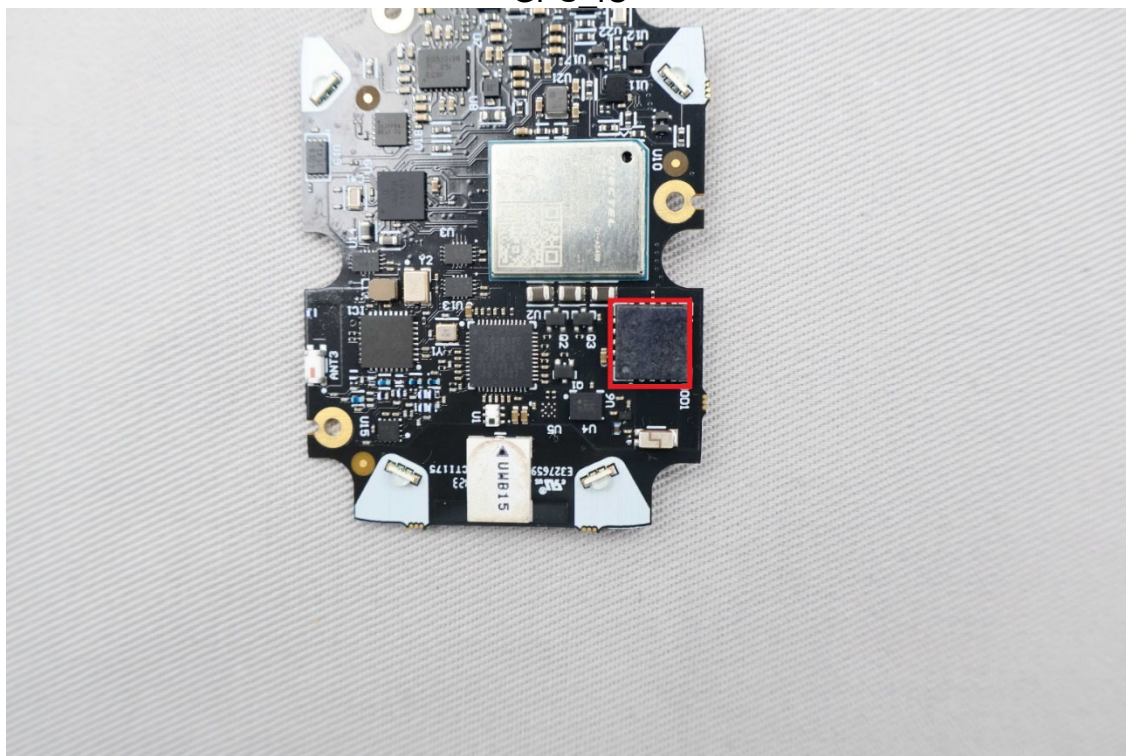
GPS IC
