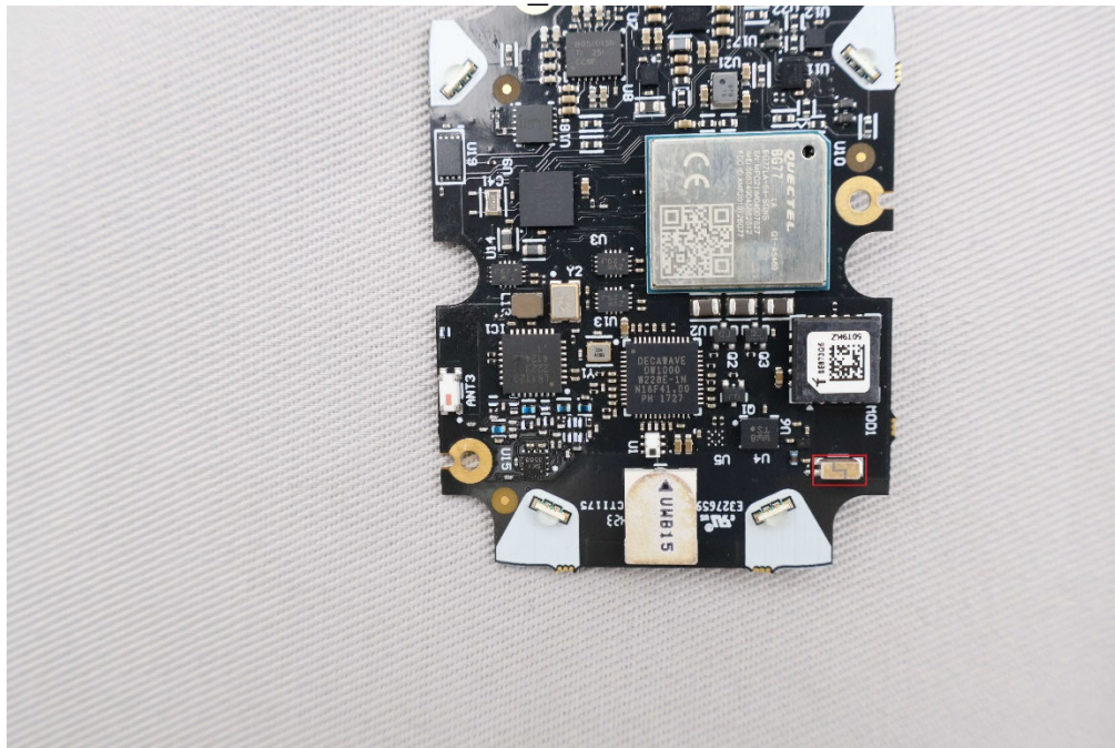
GPS_Antenna
