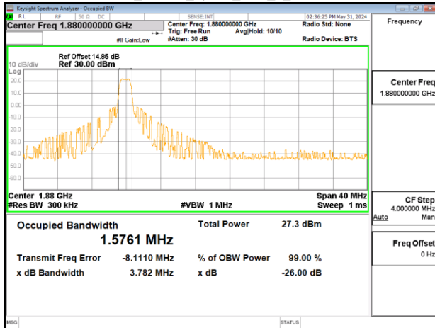
Band2_20MHz_QPSK_RB6_0_CH19100
