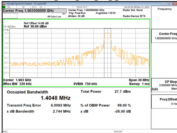
Band2_15MHz_QPSK_RB6_0_CH19125
