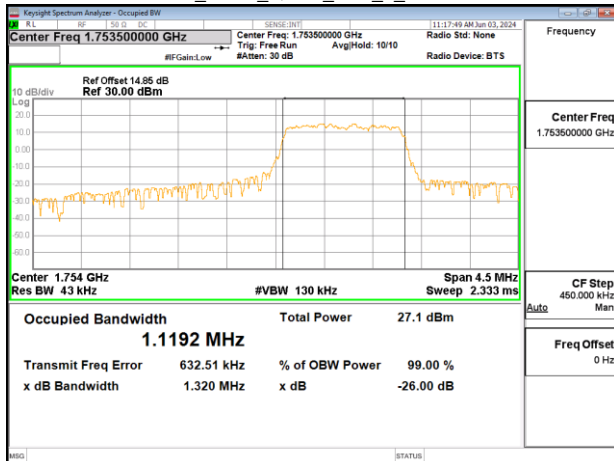
Band4_3MHz_QPSK_RB6_0_CH20385
