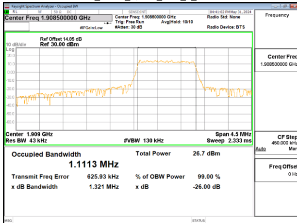
Band2_3MHz_QPSK_RB6_0_CH19185
