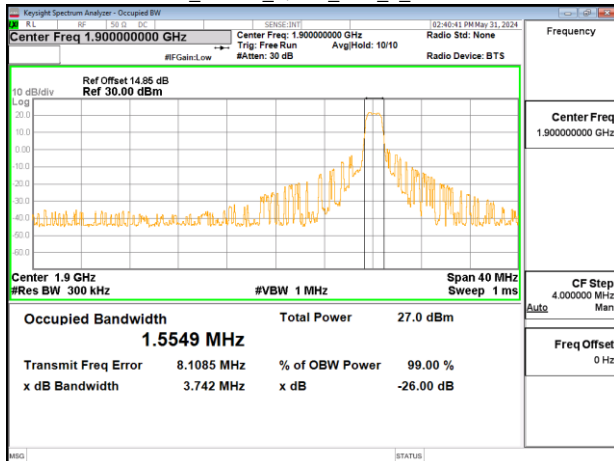
Band2_20MHz_QPSK_RB6_0_CH19100
