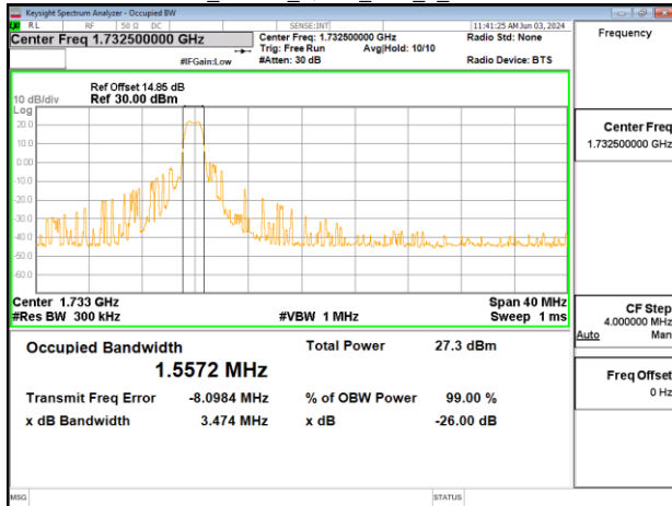
Band4_20MHz_QPSK_RB6_0_CH20300
