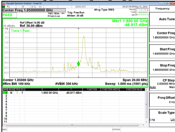
Band Edge_Band2_10MHz_QPSK_RB1_5_CH19150
