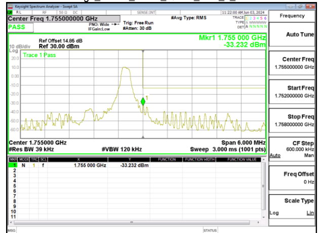
Band Edge_Band4_3MHz_QPSK_RB1_5_CH20385
