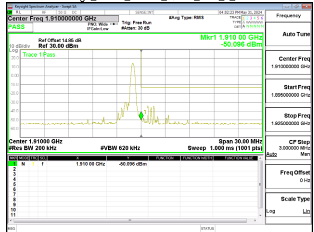
Band Edge_Band2_15MHz_QPSK_RB1_5_CH19125
