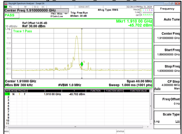
Band Edge_Band2_20MHz_QPSK_RB6_0_CH18700
