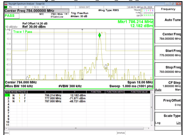
Band Edge_Band13_10MHz_QPSK_RB1_5_CH23230
