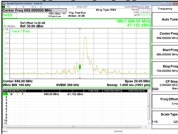
Band Edge_Band12_10MHz_QPSK_RB1_5_CH23130
