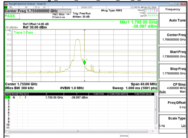
Band Edge_Band4_20MHz_QPSK_RB6_0_CH20300
