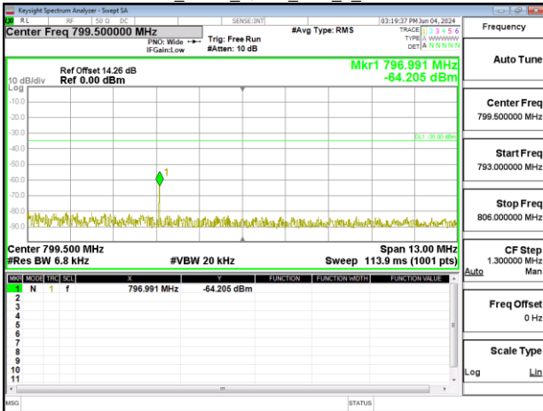
Band13_5MHz_QPSK_RB1_5_CH23255
