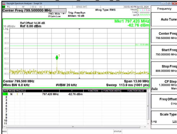
Band13_10MHz_QPSK_RB1_5_CH23230
