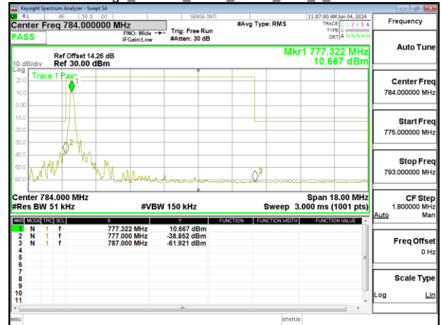
Band Edge_Band13_5MHz_QPSK_RB1_5_CH23255
