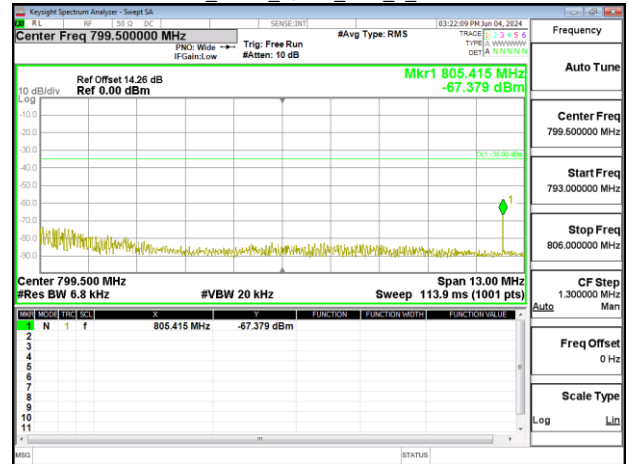
Band Edge_Band13_10MHz_QPSK_RB1_0_CH23230
