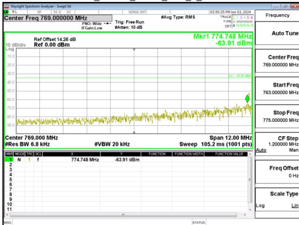
Band13_10MHz_QPSK_RB1_0_CH23230
