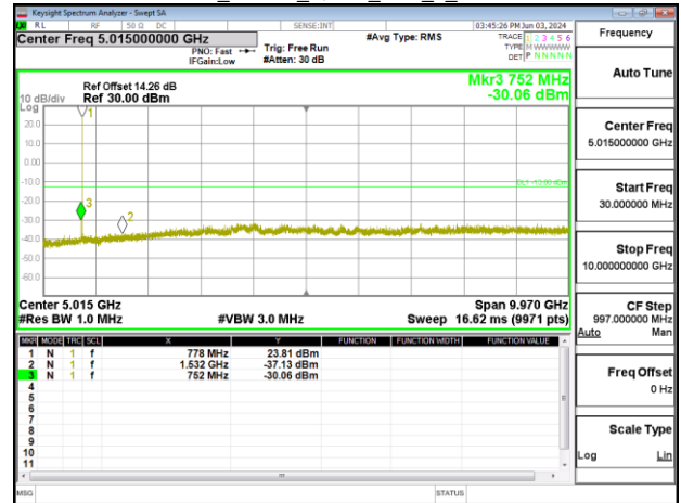
Band13_10MHz_QPSK_RB1_0_CH23230
