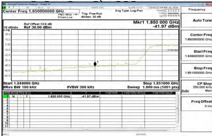
Cat M1 Band2 10MHz QPSK 6 0 LowCH18650-1855
