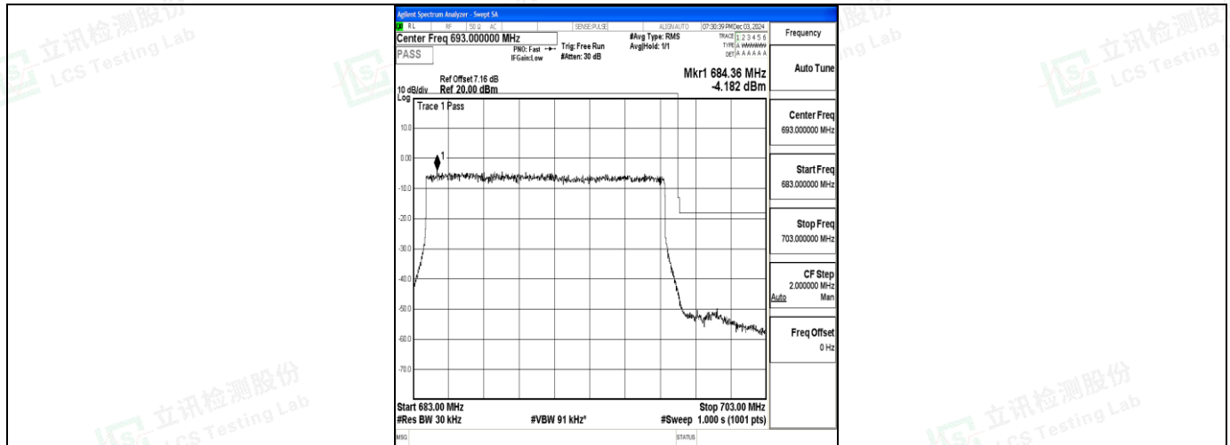
Band71_15MHz_QPSK_133397_75RB#0
