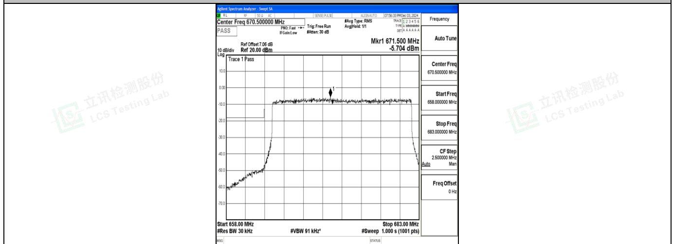
Band71_20MHz_QPSK_133222_100RB#0
