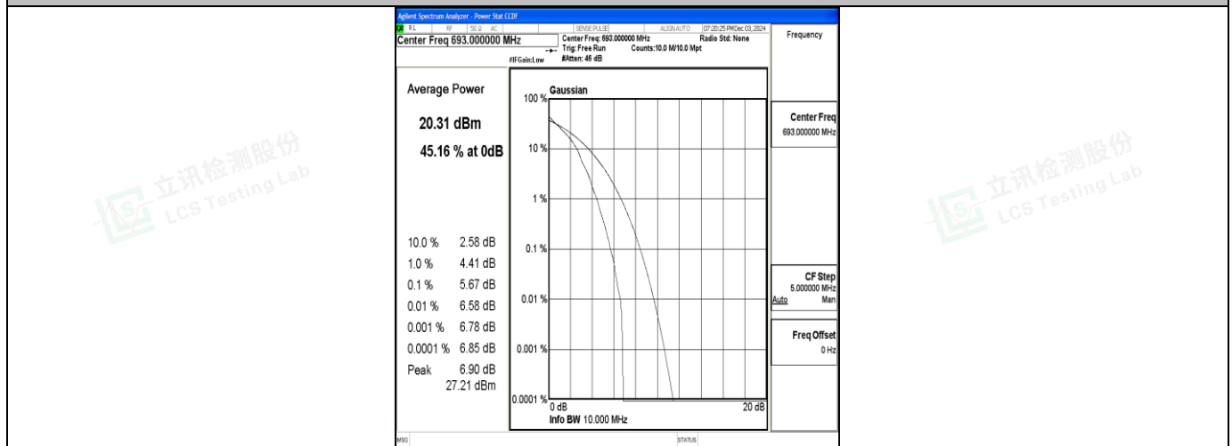
Band71-10MHz-QPSK-133422-1RB#0-PASS
