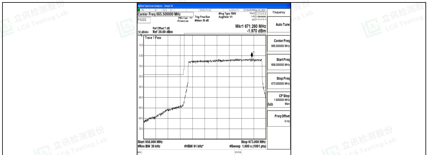
Band71_10MHz_QPSK_133172_50RB#0
