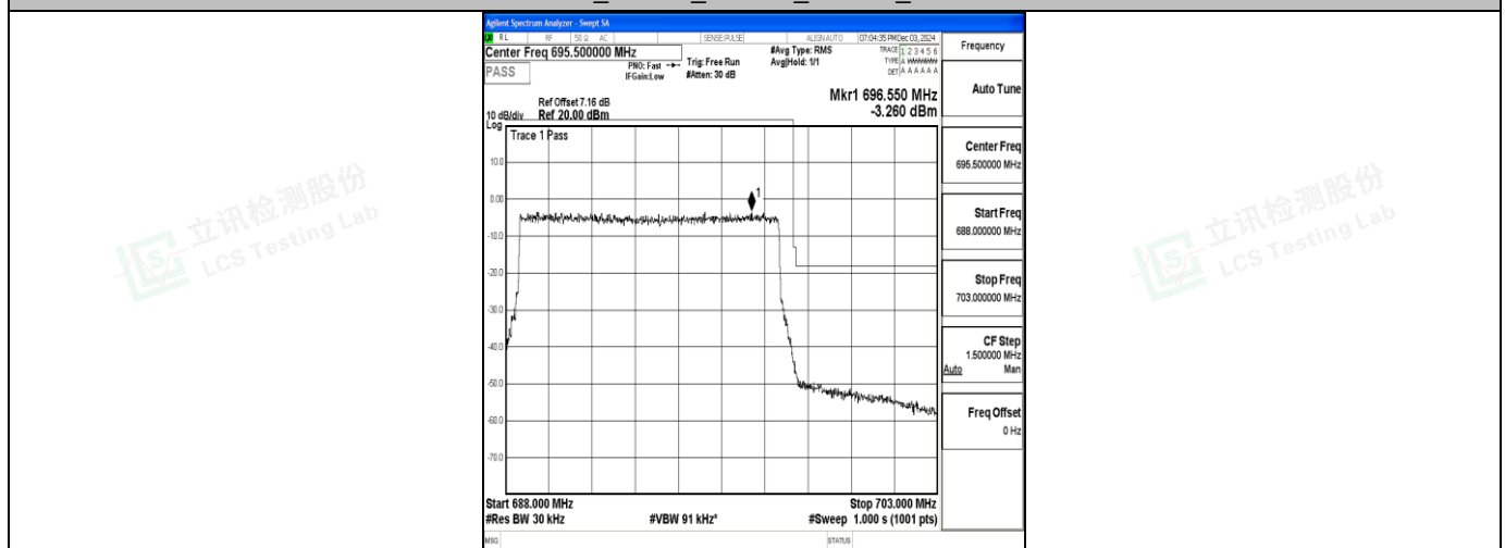
Band71_10MHz_QPSK_133422_50RB#0
