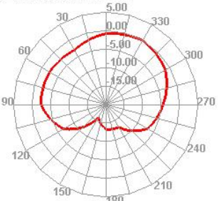
5250.000MHz E1
