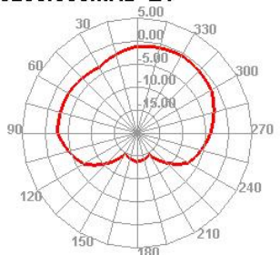
5200.000MHz E1
