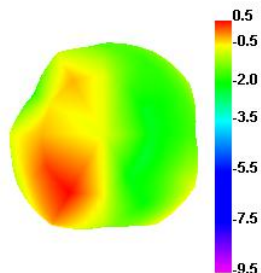
5200.000MHz E1
