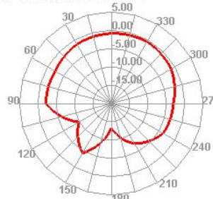
5250.000MHz E2
