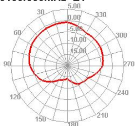
5150.000MHz E1
