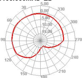
5150.000MHz E2
