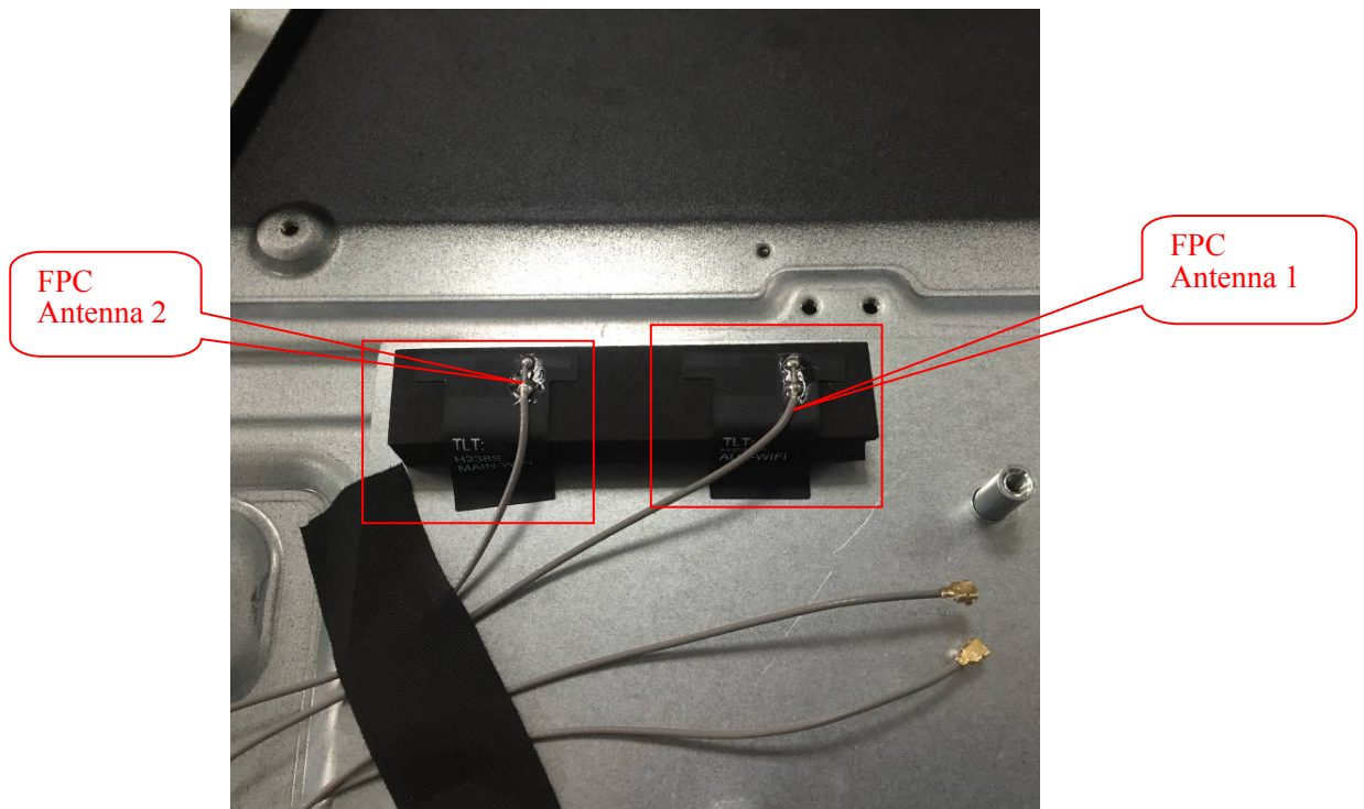
FPC Antennas
