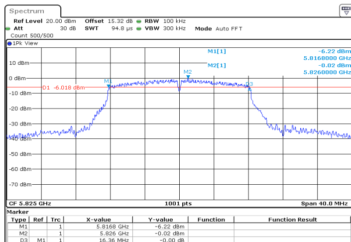
11A_Ant1_5825
