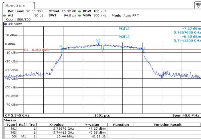
11A_Ant1_5745
