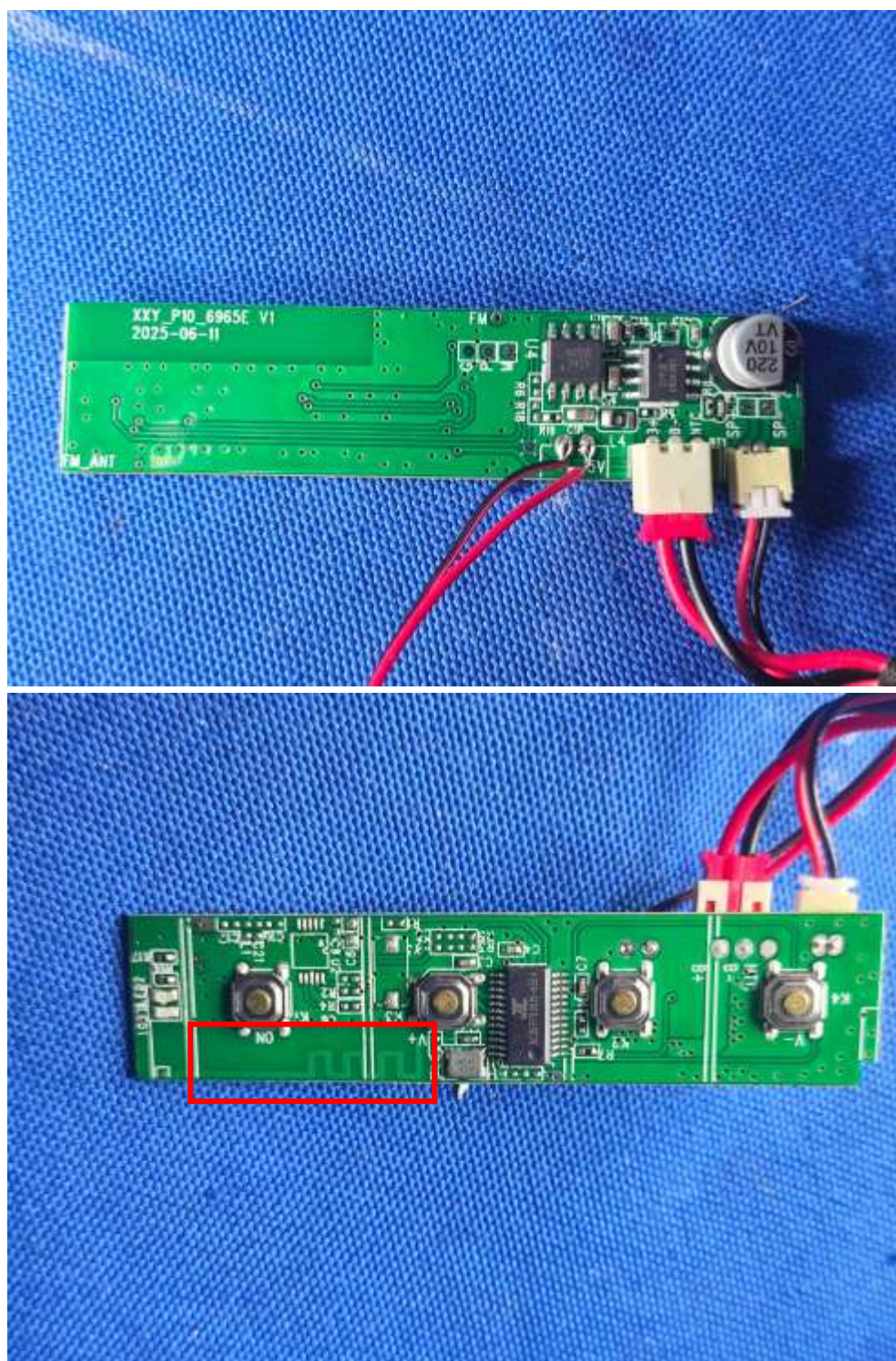
Antenna
