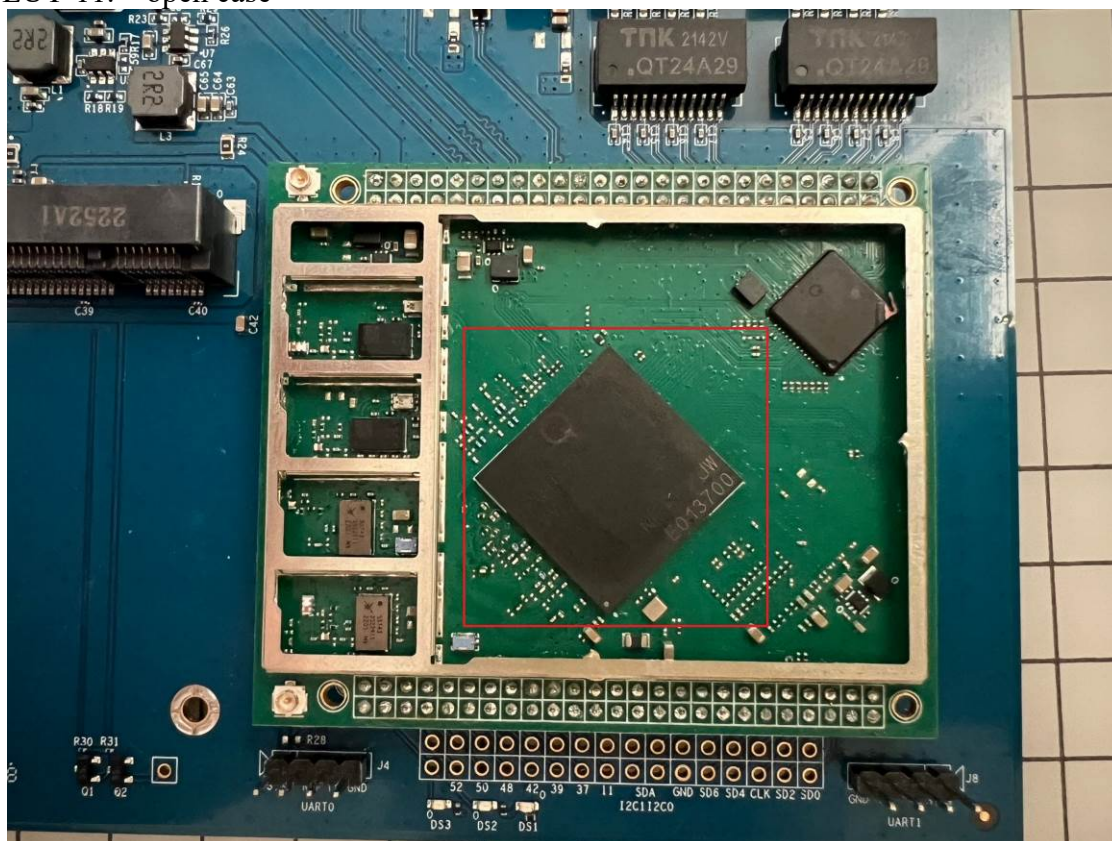
EUT-11. open case
