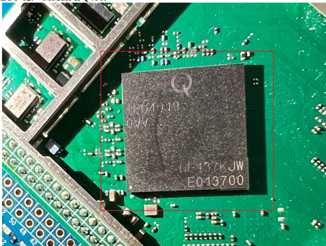
EUT-12. Module IPQ4019
