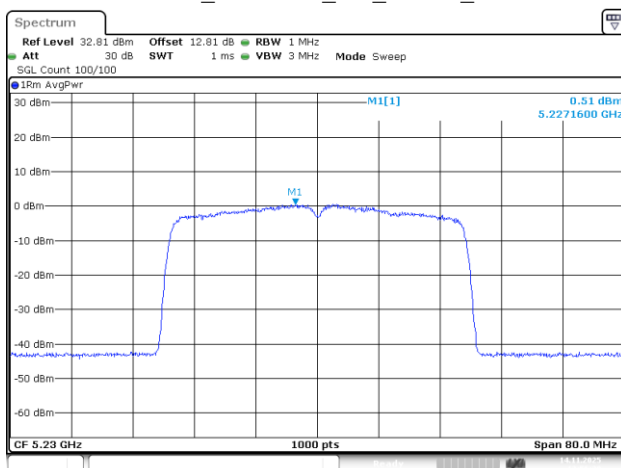
802.11be40_5230MHz_RU_484/65_Chain 1
