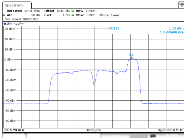
802.11be40_5230MHz_RU_52/44_Chain 0
