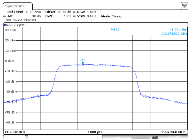
802.11a_5320MHz_Chain 3
