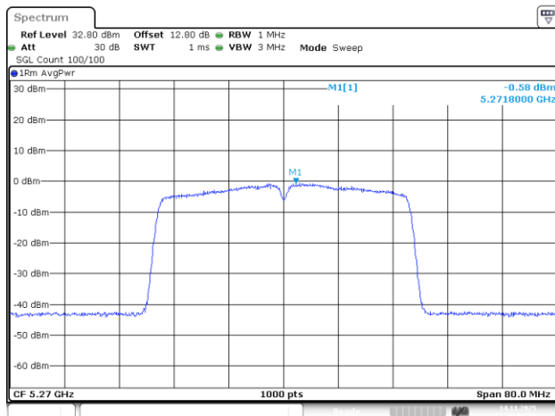
802.11ac40_5270MHz_Chain 2
