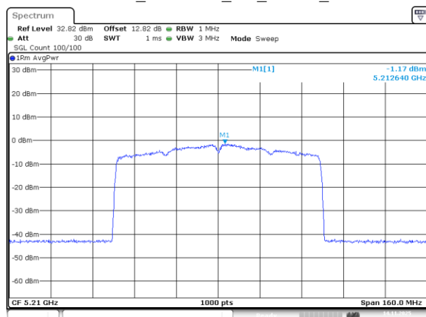
802.11be80_5210MHz_RU_996/67_Chain 2
