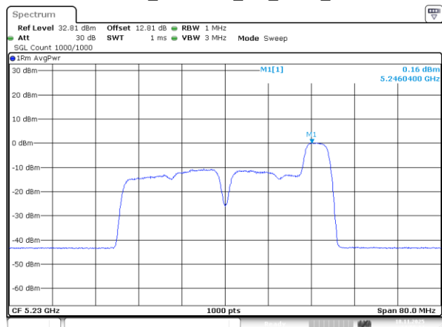
802.11be40_5230MHz_RU_52/44_Chain 3
