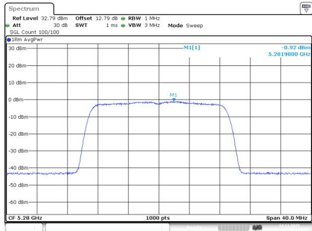
802.11ac20_5280MHz_Chain 0
