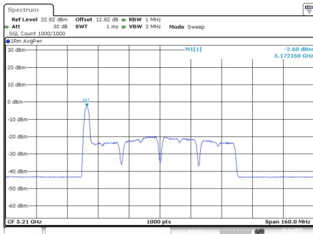
802.11be80_5210MHz_RU_26/0_Chain 0
