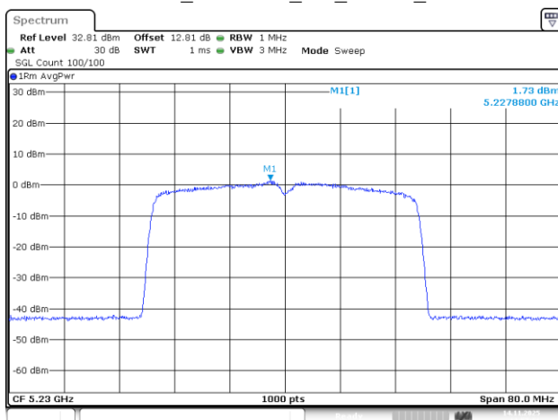
802.11be40_5230MHz_RU_484/65_Chain 2
