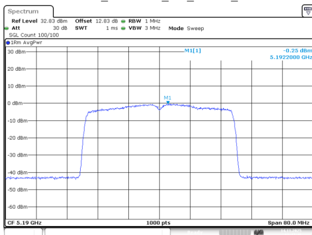
802.11be40_5190MHz_RU_484/65_Chain 0
