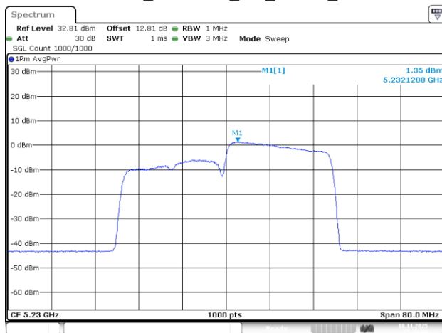
802.11be40_5230MHz_RU_242/62_Chain 2
