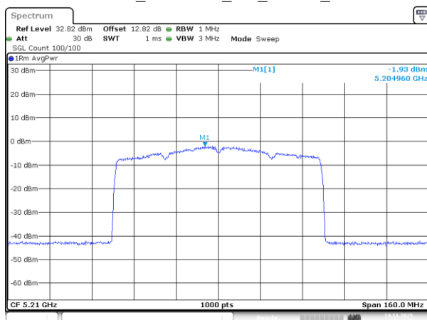
802.11be80_5210MHz_RU_996/67_Chain 1
