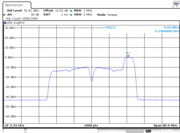
802.11be40_5230MHz_RU_52/44_Chain 1
