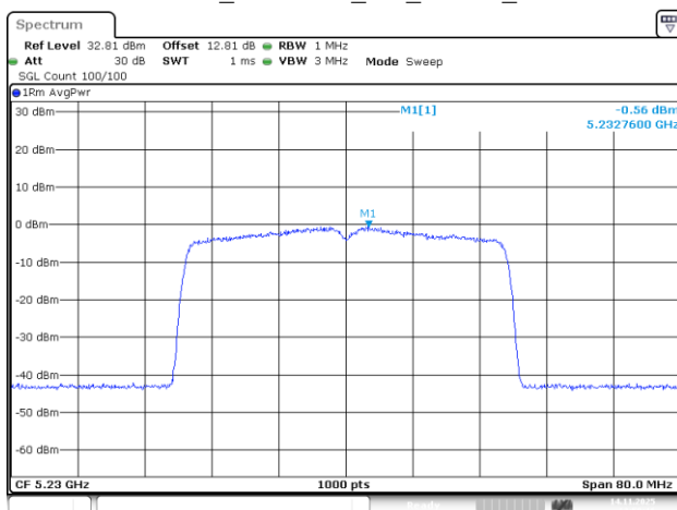
802.11be40_5230MHz_RU_484/65_Chain 3
