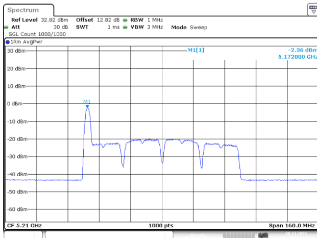
802.11be80_5210MHz_RU_26/0_Chain 1
