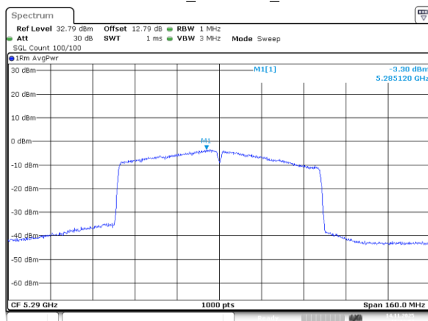
802.11ac80_5290MHz_Chain 3
