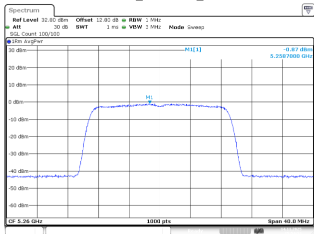
802.11ac20_5260MHz_Chain 1
