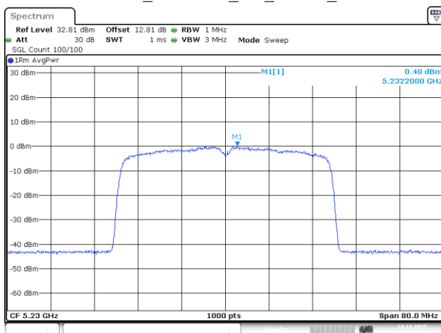
802.11be40_5230MHz_RU_484/65_Chain 0
