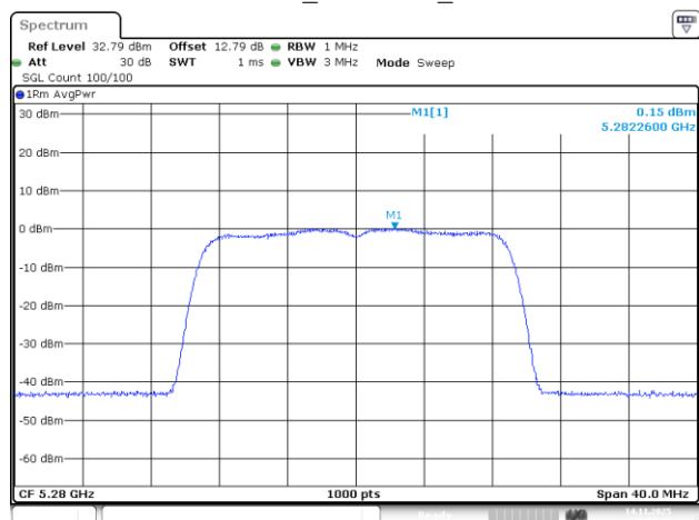
802.11ac20_5280MHz_Chain 2
