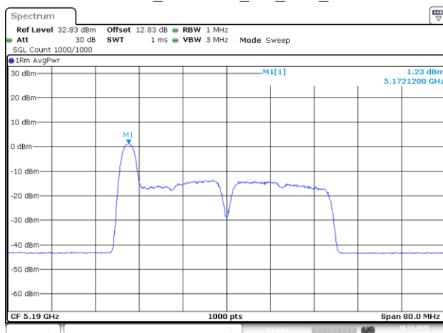
802.11be40_5190MHz_RU_26/0_Chain 2
