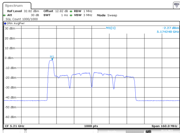
802.11be80_5210MHz_RU_52/37_Chain 1
