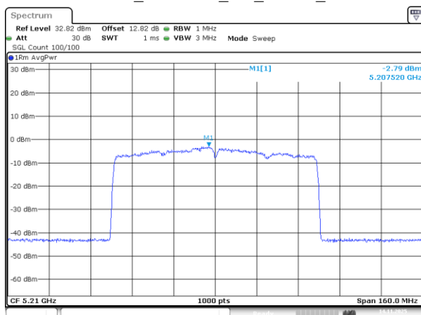
802.11be80_5210MHz_RU_996/67_Chain 3
