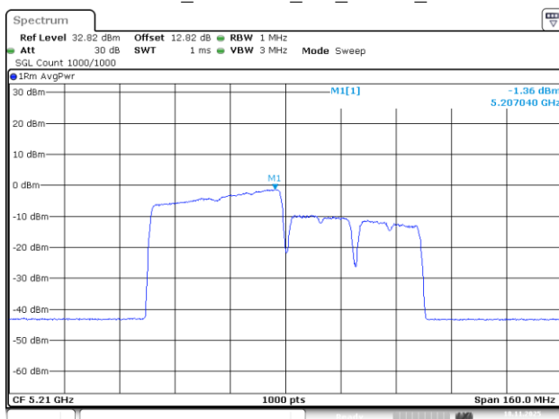
802.11be80_5210MHz_RU_484/65_Chain 1
