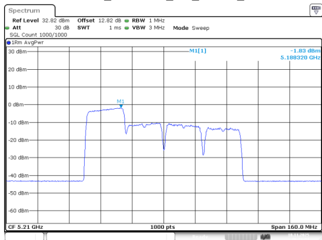
802.11be80_5210MHz_RU_242/61_Chain 3
