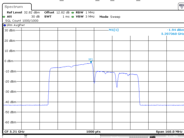
802.11be80_5210MHz_RU_484/65_Chain 0
