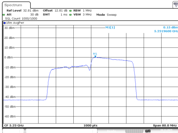
802.11be40_5230MHz_RU_242/62_Chain 0
