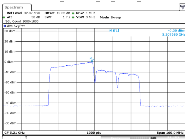
802.11be80_5210MHz_RU_484/65_Chain 2
