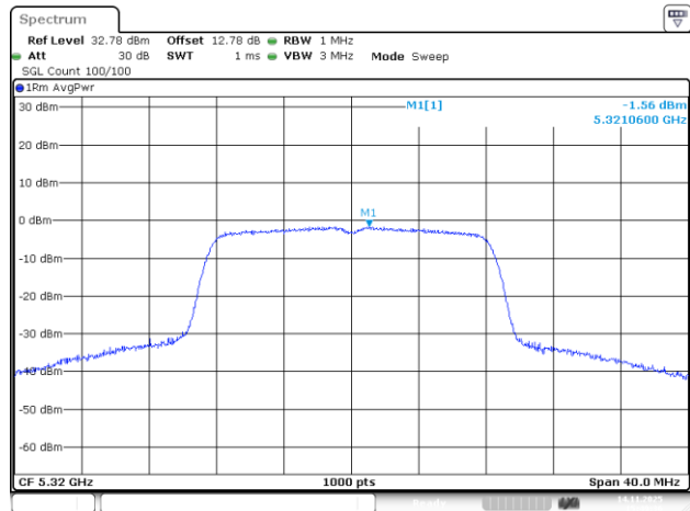
802.11a_5320MHz_Chain 1
