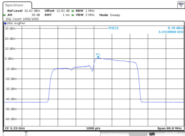
802.11be40_5230MHz_RU_242/62_Chain 1
