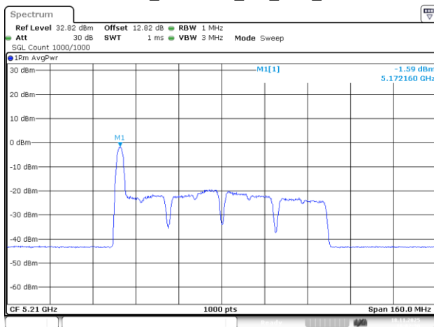
802.11be80_5210MHz_RU_26/0_Chain 3
