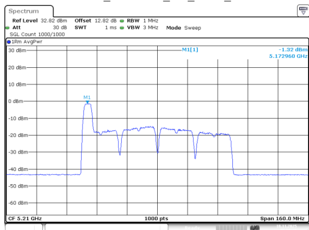
802.11be80_5210MHz_RU_52/37_Chain 3
