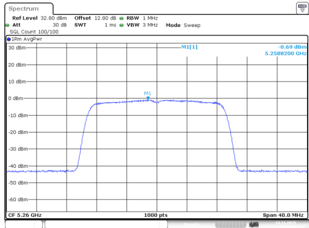
802.11ac20_5260MHz_Chain 3
