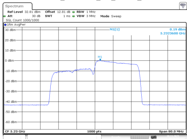
802.11be40_5230MHz_RU_242/62_Chain 3
