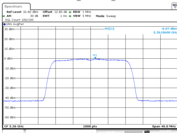
802.11ac20_5260MHz_Chain 2
