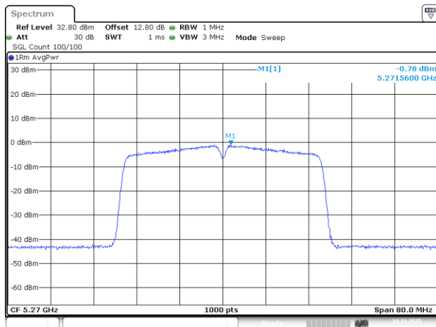
802.11ac40_5270MHz_Chain 0
