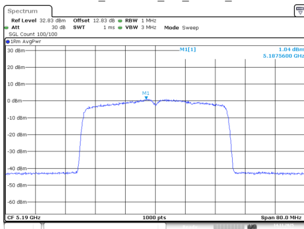
802.11be40_5190MHz_RU_484/65_Chain 2
