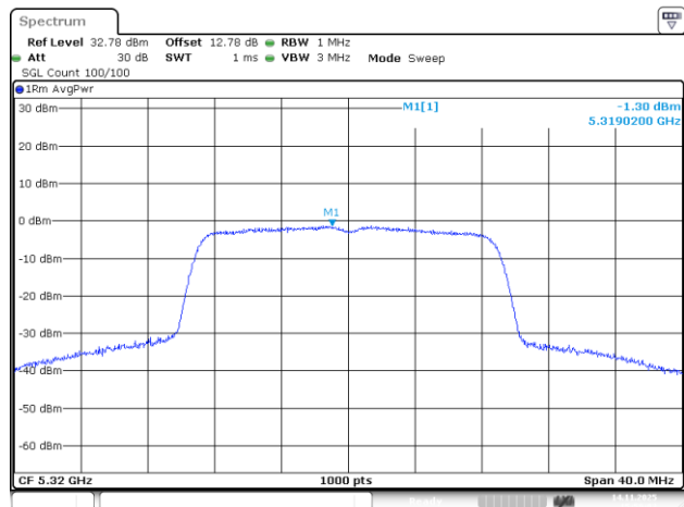
802.11ac20_5320MHz_Chain 1
