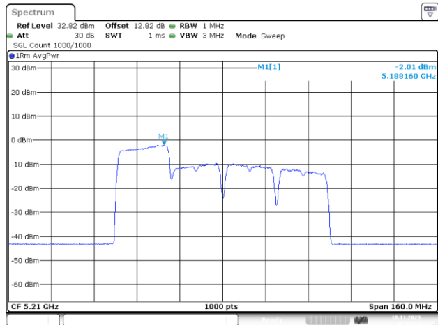
802.11be80_5210MHz_RU_242/61_Chain 1
