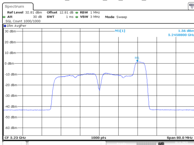
802.11be40_5230MHz_RU_52/44_Chain 2
