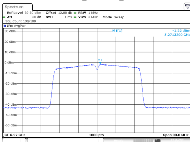
802.11ac40_5270MHz_Chain 1
