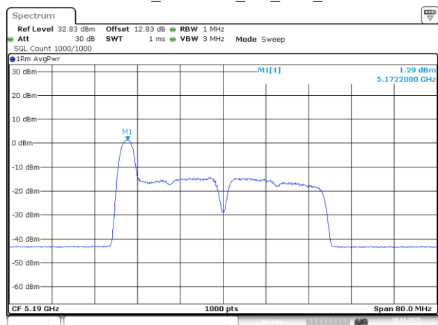
802.11be40_5190MHz_RU_26/0_Chain 3
