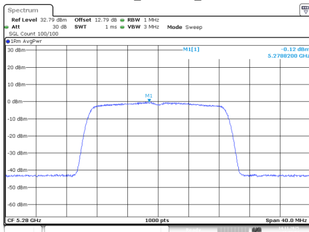
802.11ac20_5280MHz_Chain 3
