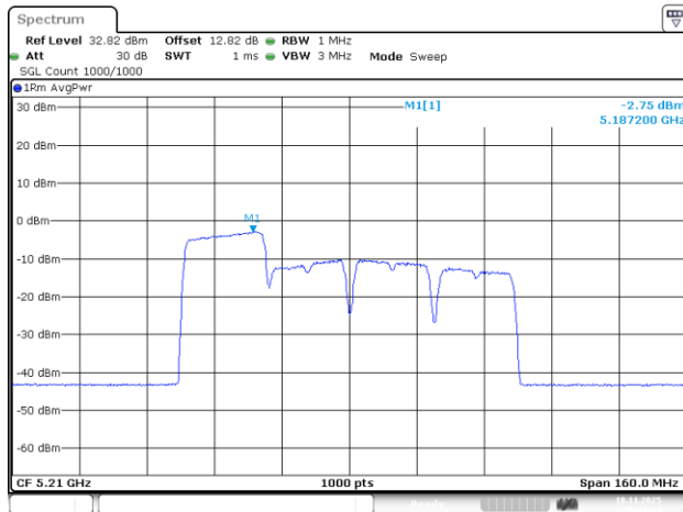
802.11be80_5210MHz_RU_242/61_Chain 0
