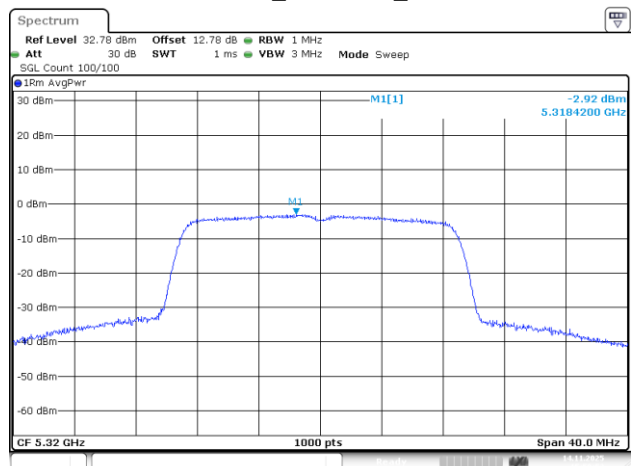
802.11ac20_5320MHz_Chain 3
