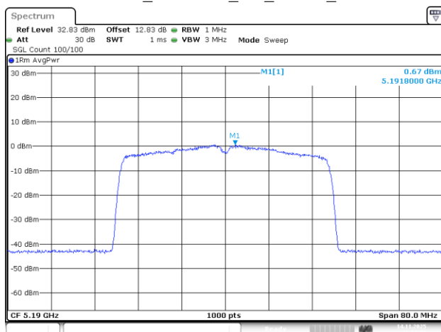
802.11be40_5190MHz_RU_484/65_Chain 3
