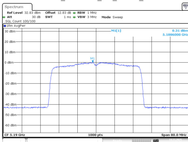
802.11be40_5190MHz_RU_484/65_Chain 1
