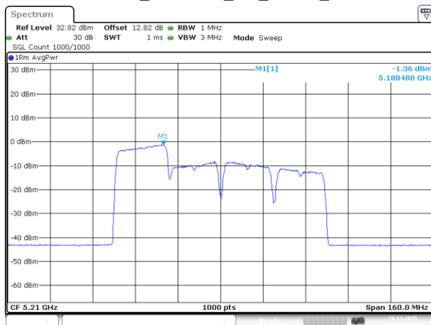
802.11be80_5210MHz_RU_242/61_Chain 2
