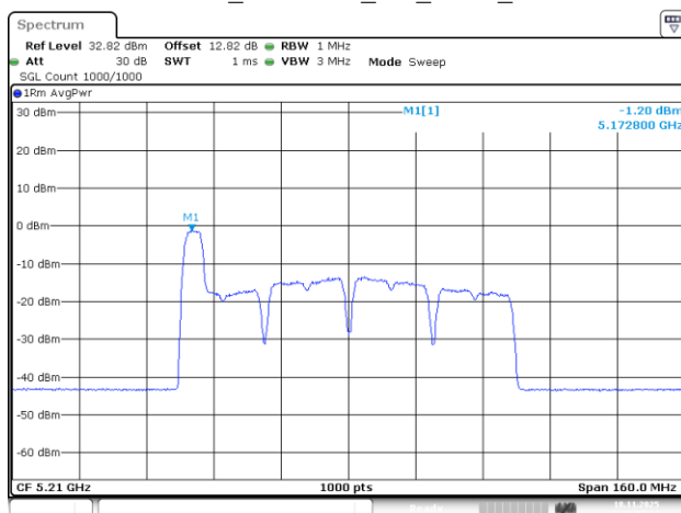
802.11be80_5210MHz_RU_52/37_Chain 2
