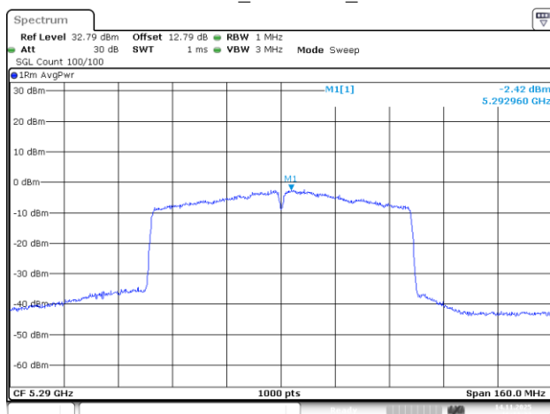
802.11ac80_5290MHz_Chain 2
