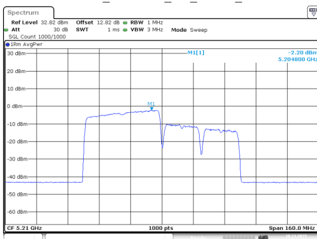
802.11be80_5210MHz_RU_484/65_Chain 3
