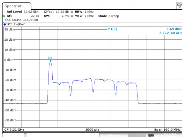
802.11be80_5210MHz_RU_26/0_Chain 2
