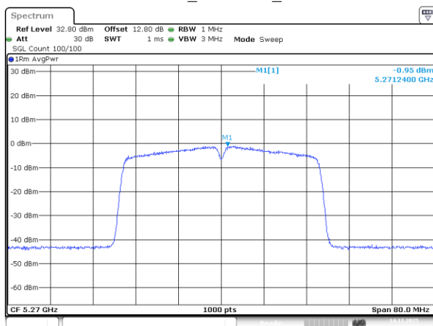
802.11ac40_5270MHz_Chain 3
