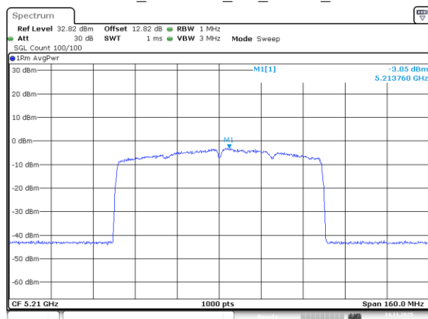
802.11be80_5210MHz_RU_996/67_Chain 0
