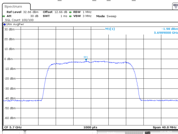
802.11be20_5700MHz_RU_242/61_Chain 1
