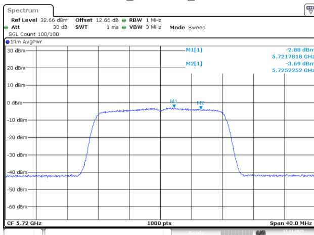
802.11a_5720MHz_Chain 3
