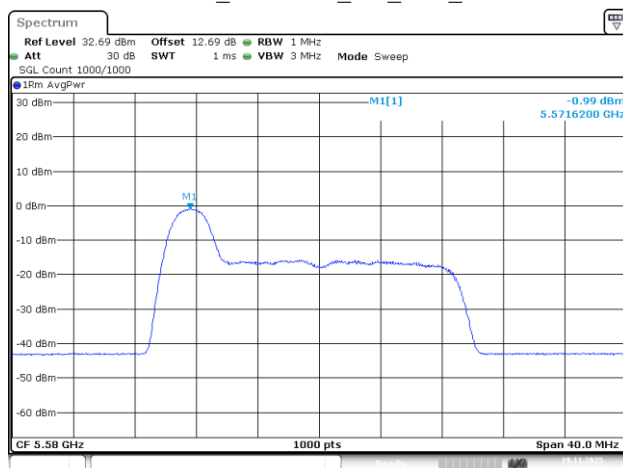
802.11be20_5580MHz_RU_26/0_Chain 2
