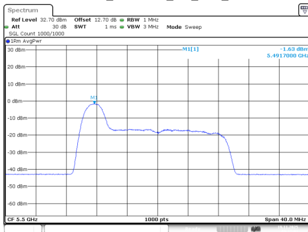
802.11be20_5500MHz_RU_26/0_Chain 1
