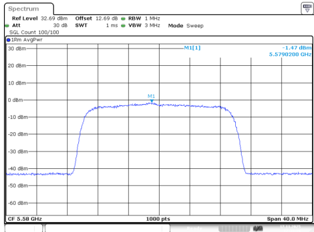
802.11be20_5580MHz_RU_242/61_Chain 3
