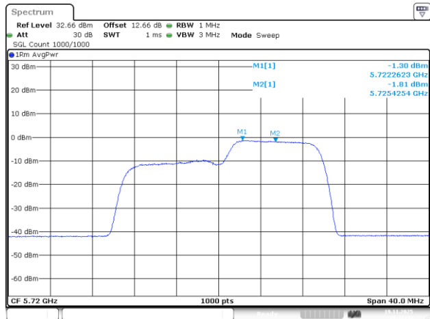
802.11be20_5720MHz_RU_106/54_Chain 0
