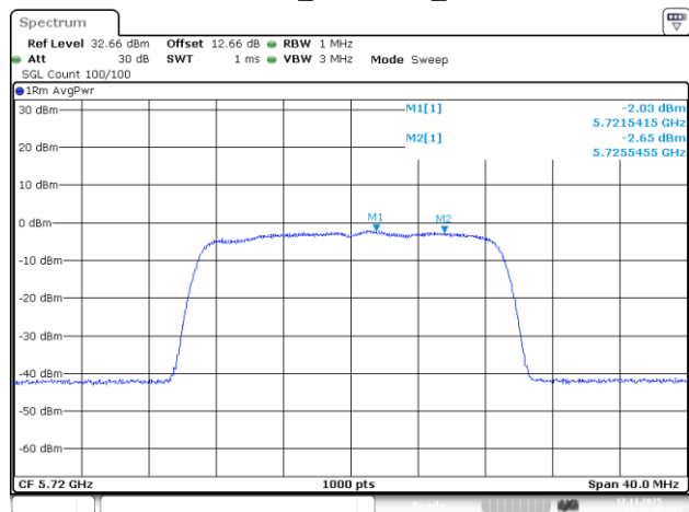
802.11ac20_5720MHz_Chain 2
