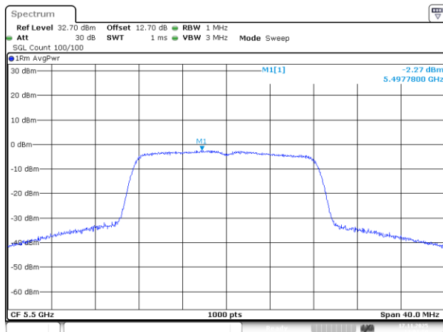
802.11a_5500MHz_Chain 1
