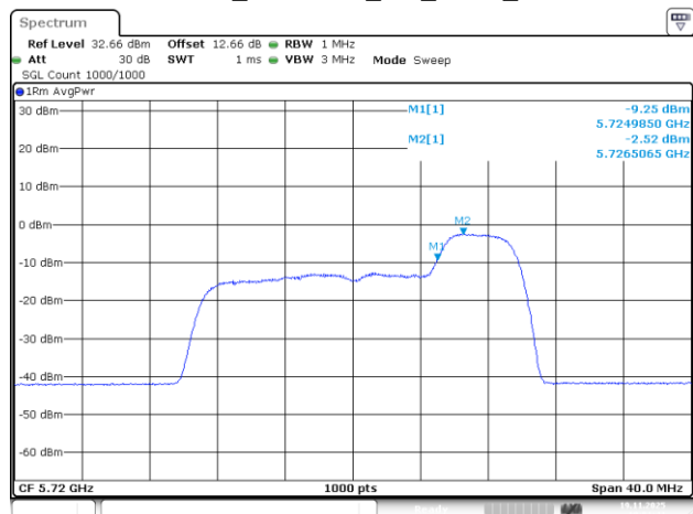
802.11be20_5720MHz_RU_52/40_Chain 3
