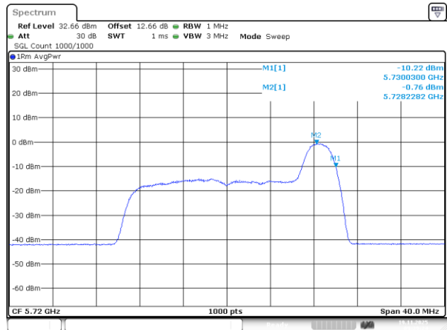
802.11be20_5720MHz_RU_26/8_Chain 2
