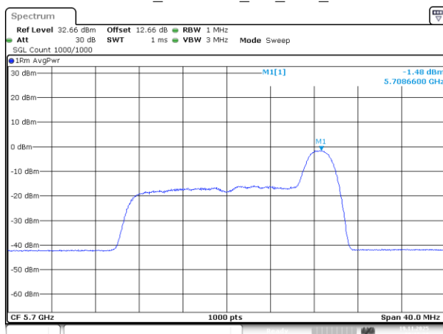
802.11be20_5700MHz_RU_26/8_Chain 1
