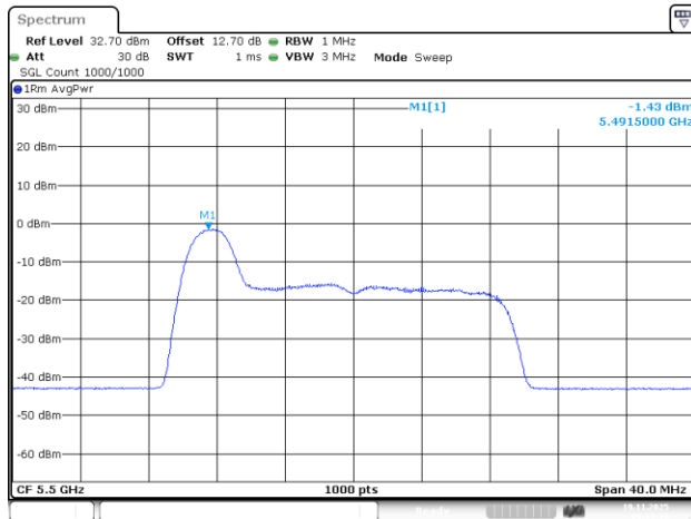
802.11be20_5500MHz_RU_26/0_Chain 0
