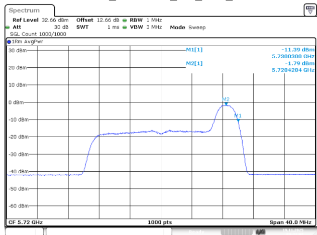
802.11be20_5720MHz_RU_26/8_Chain 3
