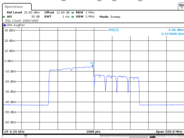
802.11be160_5250MHz_RU_996/67_Chain 0
