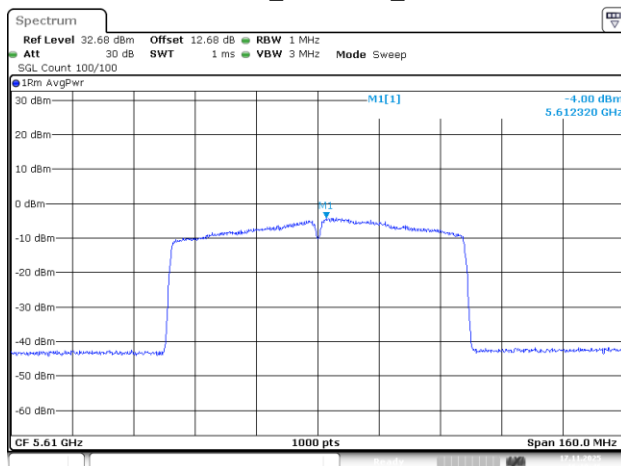
802.11ac80_5610MHz_Chain 3
