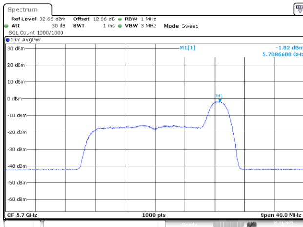
802.11be20_5700MHz_RU_26/8_Chain 0
