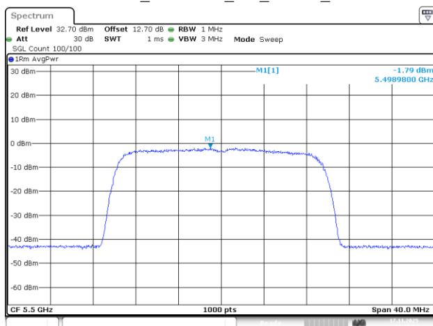
802.11be20_5500MHz_RU_242/61_Chain 1
