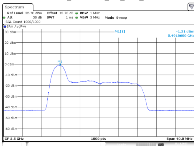
802.11be20_5500MHz_RU_26/0_Chain 2
