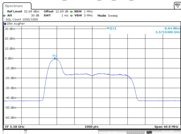
802.11be20_5580MHz_RU_26/0_Chain 1
