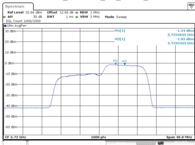
802.11be20_5720MHz_RU_106/54_Chain 1
