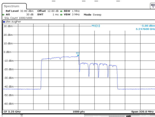
802.11be160_5250MHz_RU_996/67_Chain 2
