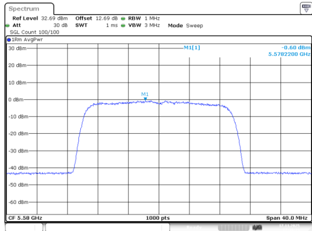
802.11be20_5580MHz_RU_242/61_Chain 2
