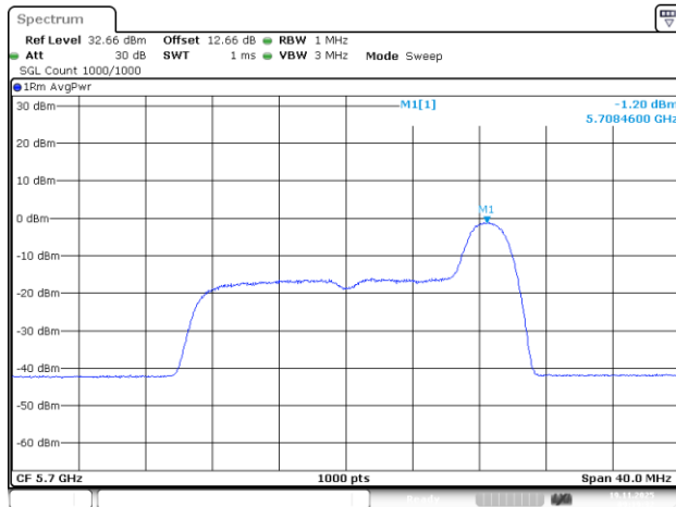
802.11be20_5700MHz_RU_26/8_Chain 2
