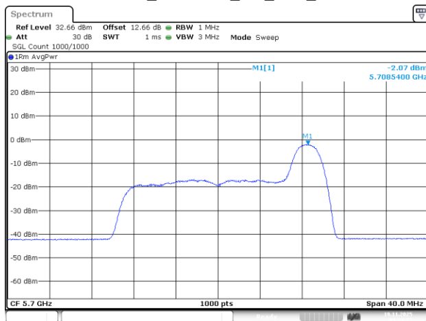
802.11be20_5700MHz_RU_26/8_Chain 3
