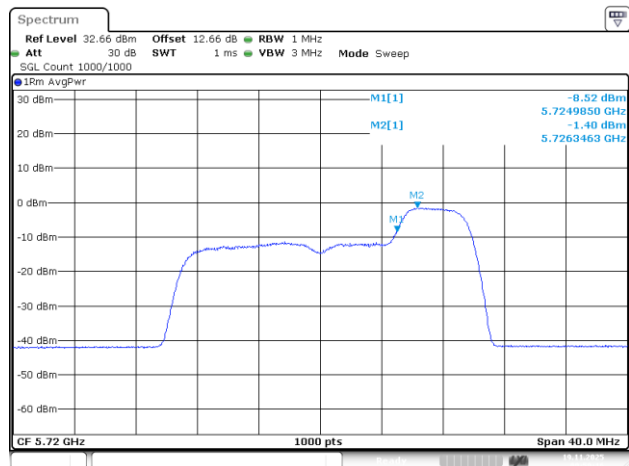
802.11be20_5720MHz_RU_52/40_Chain 0
