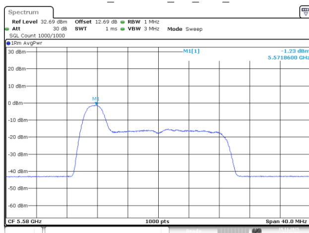
802.11be20_5580MHz_RU_26/0_Chain 3
