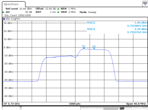
802.11be20_5720MHz_RU_106/54_Chain 2
