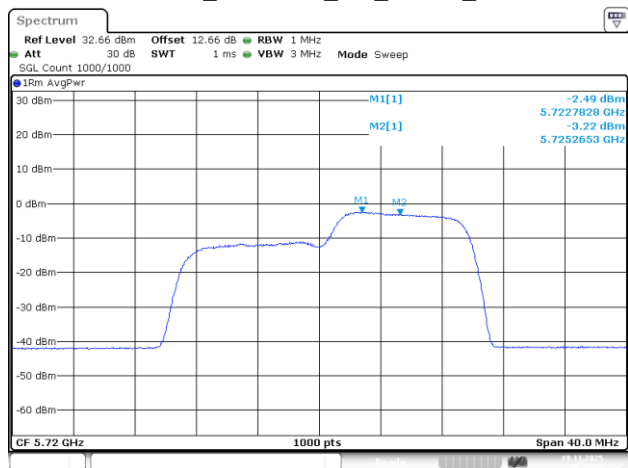
802.11be20_5720MHz_RU_106/54_Chain 3
