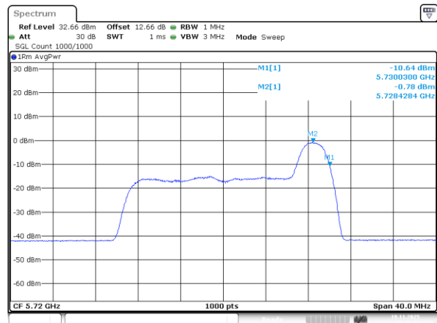
802.11be20_5720MHz_RU_26/8_Chain 0
