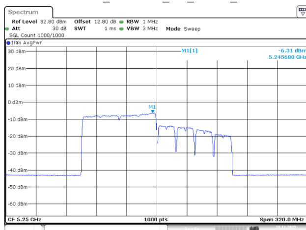
802.11be160_5250MHz_RU_996/67_Chain 3
