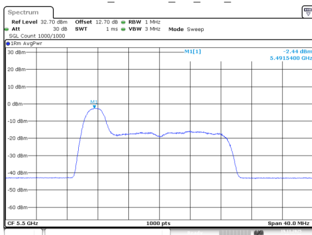
802.11be20_5500MHz_RU_26/0_Chain 3
