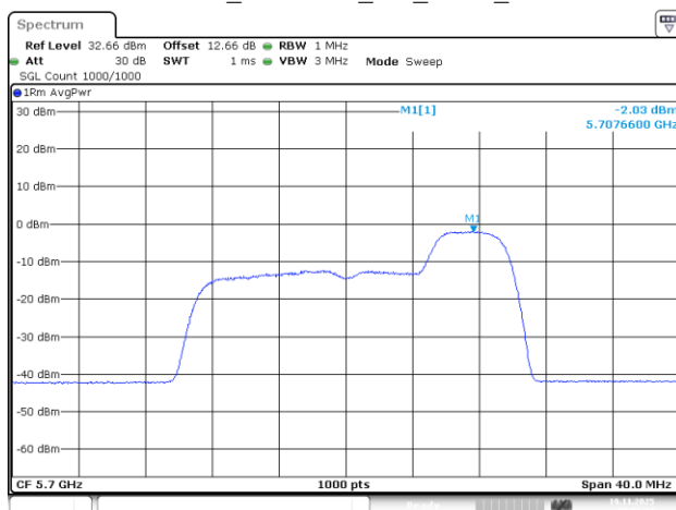
802.11be20_5700MHz_RU_52/40_Chain 1
