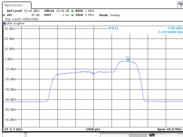
802.11be20_5700MHz_RU_52/40_Chain 2
