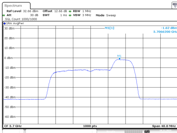
802.11be20_5700MHz_RU_52/40_Chain 0
