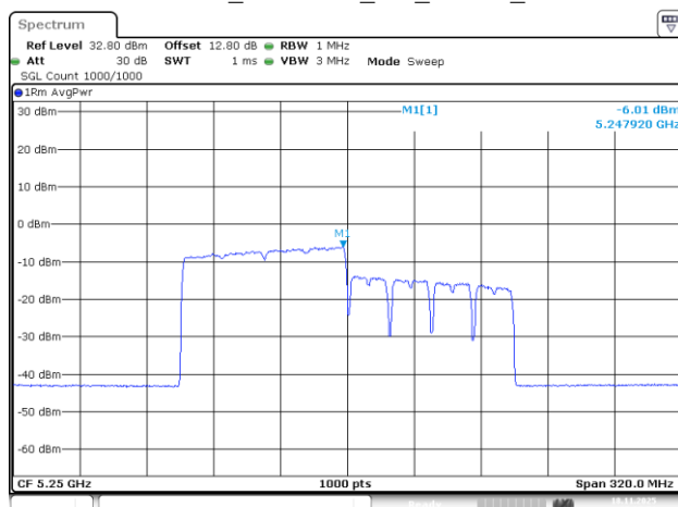
802.11be160_5250MHz_RU_996/67_Chain 1
