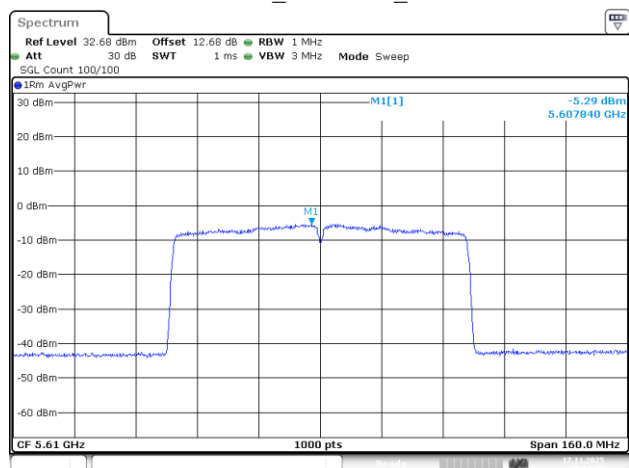
802.11ac80_5610MHz_Chain 2
