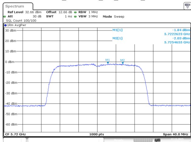
802.11be20_5720MHz_RU_242/61_Chain 2
