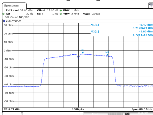
802.11ac40_5710MHz_Chain 3
