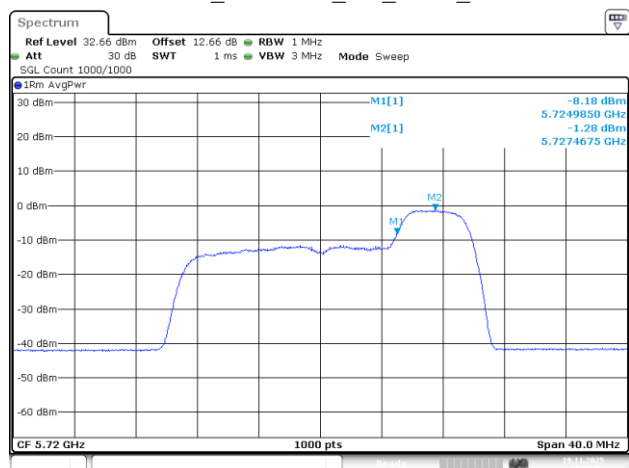
802.11be20_5720MHz_RU_52/40_Chain 1
