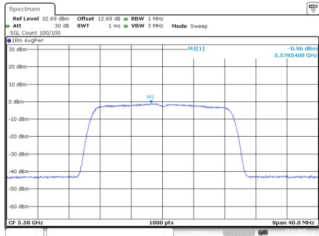
802.11ac20_5580MHz_Chain 2
