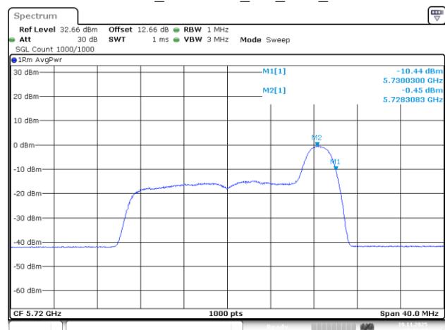
802.11be20_5720MHz_RU_26/8_Chain 1
