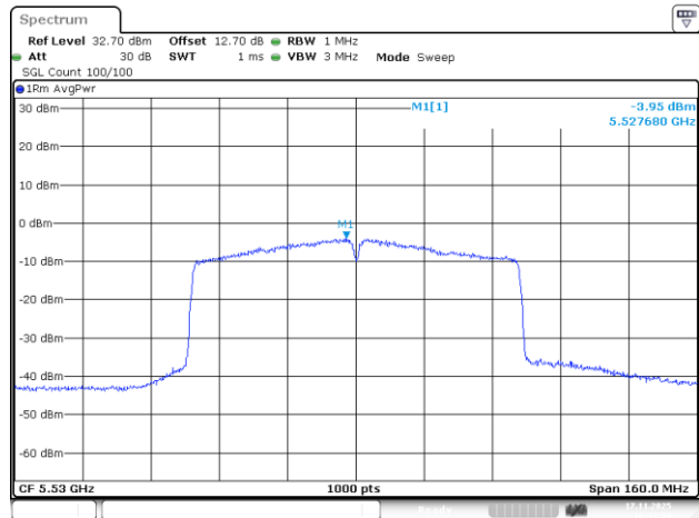
802.11ac80_5530MHz_Chain 3
