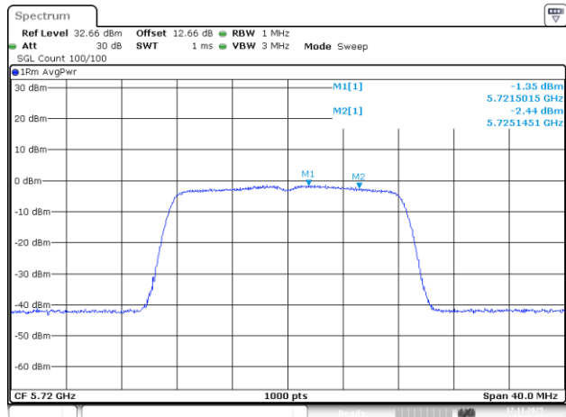
802.11a_5720MHz_Chain 0
