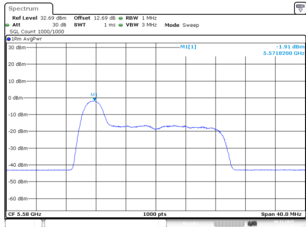
802.11be20_5580MHz_RU_26/0_Chain 0
