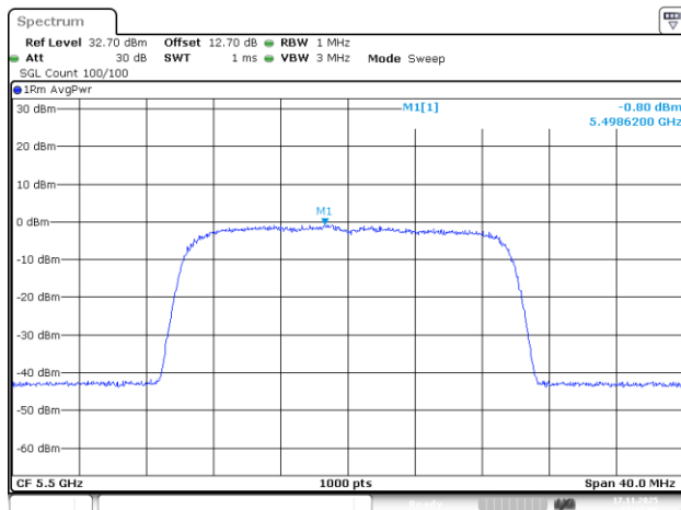
802.11be20_5500MHz_RU_242/61_Chain 0
