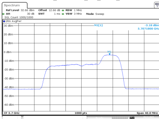
802.11be20_5700MHz_RU_52/40_Chain 3
