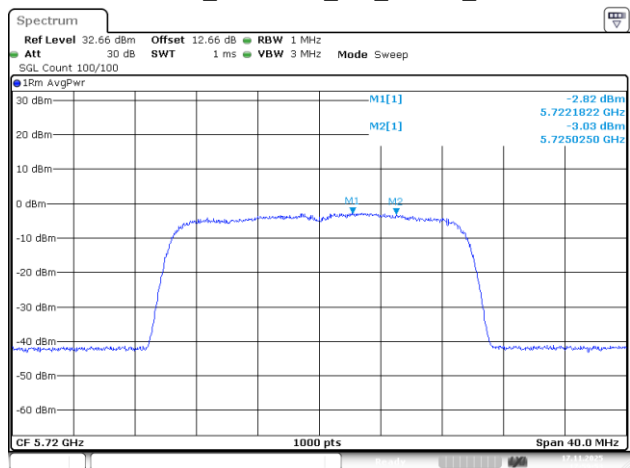
802.11be20_5720MHz_RU_242/61_Chain 3
