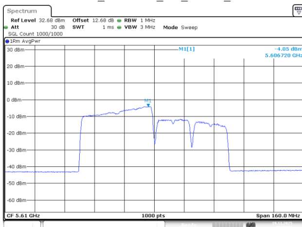
802.11be80_5610MHz_RU_484/65_Chain 3
