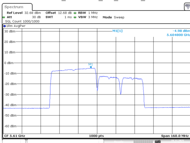
802.11be80_5610MHz_RU_484/65_Chain 2
