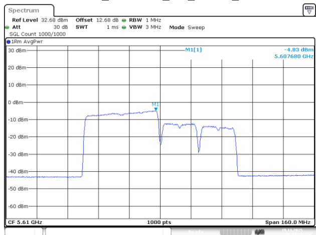
802.11be80_5610MHz_RU_484/65_Chain 1
