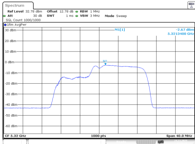
802.11be20_5320MHz_RU_26&106_MRU2_Chain 1
