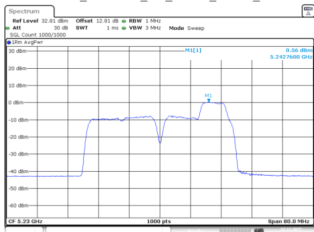
802.11be40_5230MHz_RU_26&52_MRU6_Chain 3
