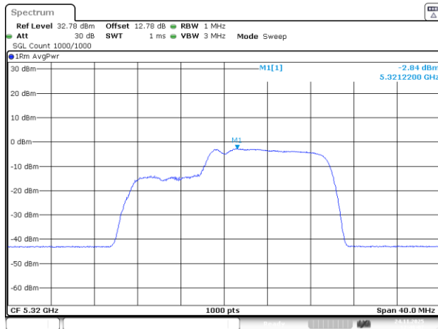
802.11be20_5320MHz_RU_26&106_MRU2_Chain 2
