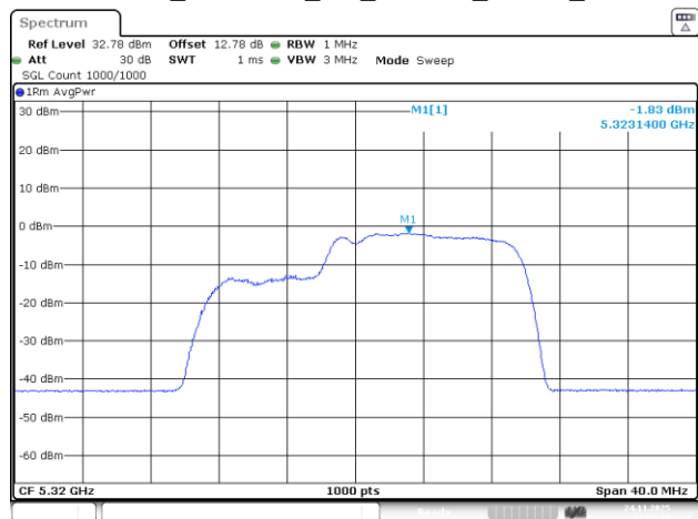
802.11be20_5320MHz_RU_26&106_MRU2_Chain 3
