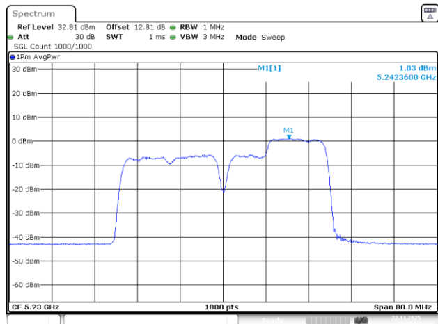
802.11be40_5230MHz_RU_26&106_MRU4_Chain 2
