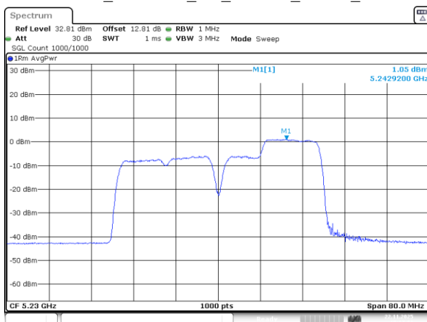
802.11be40_5230MHz_RU_26&106_MRU4_Chain 0
