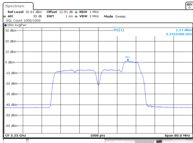
802.11be40_5230MHz_RU_26&52_MRU6_Chain 2
