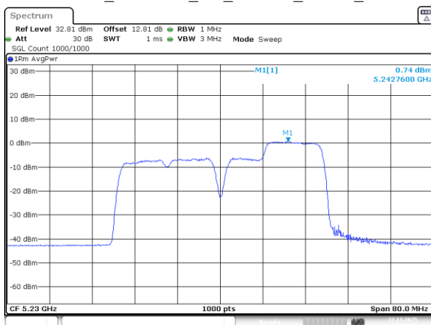
802.11be40_5230MHz_RU_26&106_MRU4_Chain 1
