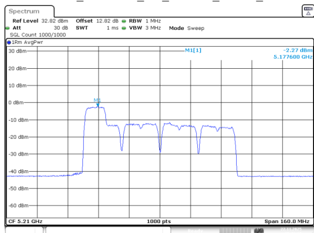
802.11be80_5210MHz_RU_26&106_MRU1_Chain 3
