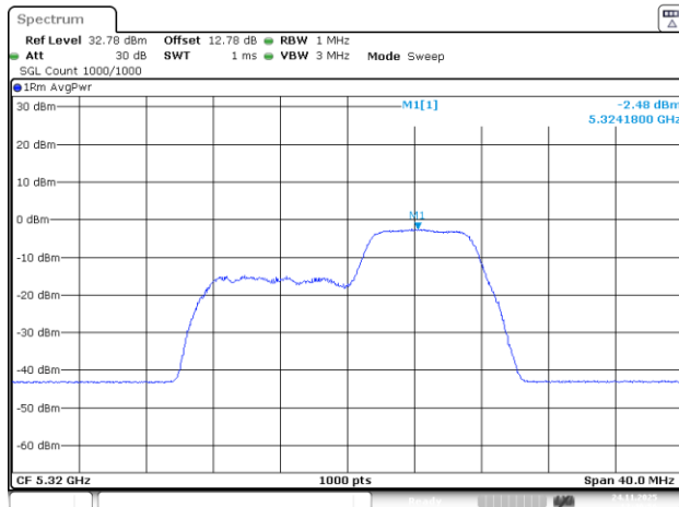
802.11be20_5320MHz_RU_26&52_MRU3_Chain 2
