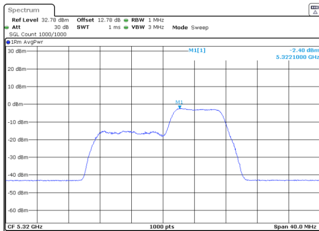
802.11be20_5320MHz_RU_26&52_MRUI_Chain 0
