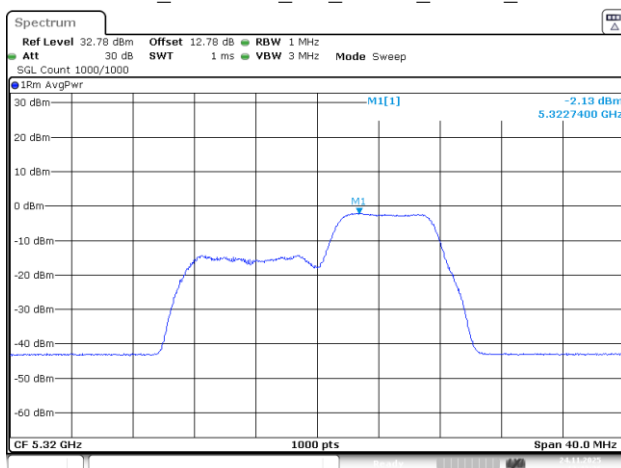
802.11be20_5320MHz_RU_26&52_MRU3_Chain 1
