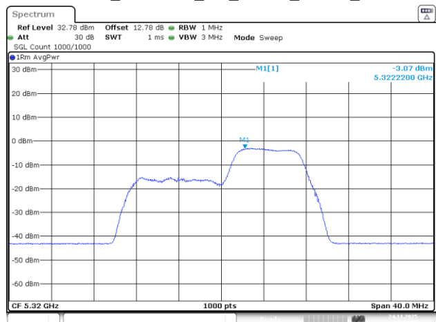
802.11be20_5320MHz_RU_26&52_MRU3_Chain 3
