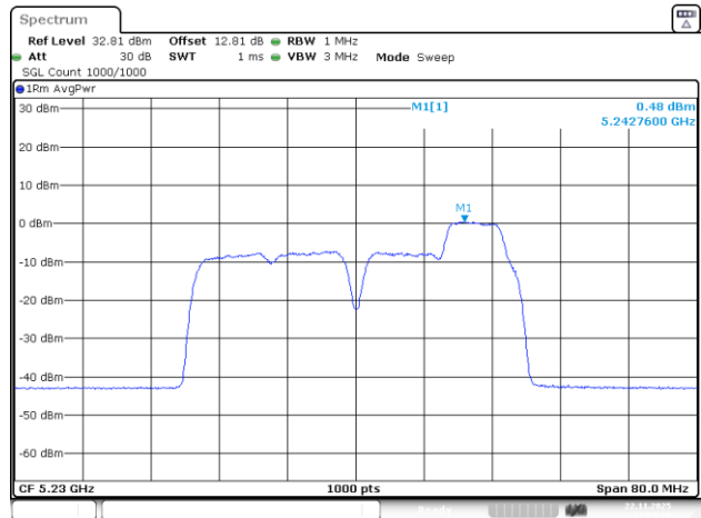
802.11be40_5230MHz_RU_26&52_MRU6_Chain 0
