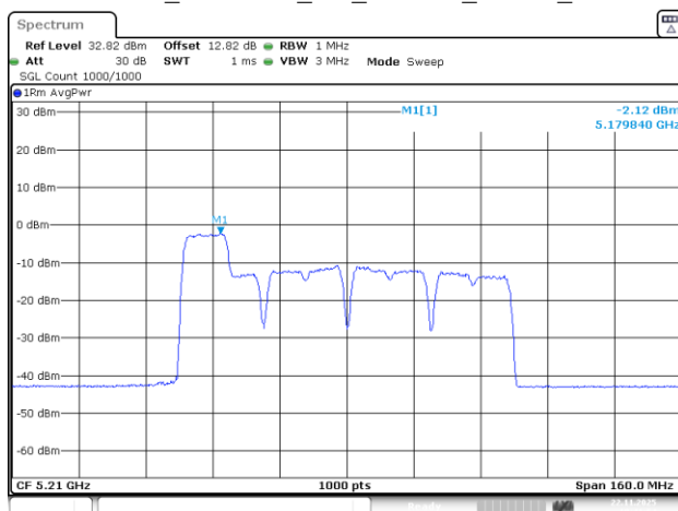
802.11be80_5210MHz_RU_26&106_MRU1_Chain 2
