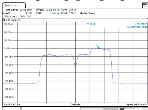
802.11be40_5230MHz_RU_26&106_MRU4_Chain 3
