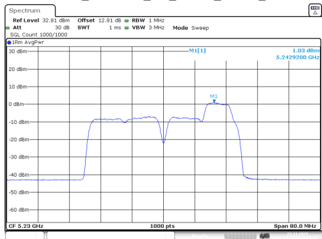
802.11be40_5230MHz_RU_26&52_MRU6_Chain 1
