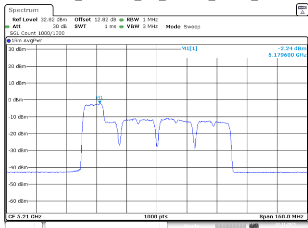
802.11be80_5210MHz_RU_26&106_MRU1_Chain 1
