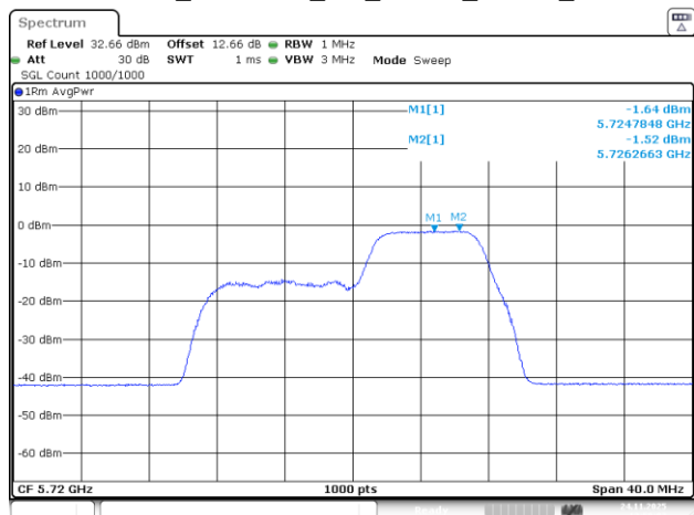
802.11be20_5720MHz_RU_26&52_MRU3_Chain 2
