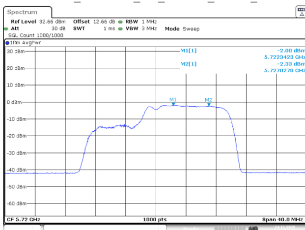
802.11be20_5720MHz_RU_26&106_MRU2_Chain 2
