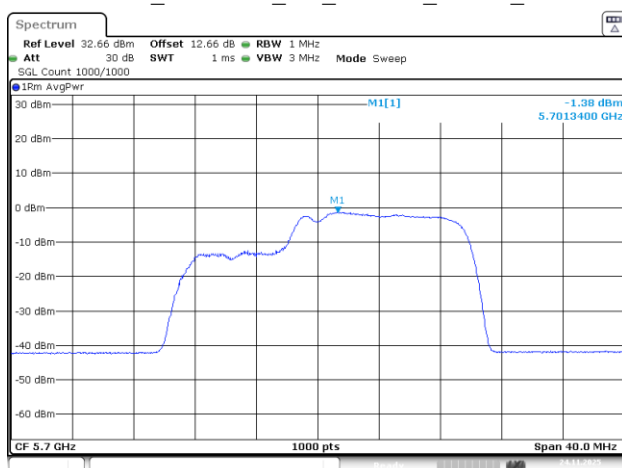
802.11be20_5700MHz_RU_26&106_MRU2_Chain 2
