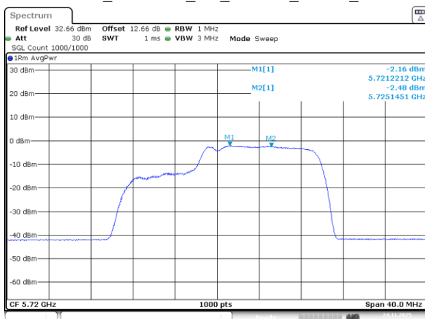
802.11be20_5720MHz_RU_26&106_MRU2_Chain 0
