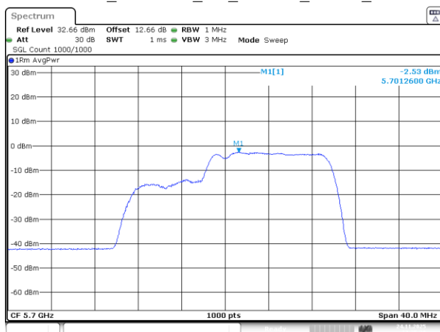
802.11be20_5700MHz_RU_26&106_MRU2_Chain 3
