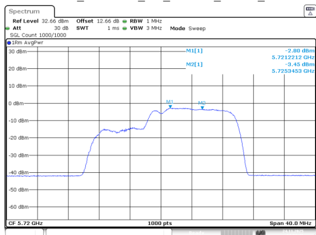
802.11be20_5720MHz_RU_26&106_MRU2_Chain 3
