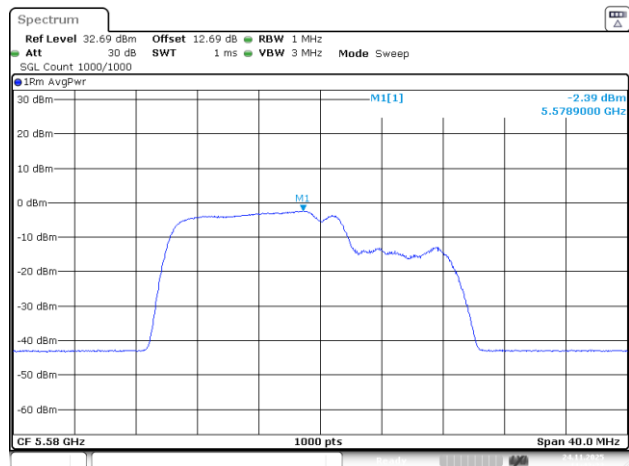
802.11be20_5580MHz_RU_26&106_MRUI_Chain 3
