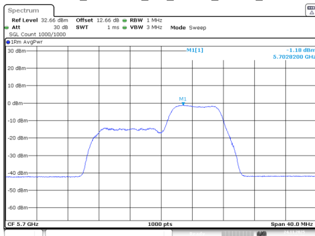
802.11be20_5700MHz_RU_26&52_MRU3_Chain 2
