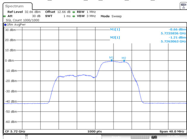
802.11be20_5720MHz_RU_26&52_MRU3_Chain 1
