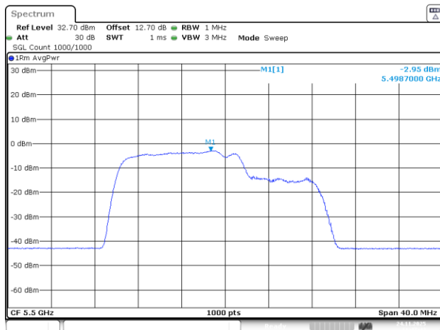
802.11be20_5500MHz_RU_26&106_MRUI_Chain 3
