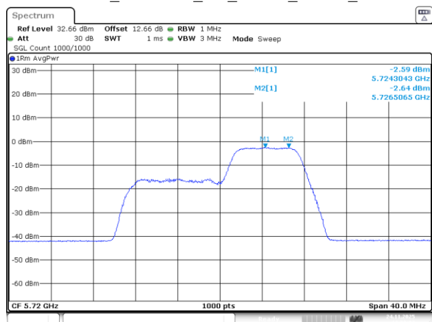
802.11be20_5720MHz_RU_26&52_MRU3_Chain 3
