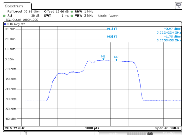
802.11be20_5720MHz_RU_26&106_MRU2_Chain 1
