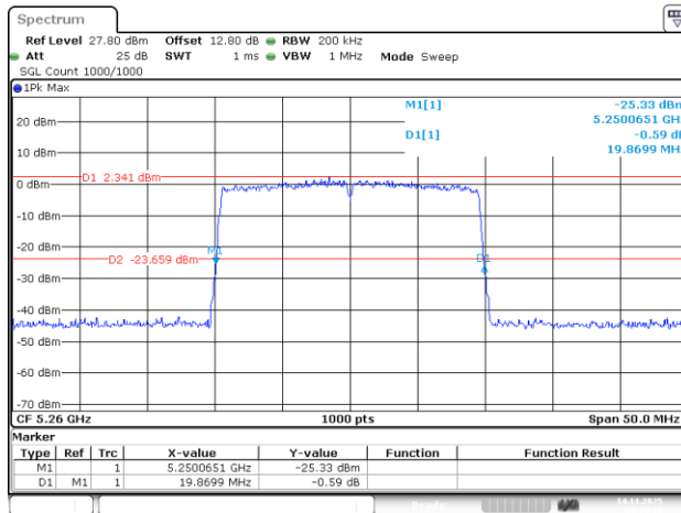
802.11be20_5260MHz_RU_242/61_Chain 0
