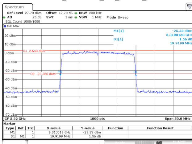
802.11be20_5320MHz_RU_242/61_Chain 2
