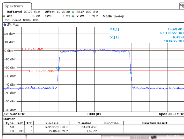
802.11be20_5320MHz_RU_242/61_Chain 0
