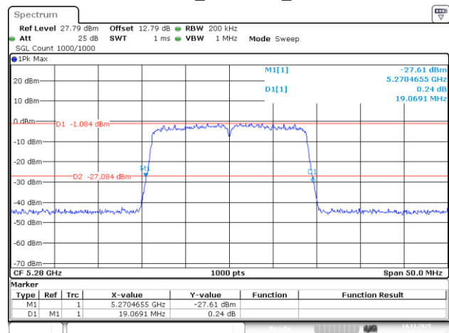
802.11ac20_5280MHz_Chain 2
