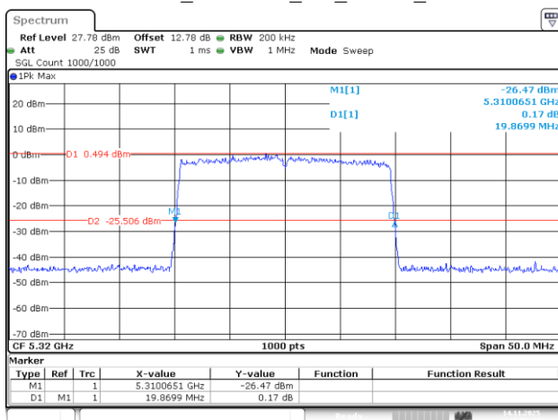
802.11be20_5320MHz_RU_242/61_Chain 3
