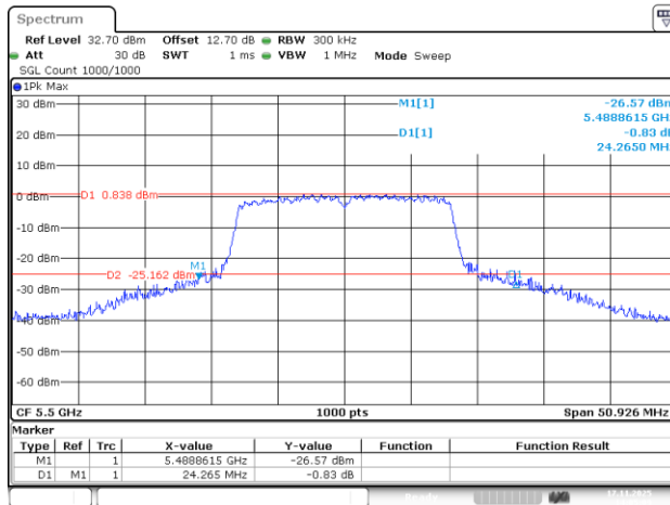
802.11a_5500MHz_Chain 3
