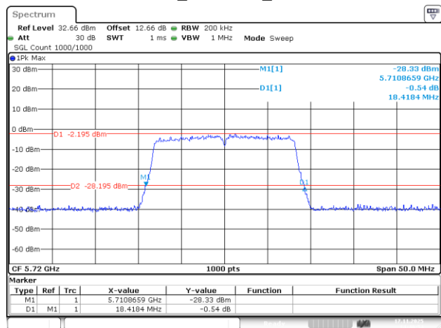
802.11a_5720MHz_Chain 3
