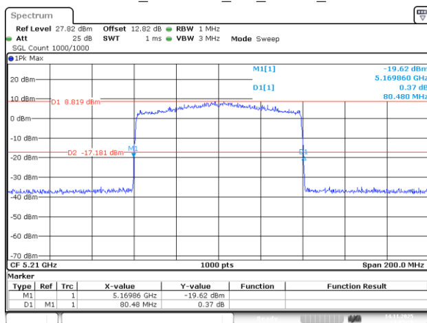
802.11be80_5210MHz_RU_996/67_Chain 2
