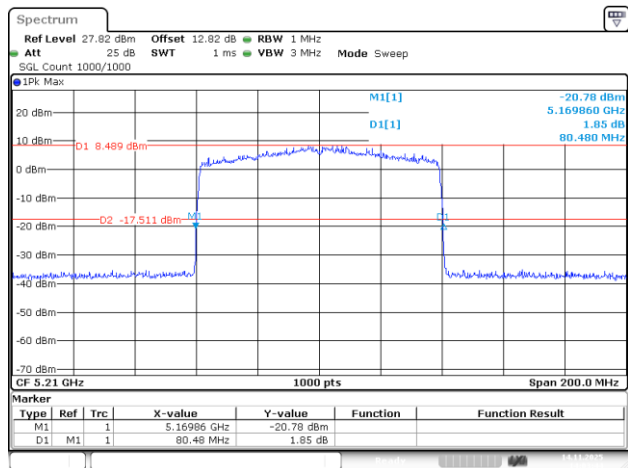
802.11be80_5210MHz_RU_996/67_Chain 1
