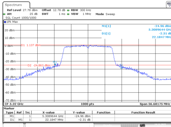
802.11a_5320MHz_Chain 0
