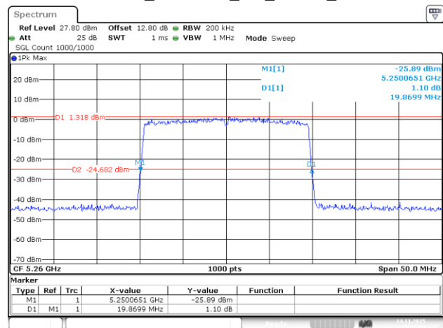
802.11be20_5260MHz_RU_242/61_Chain 1
