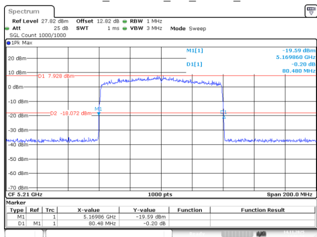
802.11be80_5210MHz_RU_996/67_Chain 3
