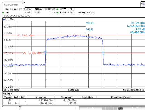
802.11be80_5210MHz_RU_996/67_Chain 0
