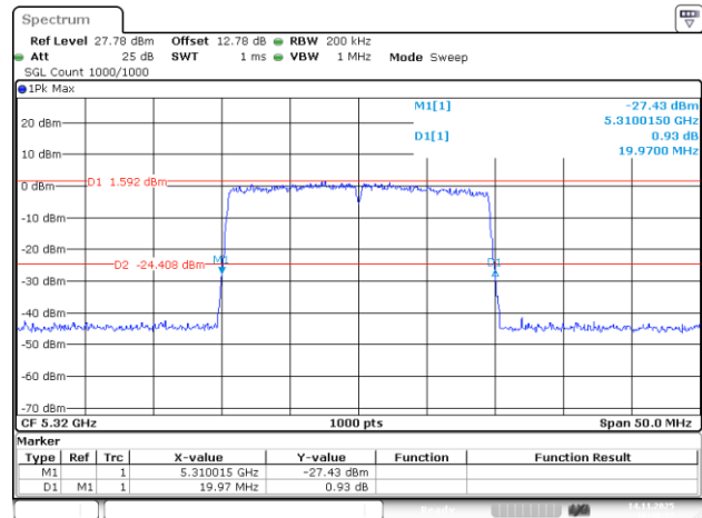
802.11be20_5320MHz_RU_242/61_Chain 1
