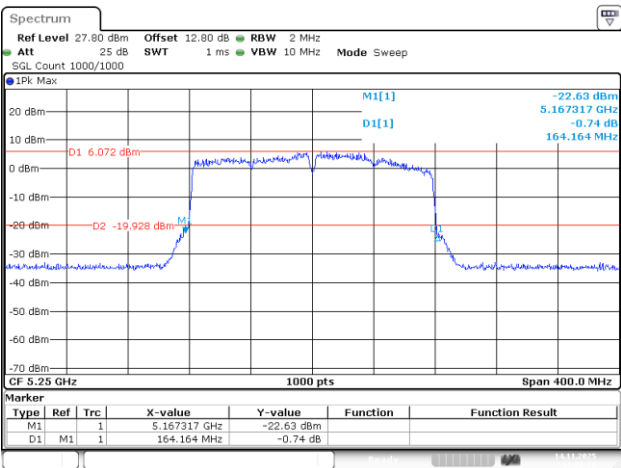
802.11ac160_5250MHz_Chain 3
