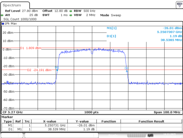
802.11ac40_5270MHz_Chain 2
