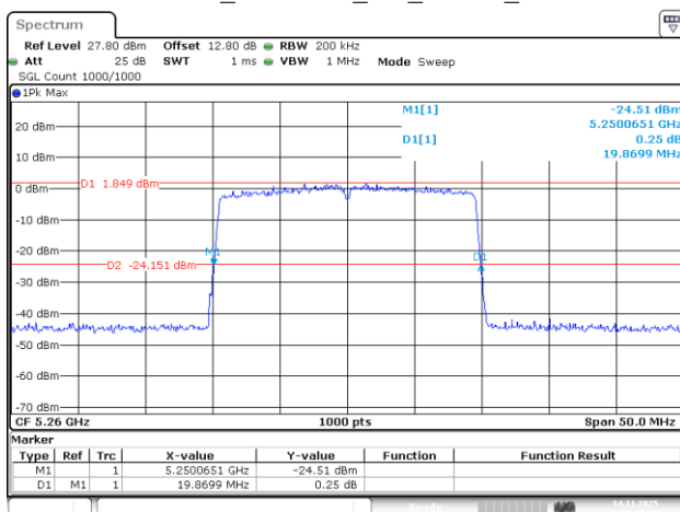
802.11be20_5260MHz_RU_242/61_Chain 3
