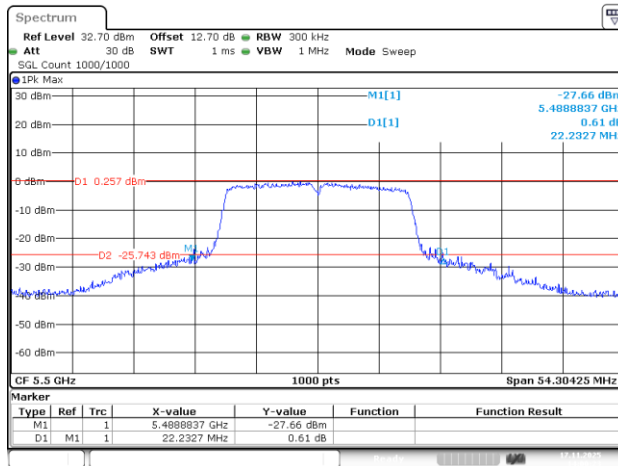
802.11a_5500MHz_Chain 1
