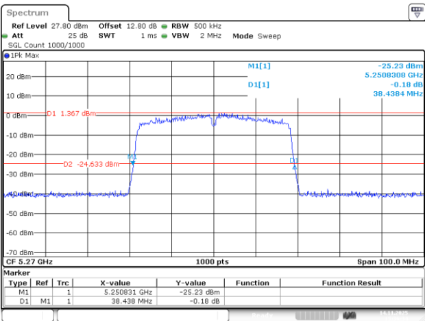
802.11ac40_5270MHz_Chain 3
