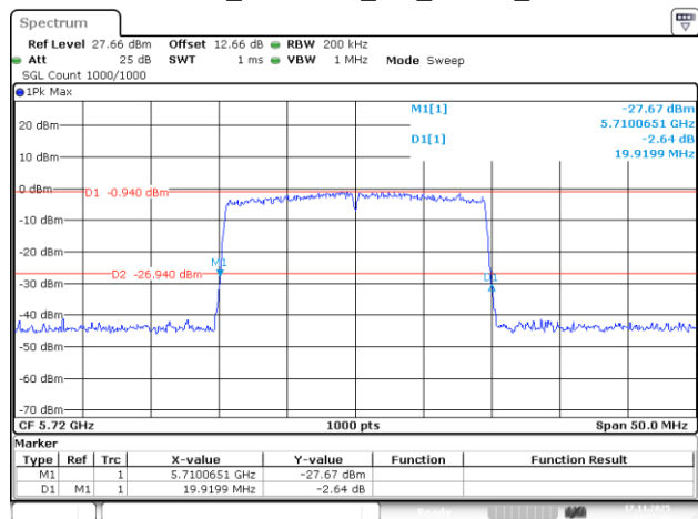
802.11be20_5720MHz_RU_242/61_Chain 3
