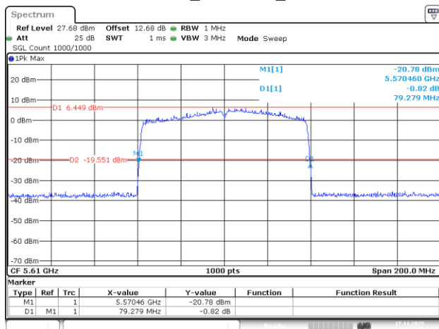
802.11ac80_5610MHz_Chain 3
