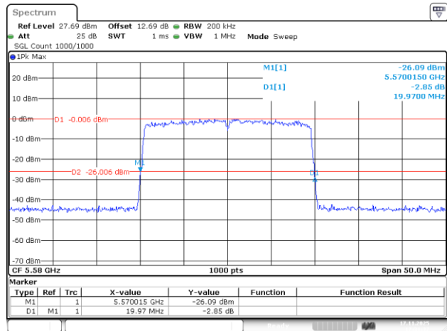
802.11be20_5580MHz_RU_242/61_Chain 3
