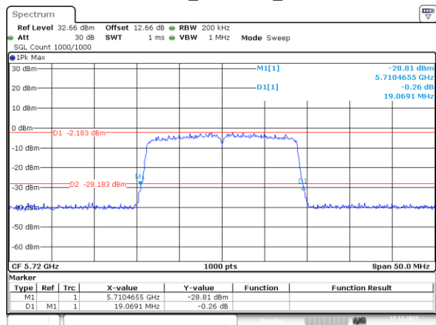
802.11ac20_5720MHz_Chain 3
