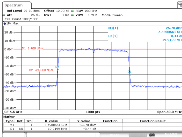
802.11be20_5500MHz_RU_242/61_Chain 0
