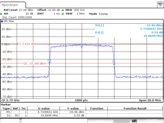
802.11be20_5720MHz_RU_242/61_Chain 1
