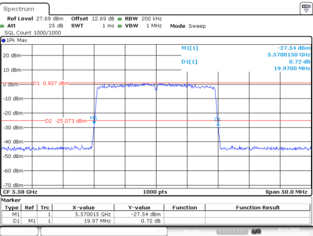
802.11be20_5580MHz_RU_242/61_Chain 1
