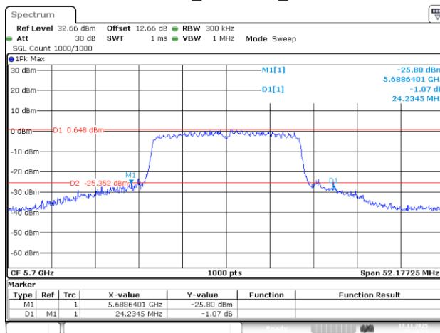
802.11ac20_5700MHz_Chain 2
