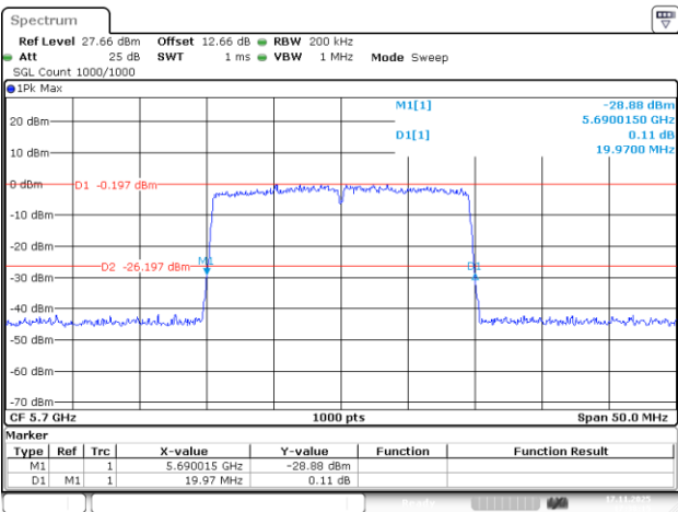
802.11be20_5700MHz_RU_242/61_Chain 1
