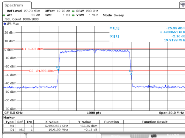
802.11be20_5500MHz_RU_242/61_Chain 3
