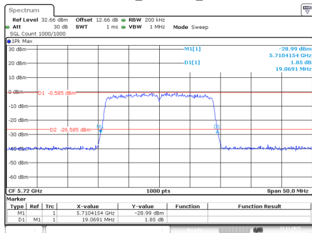
802.11ac20_5720MHz_Chain 0
