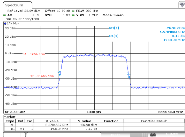
802.11ac20_5580MHz_Chain 0
