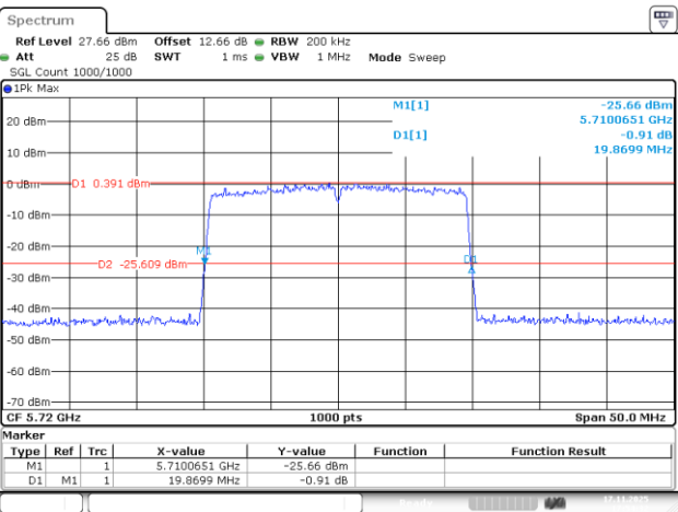
802.11be20_5720MHz_RU_242/61_Chain 2
