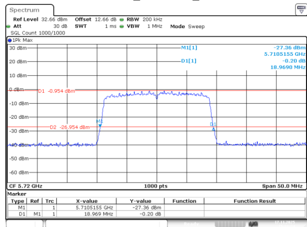
802.11ac20_5720MHz_Chain 2
