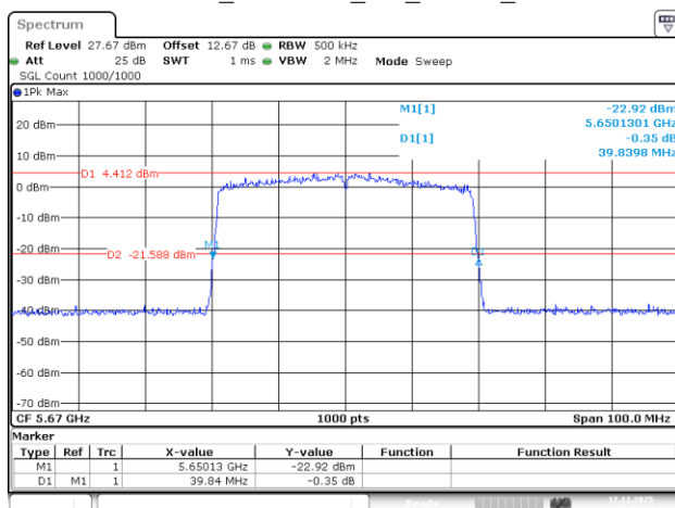
802.11be40_5670MHz_RU_484/65_Chain 1
