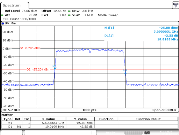
802.11be20_5700MHz_RU_242/61_Chain 2
