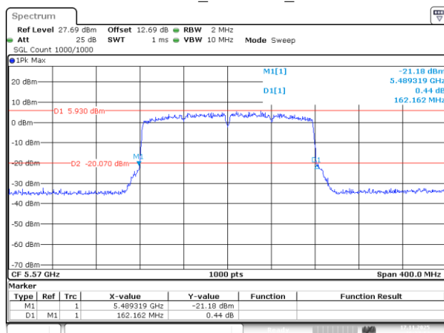
802.11ac160_5570MHz_Chain 3
