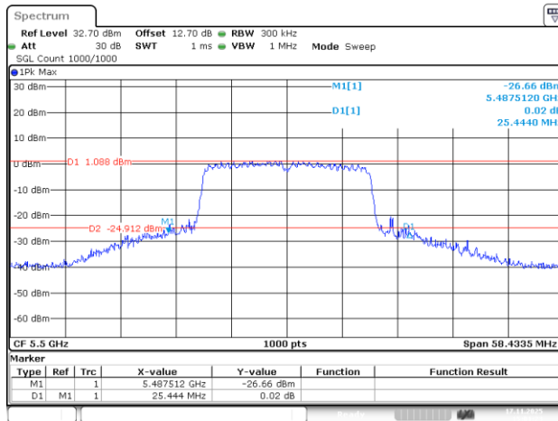
802.11ac20_5500MHz_Chain 2
