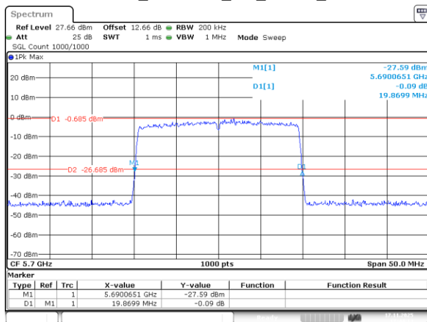
802.11be20_5700MHz_RU_242/61_Chain 3
