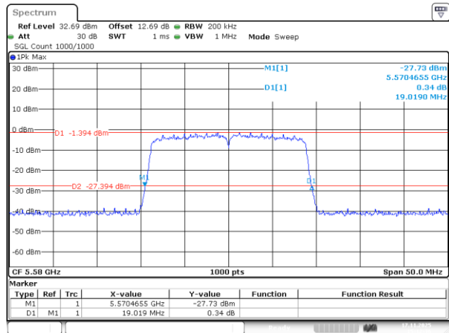
802.11ac20_5580MHz_Chain 3
