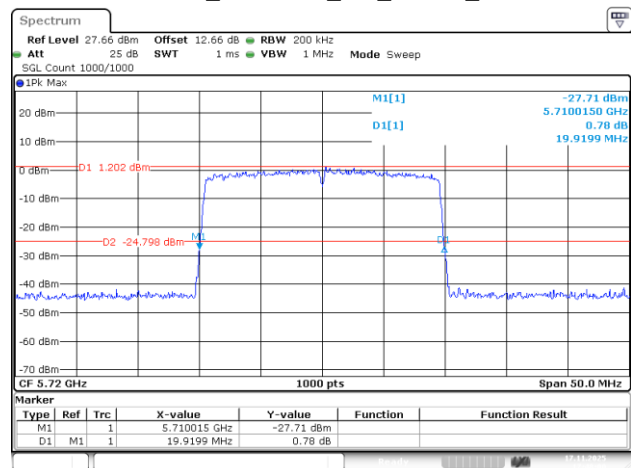
802.11be20_5720MHz_RU_242/61_Chain 0
