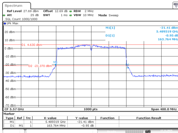
802.11ac160_5570MHz_Chain 1
