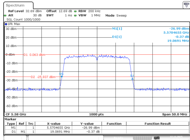
802.11ac20_5580MHz_Chain 2
