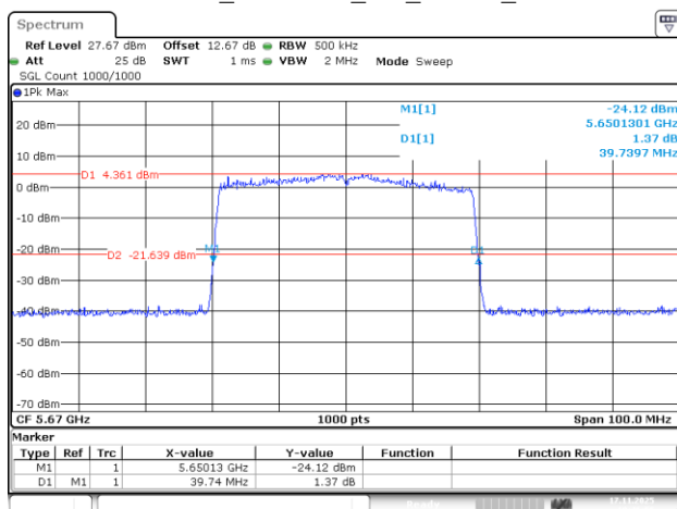
802.11be40_5670MHz_RU_484/65_Chain 2
