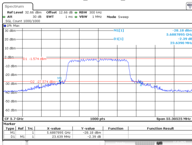
802.11ac20_5700MHz_Chain 3
