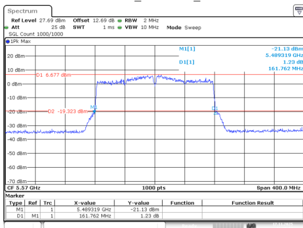
802.11ac160_5570MHz_Chain 2
