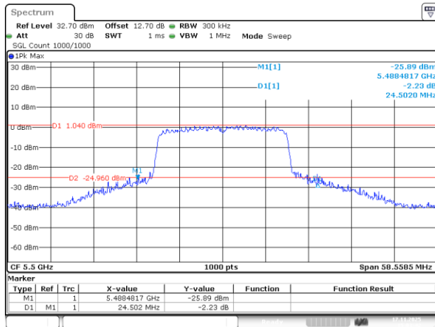
802.11ac20_5500MHz_Chain 3
