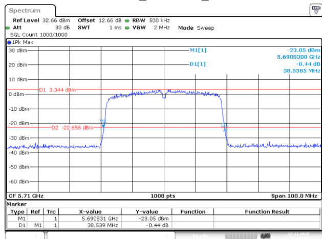
802.11ac40_5710MHz_Chain 2
