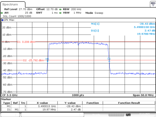
802.11be20_5500MHz_RU_242/61_Chain 1
