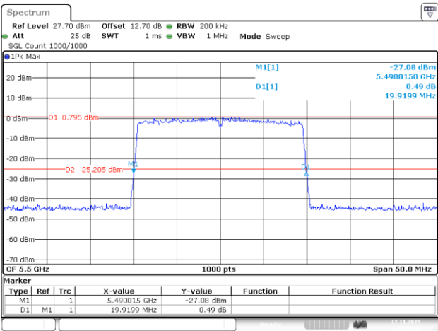
802.11be20_5500MHz_RU_242/61_Chain 2
