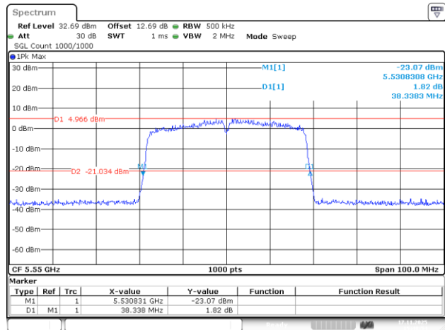
802.11ac40_5550MHz_Chain 2
