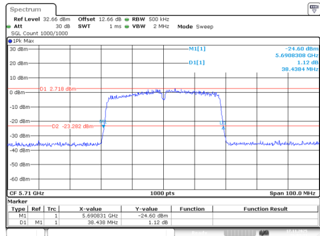
802.11ac40_5710MHz_Chain 3
