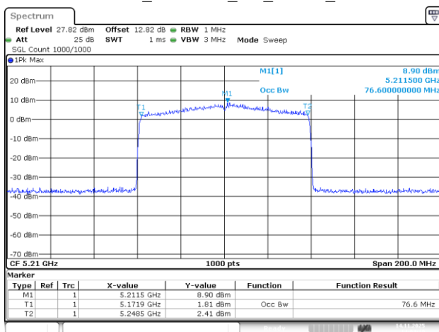
802.11be80_5210MHz_RU_996/67_Chain 1
