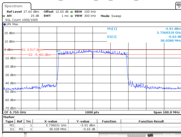
802.11be40_5755MHz_RU_484/65_Chain 1
