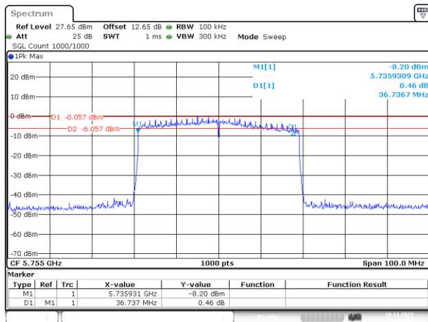
802.11be40_5755MHz_RU_484/65_Chain 2
