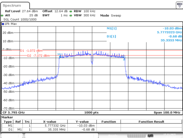
802.11ac40_5795MHz_Chain 3
