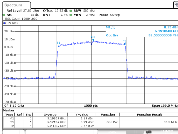
802.11be40_5190MHz_RU_484/65_Chain 2
