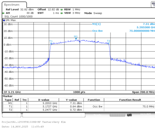
802.11ac80_5210MHz_Chain 2
