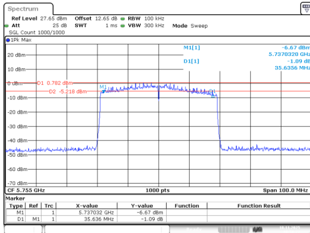
802.11be40_5755MHz_RU_484/65_Chain 0
