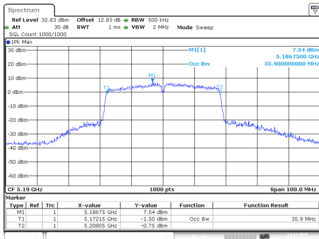
802.11ac40_5190MHz_Chain 2
