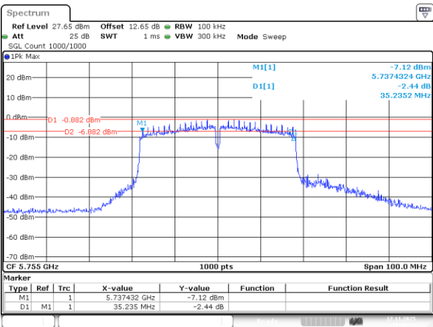
802.11ac40_5755MHz_Chain 3
