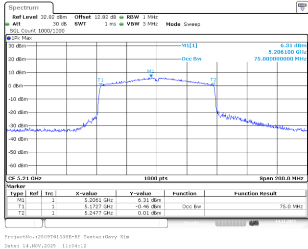
802.11ac80_5210MHz_Chain 3
