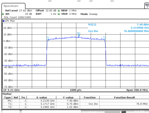
802.11be80_5210MHz_RU_996/67_Chain 3
