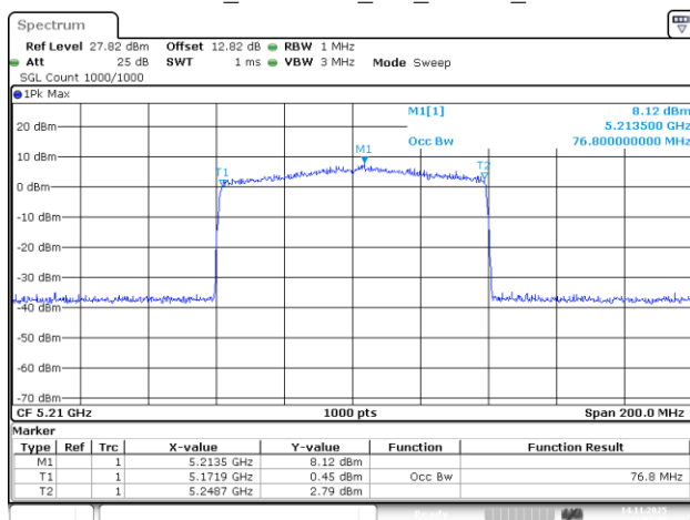
802.11be80_5210MHz_RU_996/67_Chain 0
