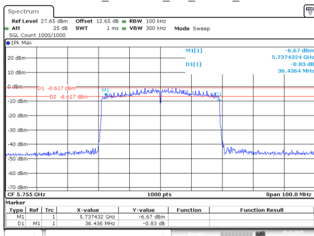
802.11be40_5755MHz_RU_484/65_Chain 3
