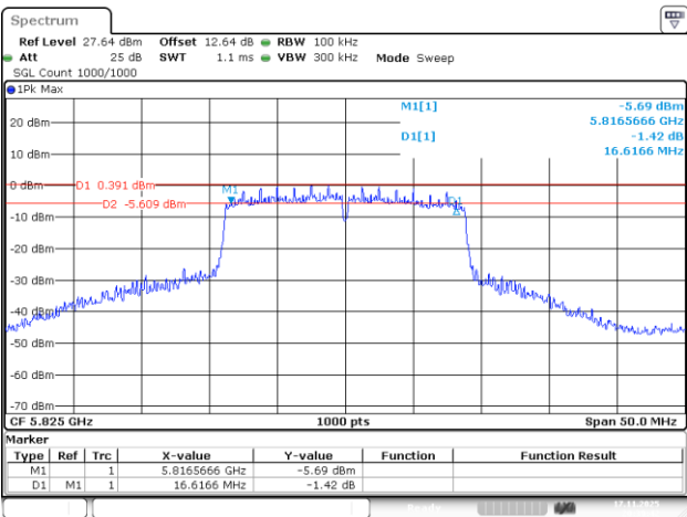
802.11ac20_5825MHz_Chain 3
