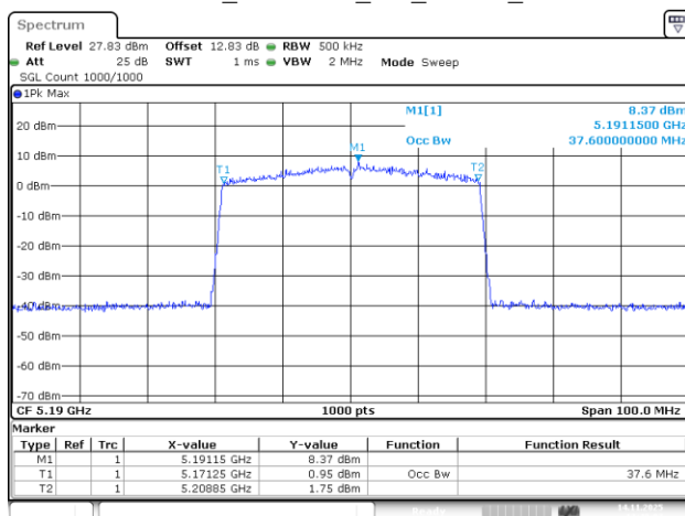
802.11be40_5190MHz_RU_484/65_Chain 1
