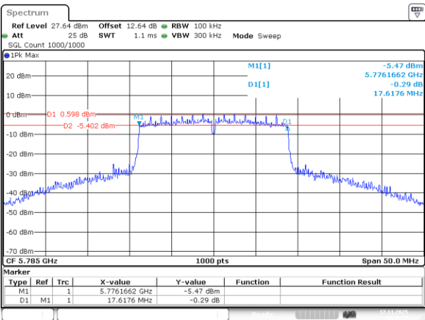
802.11ac20_5785MHz_Chain 3
