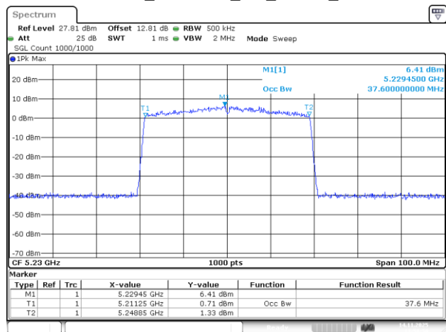
802.11be40_5230MHz_RU_484/65_Chain 3
