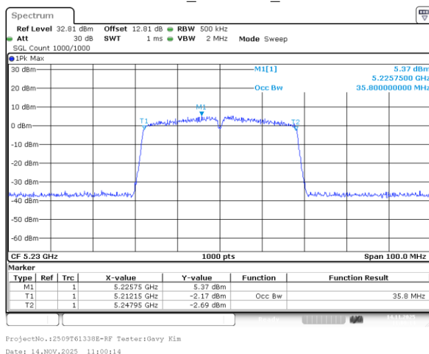
802.11ac40_5230MHz_Chain 3
