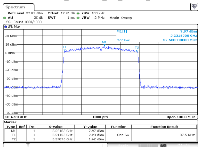
802.11be40_5230MHz_RU_484/65_Chain 1
