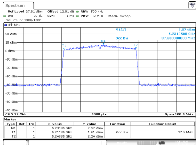
802.11be40_5230MHz_RU_484/65_Chain 0
