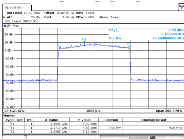
802.11be80_5210MHz_RU_996/67_Chain 2
