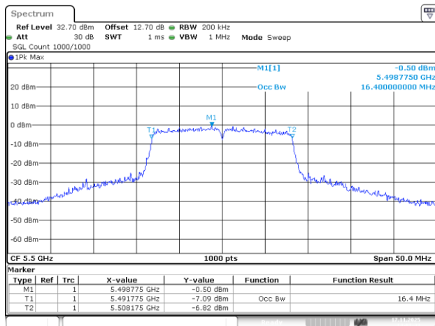
802.11a_5500MHz_Chain 2
