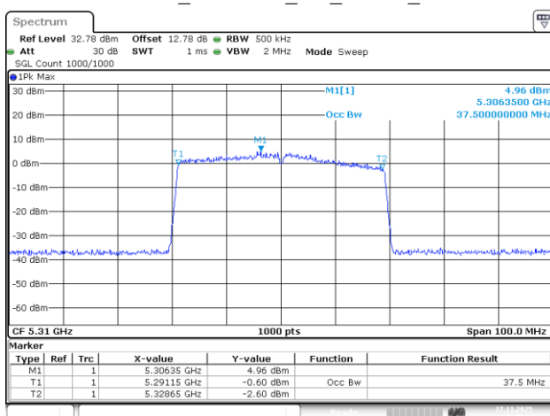
802.11be40_5310MHz_RU_484/65_Chain 3
