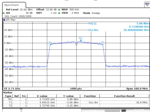
802.11ac40_5710MHz_Chain 0
