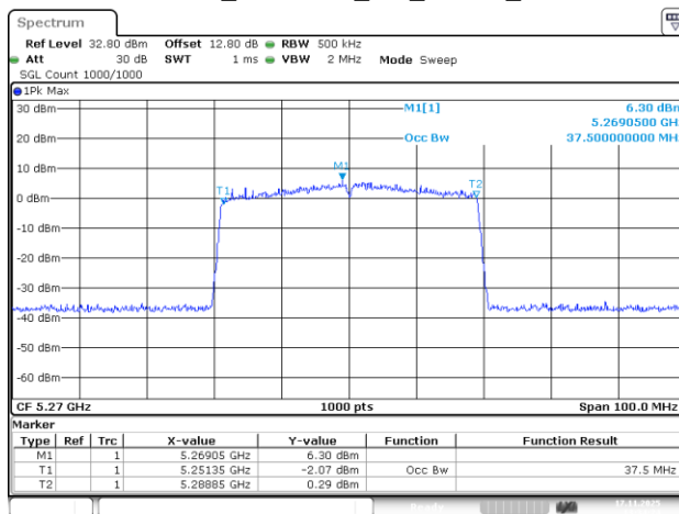
802.11be40_5270MHz_RU_484/65_Chain 1
