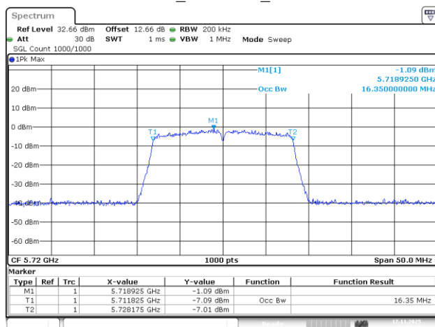
802.11a_5720MHz_Chain 2
