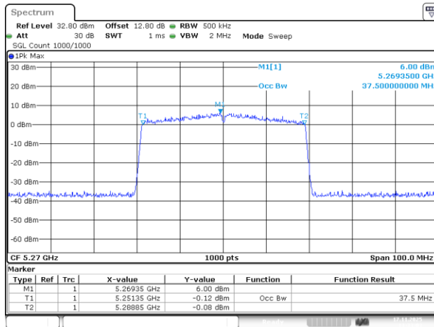
802.11be40_5270MHz_RU_484/65_Chain 0
