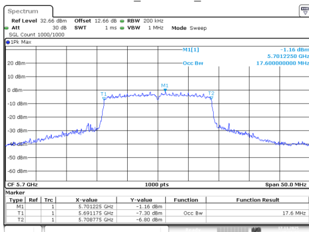
802.11ac20_5700MHz_Chain 2
