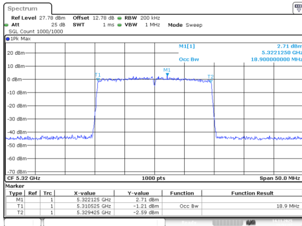
802.11be20_5320MHz_RU_242/61_Chain 2
