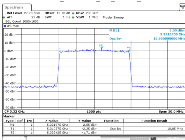
802.11be20_5320MHz_RU_242/61_Chain 0
