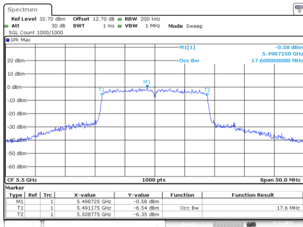
802.11ac20_5500MHz_Chain 2
