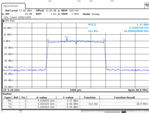
802.11be20_5260MHz_RU_242/61_Chain 1
