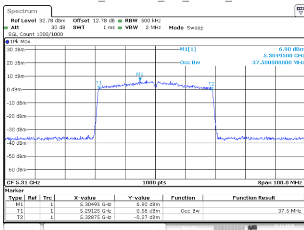
802.11be40_5310MHz_RU_484/65_Chain 2
