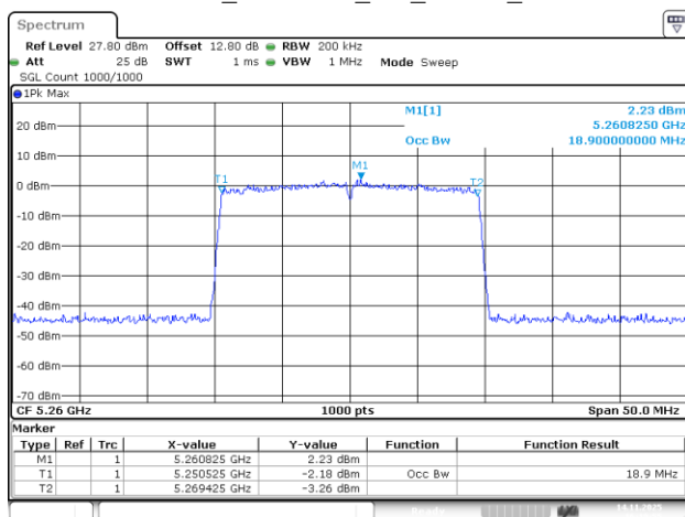
802.11be20_5260MHz_RU_242/61_Chain 0
