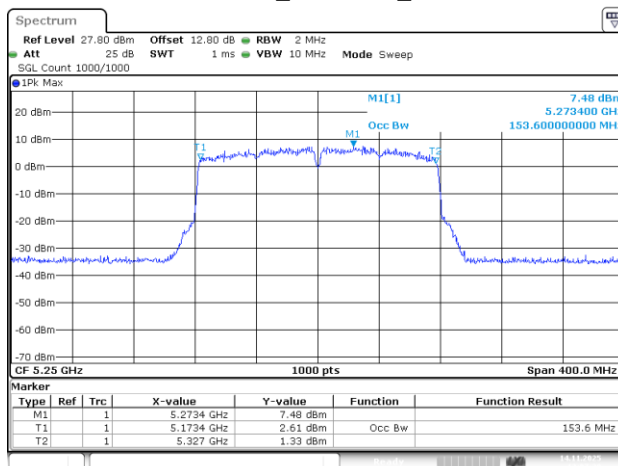
802.11ac160_5250MHz_Chain 2
