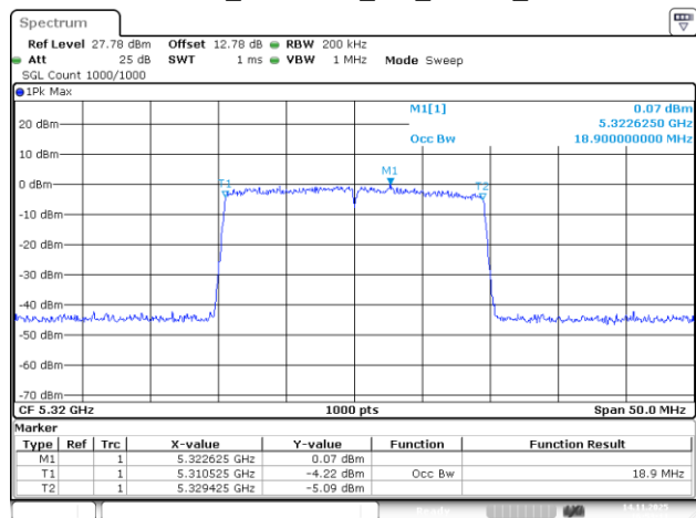
802.11be20_5320MHz_RU_242/61_Chain 3
