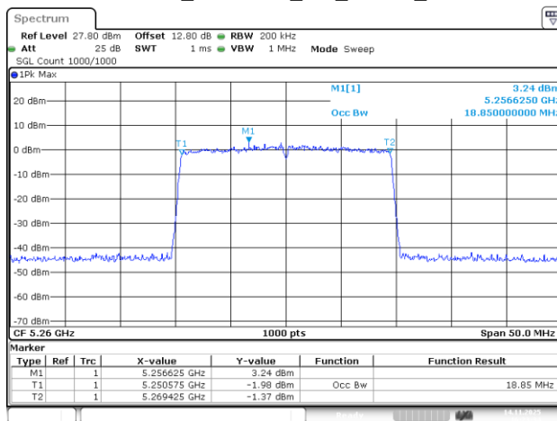
802.11be20_5260MHz_RU_242/61_Chain 2
