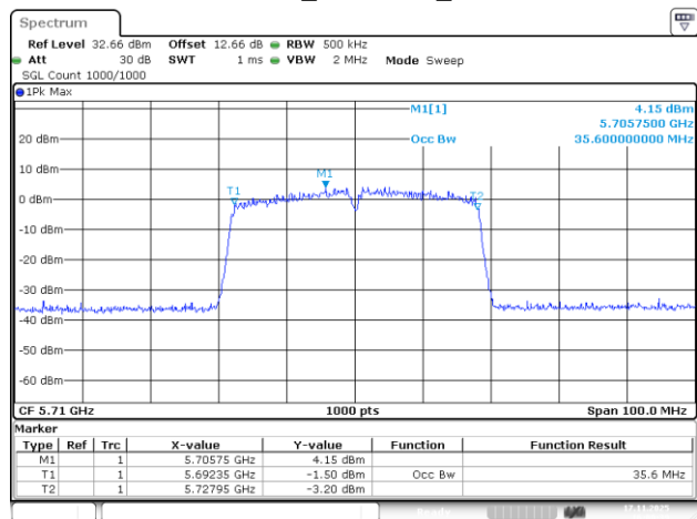
802.11ac40_5710MHz_Chain 1
