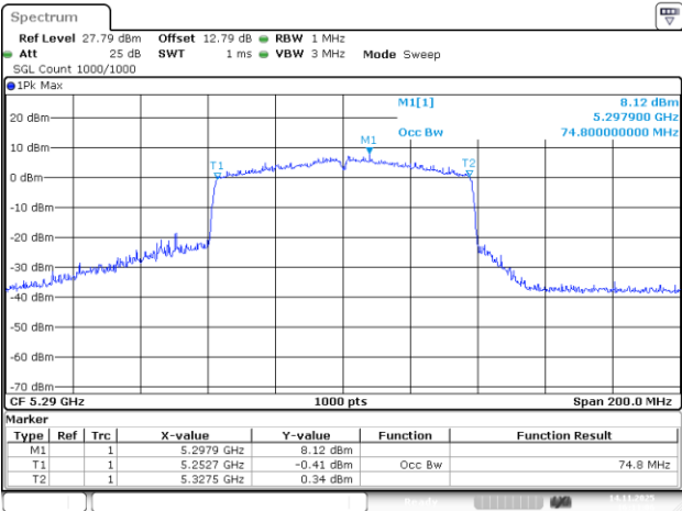
802.11ac80_5290MHz_Chain 2
