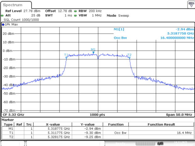
802.11a_5320MHz_Chain 3
