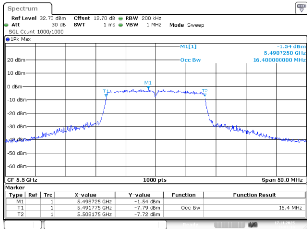
802.11a_5500MHz_Chain 1
