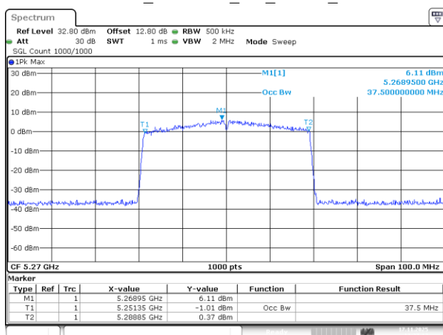
802.11be40_5270MHz_RU_484/65_Chain 3
