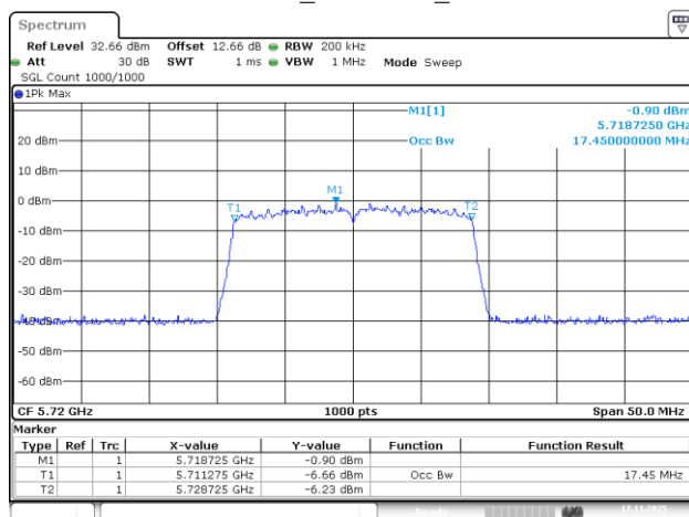
802.11ac20_5720MHz_Chain 2
