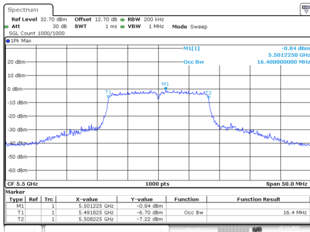
802.11a_5500MHz_Chain 3
