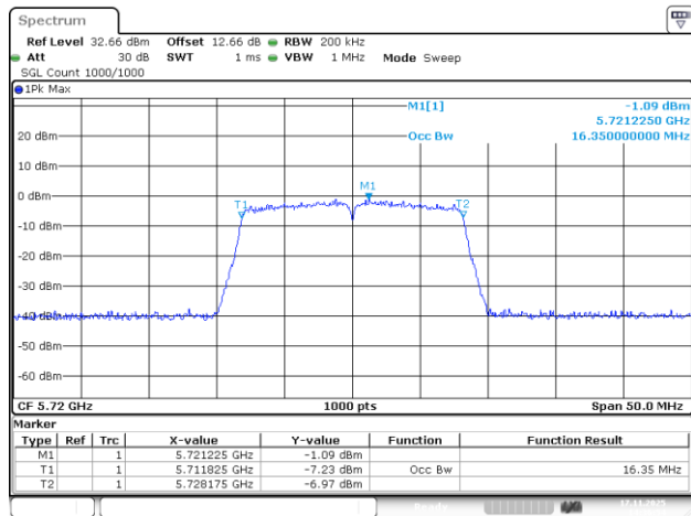
802.11a_5720MHz_Chain 1
