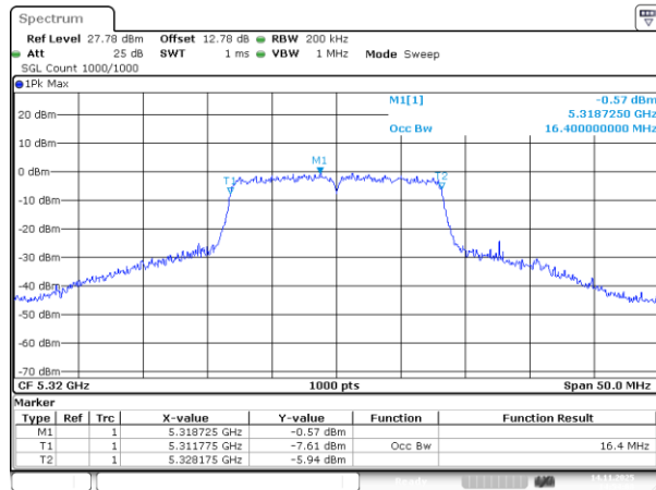
802.11a_5320MHz_Chain 0
