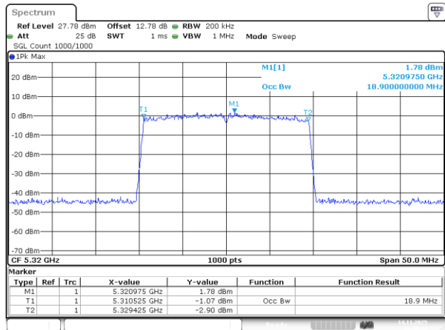
802.11be20_5320MHz_RU_242/61_Chain 1
