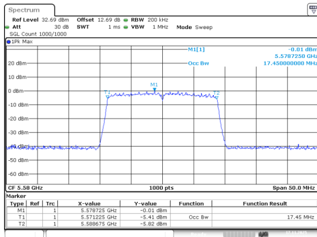
802.11ac20_5580MHz_Chain 2
