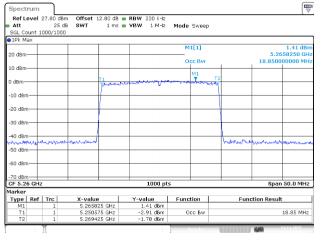
802.11be20_5260MHz_RU_242/61_Chain 3
