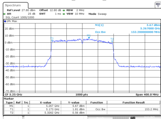
802.11ac160_5250MHz_Chain 3
