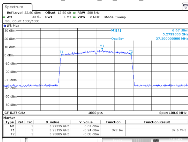
802.11be40_5270MHz_RU_484/65_Chain 2
