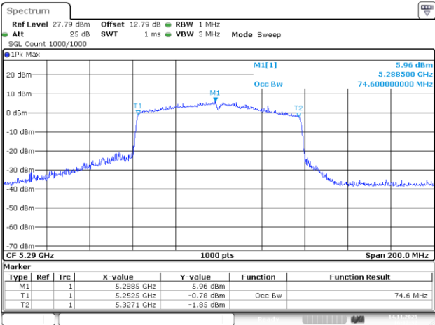
802.11ac80_5290MHz_Chain 3
