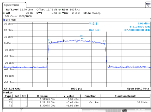
802.11be40_5310MHz_RU_484/65_Chain 1
