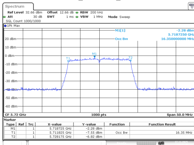
802.11a_5720MHz_Chain 3
