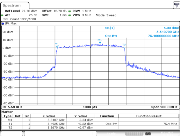
802.11ac80_5530MHz_Chain 2
