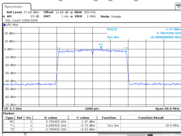
802.11be20_5700MHz_RU_242/61_Chain 2
