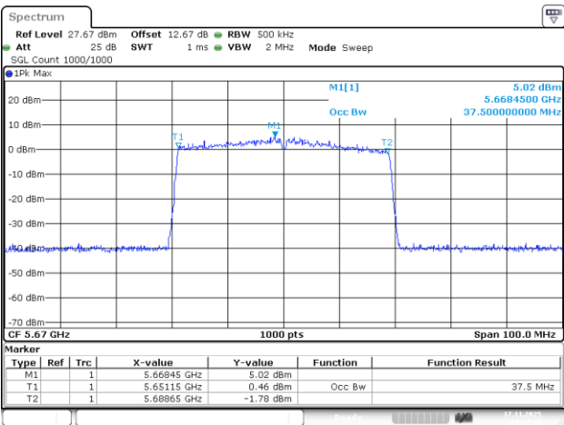
802.11be40_5670MHz_RU_484/65_Chain 2
