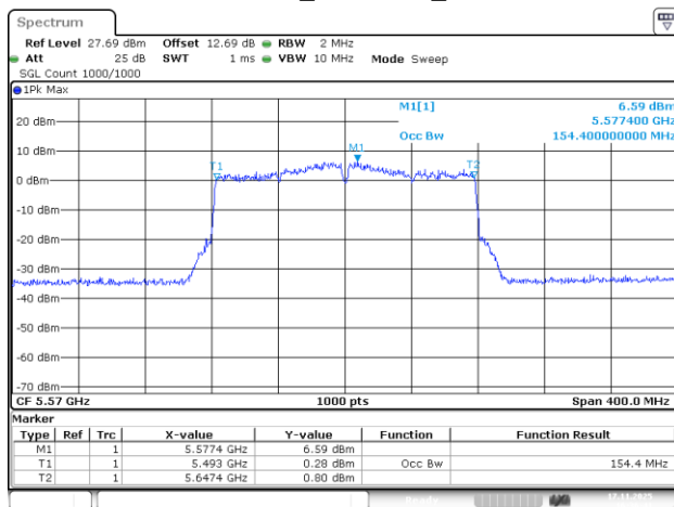
802.11ac160_5570MHz_Chain 2
