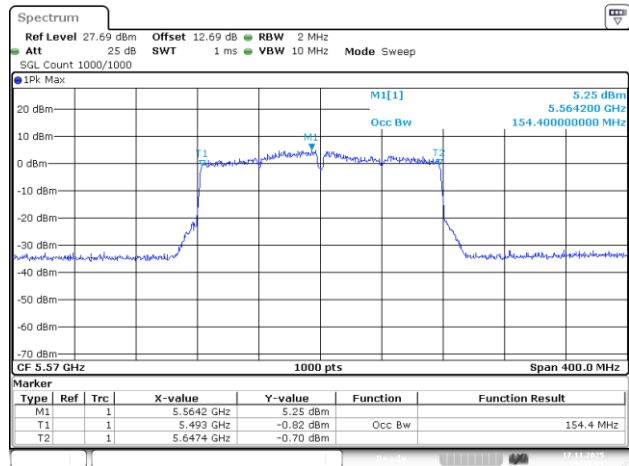
802.11ac160_5570MHz_Chain 1
