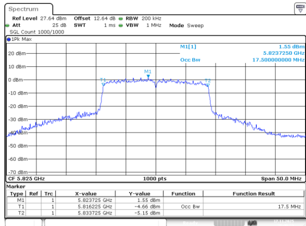
802.11ac20_5825MHz_Chain 3
