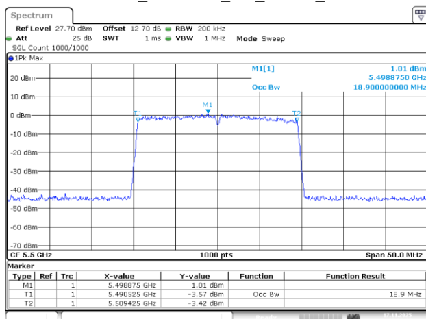
802.11be20_5500MHz_RU_242/61_Chain 2
