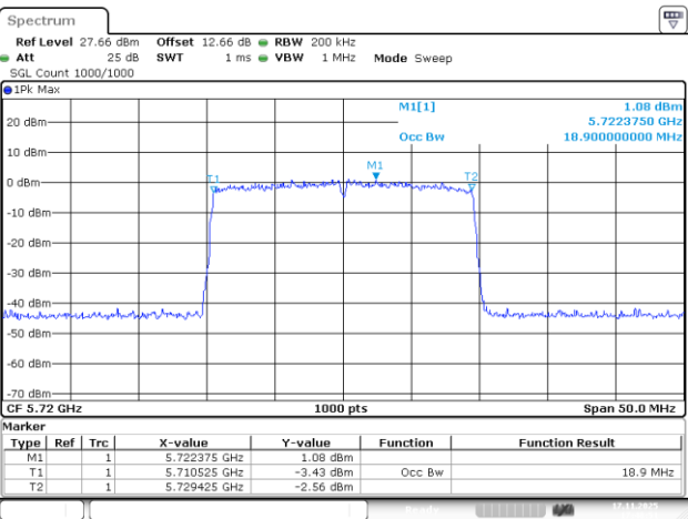
802.11be20_5720MHz_RU_242/61_Chain 0
