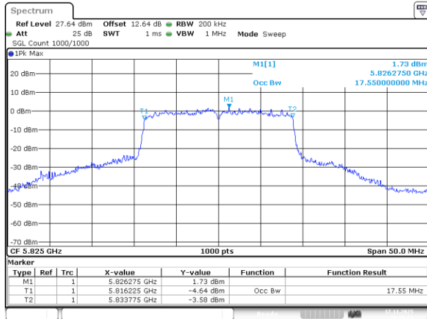
802.11ac20_5825MHz_Chain 2
