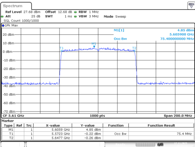
802.11ac80_5610MHz_Chain 2
