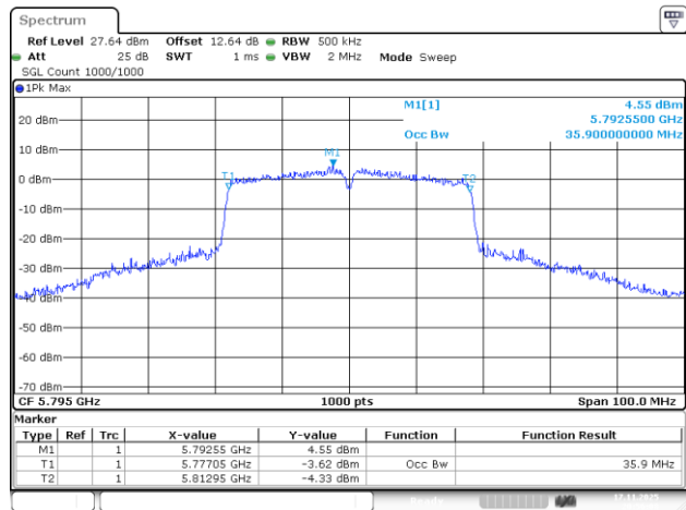
802.11ac40_5795MHz_Chain 3
