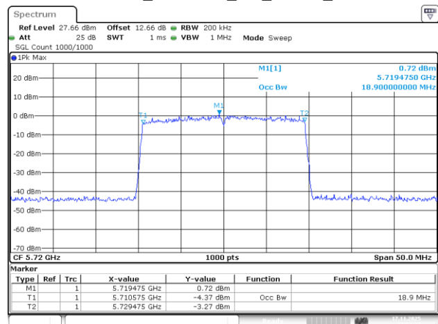
802.11be20_5720MHz_RU_242/61_Chain 1
