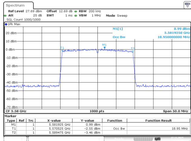
802.11be20_5580MHz_RU_242/61_Chain 1
