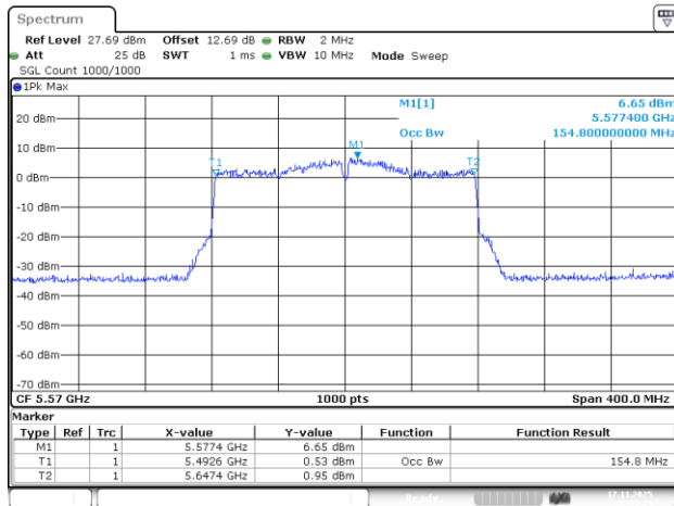
802.11ac160_5570MHz_Chain 0
