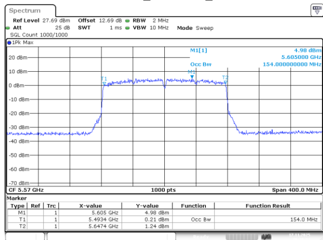
802.11ac160_5570MHz_Chain 3
