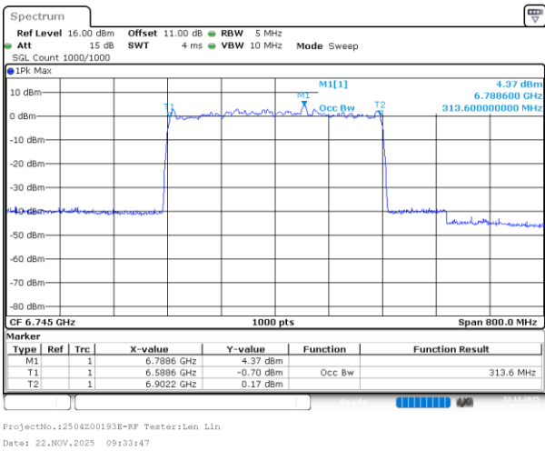
802.11be320_6745MHz_RU_4*996_Chain 3
