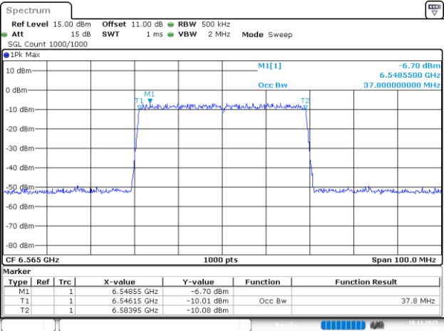
802.11be40_6565MHz_RU_484/65_Chain 3
