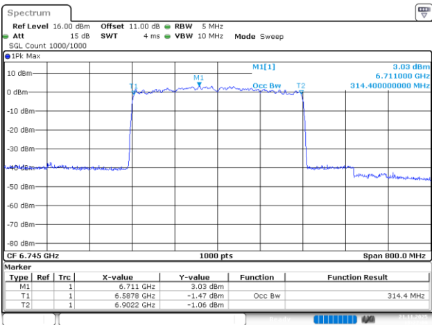
802.11be320_6745MHz_RU_4*996_Chain 2
