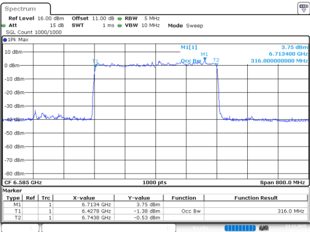
802.11be320_6585MHz_RU_4*996_Chain 0
