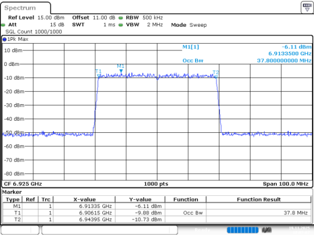
802.11be40_6925MHz_RU_484/65_Chain 3
