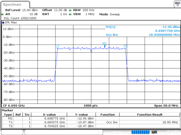
802.11be20_6695MHz_RU_242/61_Chain 2
