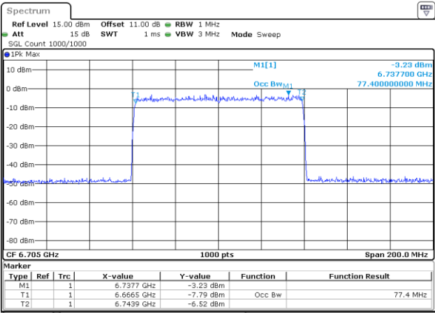
802.11be80_6705MHz_RU_996/67_Chain 1
