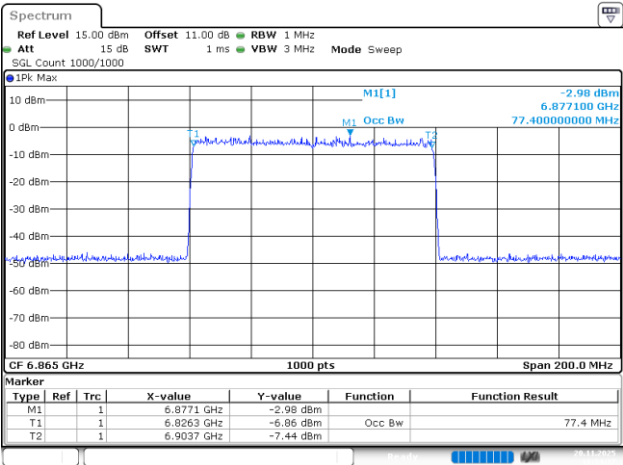
802.11be80_6865MHz_RU_996/67_Chain 1
