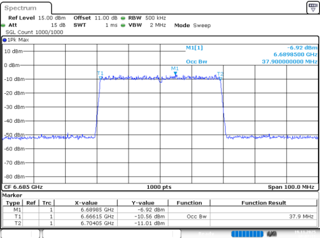
802.11be40_6685MHz_RU_484/65_Chain 0
