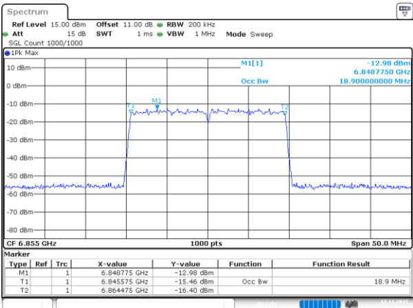
802.11be20_6855MHz_RU_242/61_Chain 0
