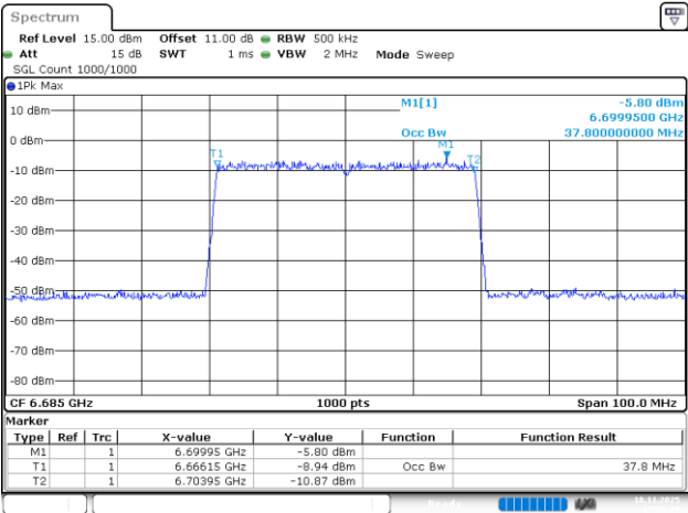
802.11be40_6685MHz_RU_484/65_Chain 3
