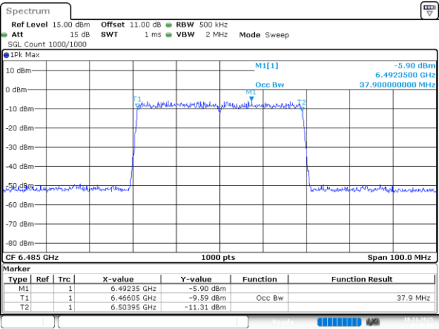
802.11be40_6485MHz_RU_484/65_Chain 3
