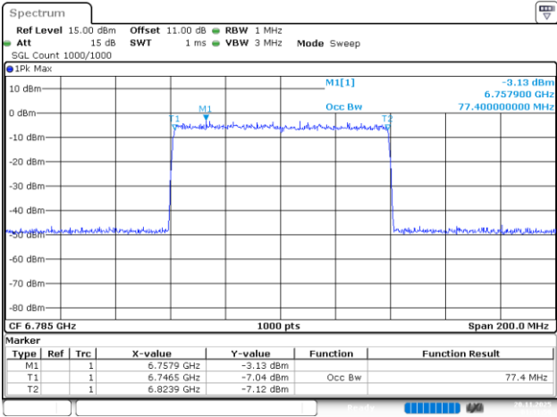
802.11be80_6785MHz_RU_996/67_Chain 3
