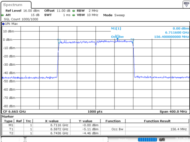
802.11be160_6665MHz_RU_2*996_Chain 3
