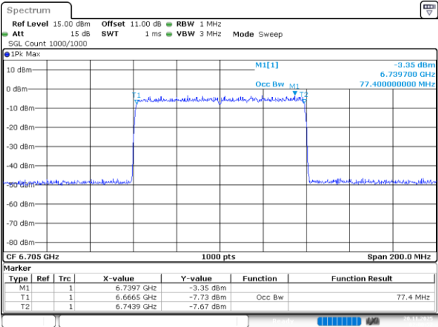
802.11be80_6705MHz_RU_996/67_Chain 0
