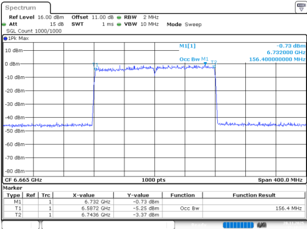
802.11be160_6665MHz_RU_2*996_Chain 1
