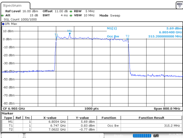
802.11be320_6905MHz_RU_4*996_Chain 1
