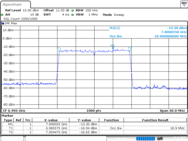
802.11be20_6995MHz_RU_242/61_Chain 1
