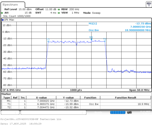
802.11be20_6995MHz_RU_242/61_Chain 0
