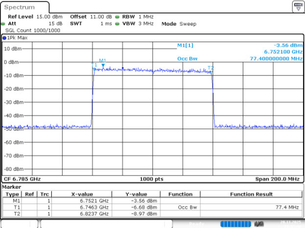
802.11be80_6785MHz_RU_996/67_Chain 0
