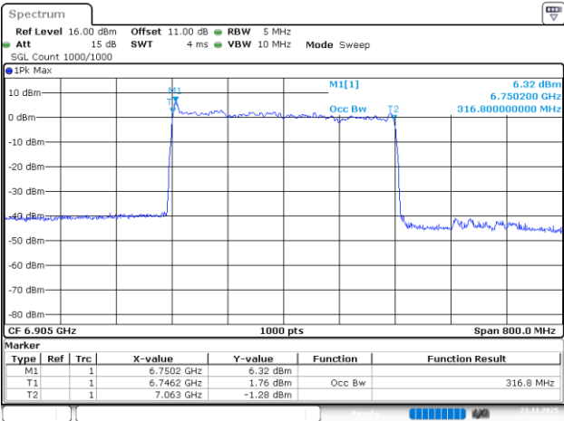
802.11be320_6905MHz_RU_4*996_Chain 2
