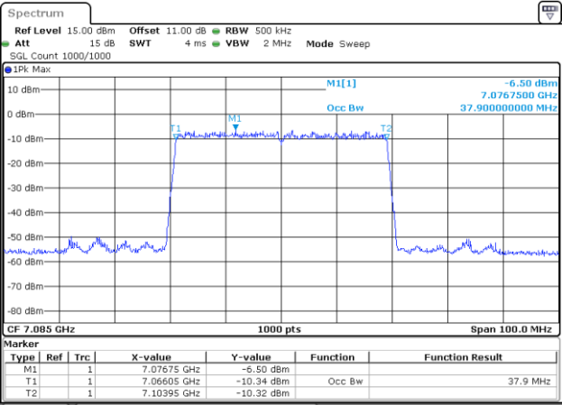
802.11be40_7085MHz_RU_484/65_Chain 0
