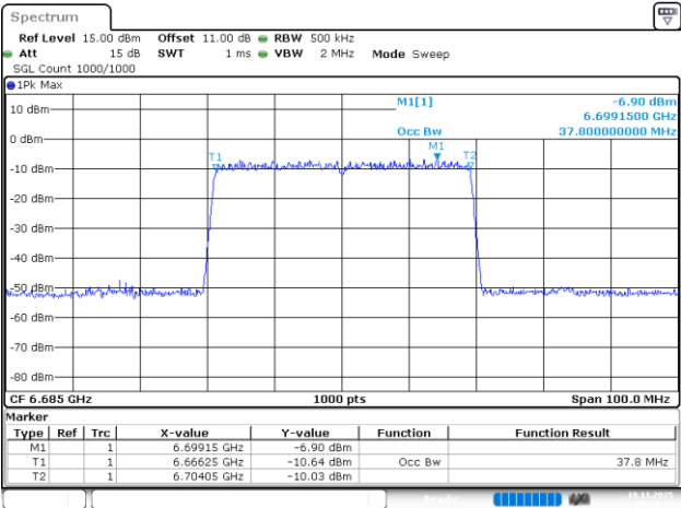
802.11be40_6685MHz_RU_484/65_Chain 1
