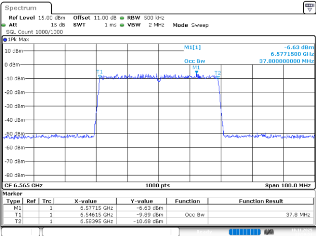
802.11be40_6565MHz_RU_484/65_Chain 0
