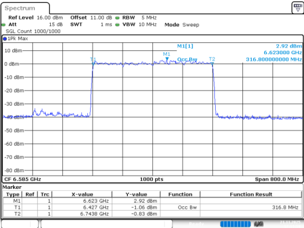
802.11be320_6585MHz_RU_4*996_Chain 1
