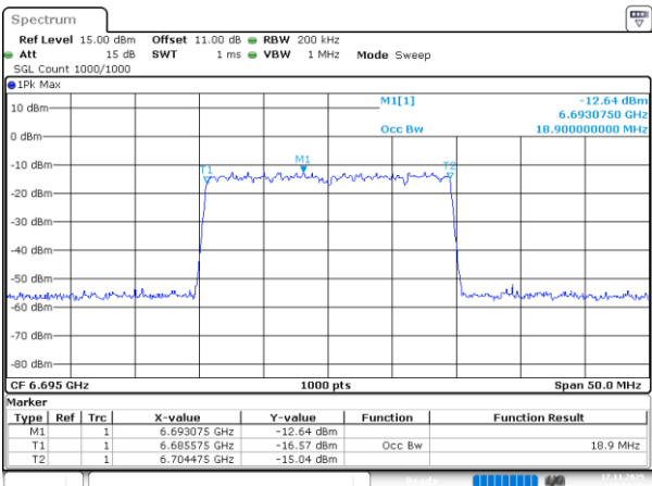
802.11be20_6695MHz_RU_242/61_Chain 1
