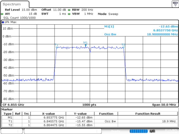
802.11be20_6855MHz_RU_242/61_Chain 2
