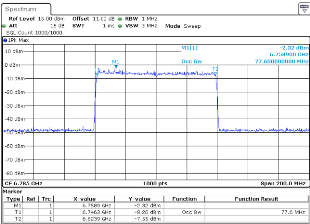
802.11be80_6785MHz_RU_996/67_Chain 2
