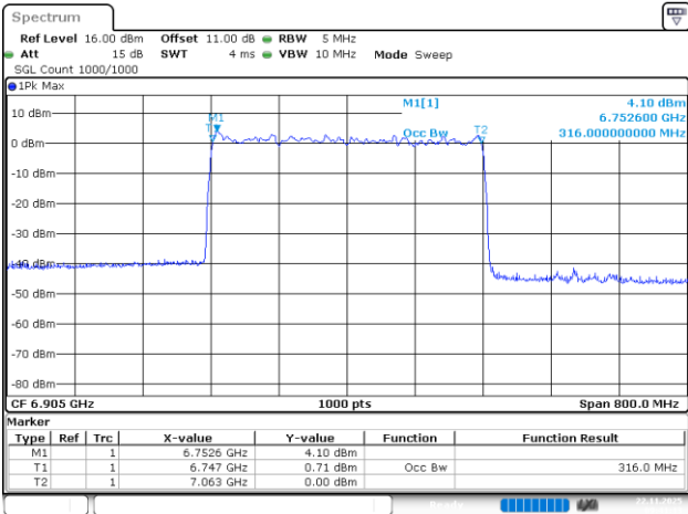
802.11be320_6905MHz_RU_4*996_Chain 3
