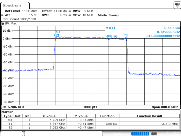
802.11be320_6905MHz_RU_4*996_Chain 0
