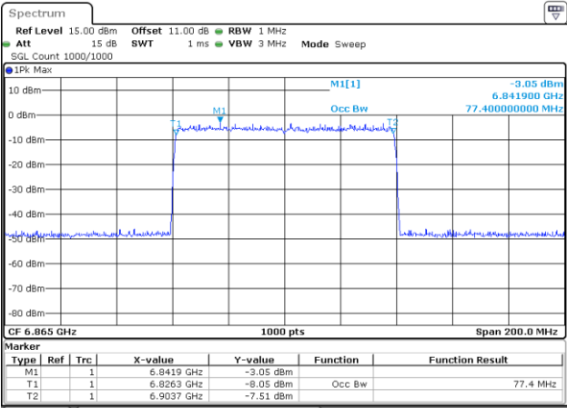
802.11be80_6865MHz_RU_996/67_Chain 2
