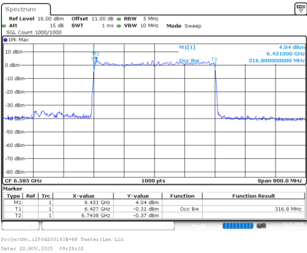
802.11be320_6585MHz_RU_4*996_Chain 3
