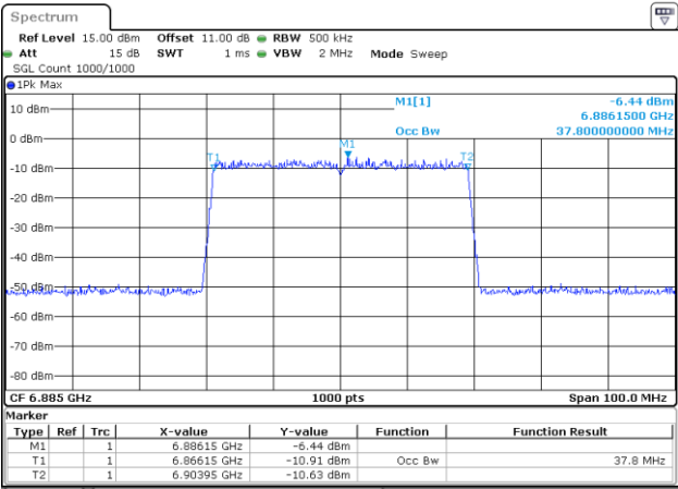
802.11be40_6885MHz_RU_484/65_Chain 0
