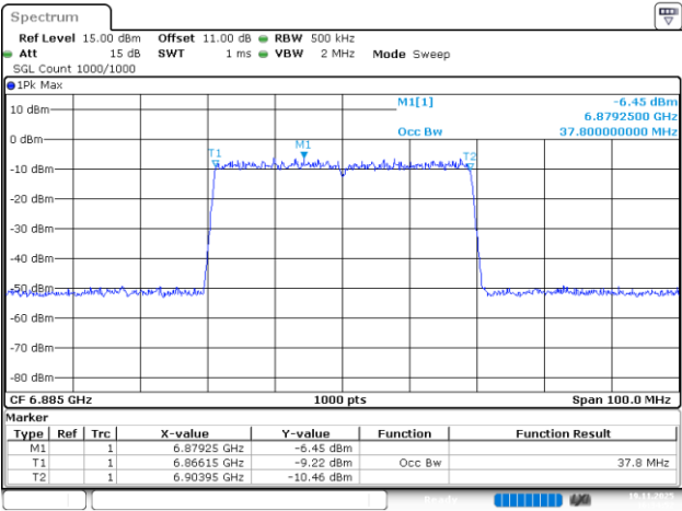
802.11be40_6885MHz_RU_484/65_Chain 3
