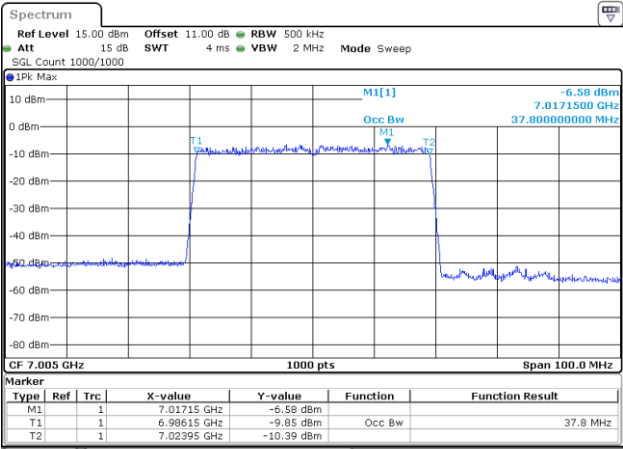
802.11be40_7005MHz_RU_484/65_Chain 0
