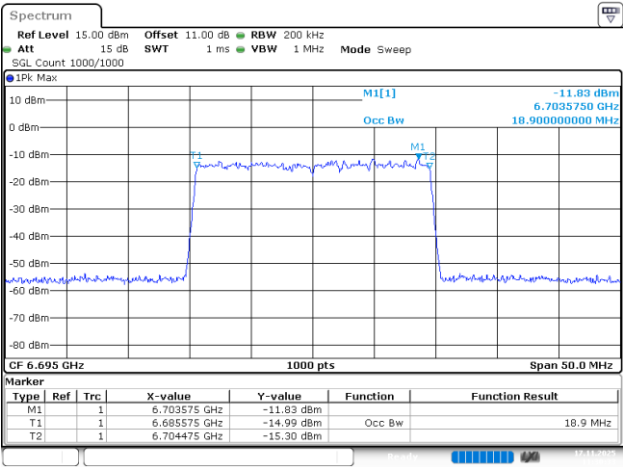
802.11be20_6695MHz_RU_242/61_Chain 3
