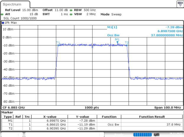
802.11be40_6885MHz_RU_484/65_Chain 2
