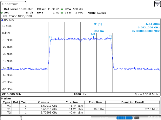
802.11be40_6685MHz_RU_484/65_Chain 2
