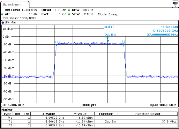
802.11be40_6885MHz_RU_484/65_Chain 1
