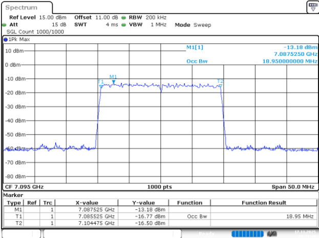
802.11be20_7095MHz_RU_242/61_Chain 1
