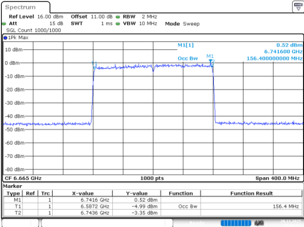
802.11be160_6665MHz_RU_2*996_Chain 2
