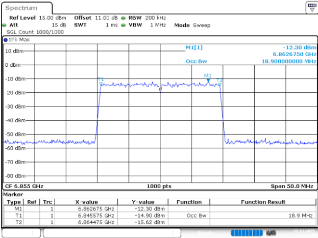
802.11be20_6855MHz_RU_242/61_Chain 3
