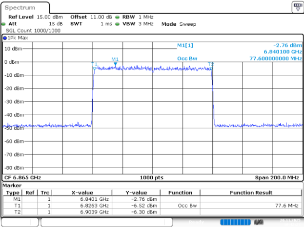
802.11be80_6865MHz_RU_996/67_Chain 3
