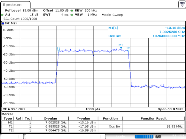
802.11be20_6995MHz_RU_242/61_Chain 3
