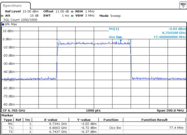
802.11be80_6705MHz_RU_996/67_Chain 2
