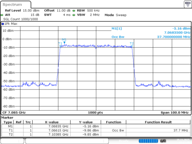
802.11be40_7085MHz_RU_484/65_Chain 3
