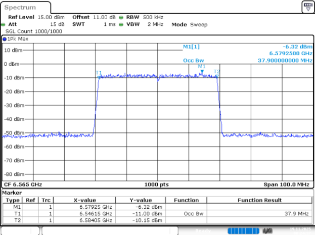
802.11be40_6565MHz_RU_484/65_Chain 1
