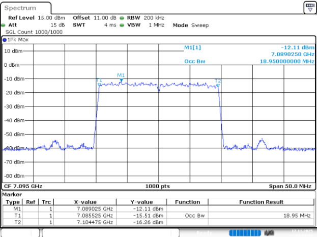
802.11be20_7095MHz_RU_242/61_Chain 3
