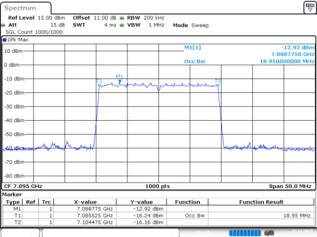
802.11be20_7095MHz_RU_242/61_Chain 2
