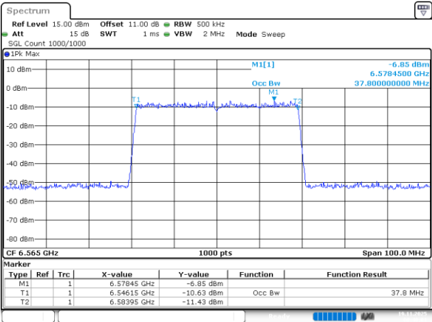
802.11be40_6565MHz_RU_484/65_Chain 2
