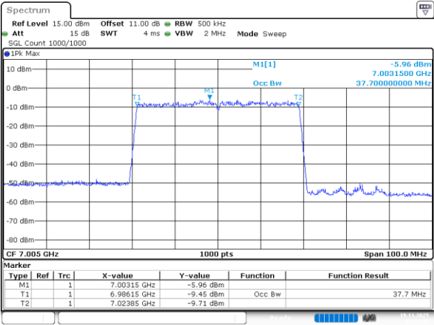
802.11be40_7005MHz_RU_484/65_Chain 3
