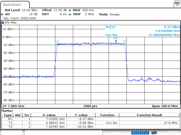
802.11be40_7005MHz_RU_484/65_Chain 2
