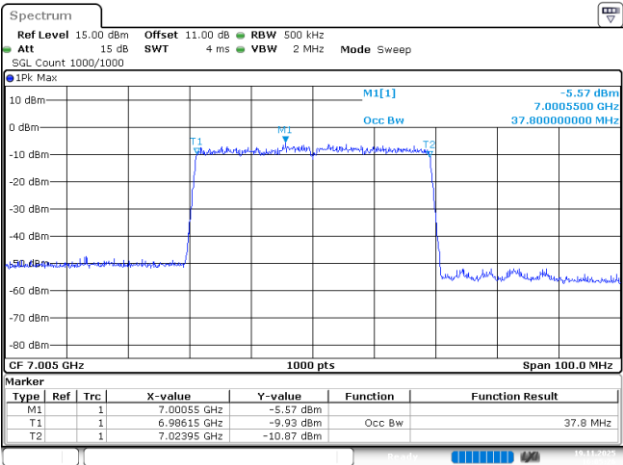
802.11be40_7005MHz_RU_484/65_Chain 1
