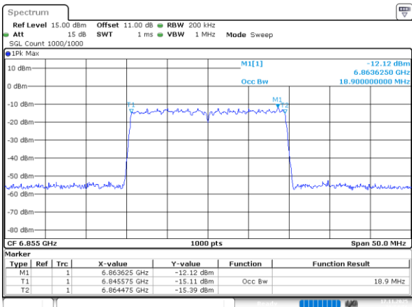
802.11be20_6855MHz_RU_242/61_Chain 1
