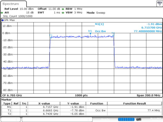
802.11be80_6705MHz_RU_996/67_Chain 3
