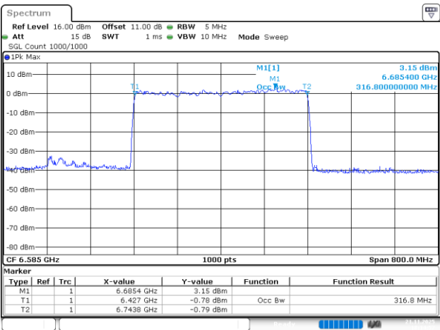
802.11be320_6585MHz_RU_4*996_Chain 2
