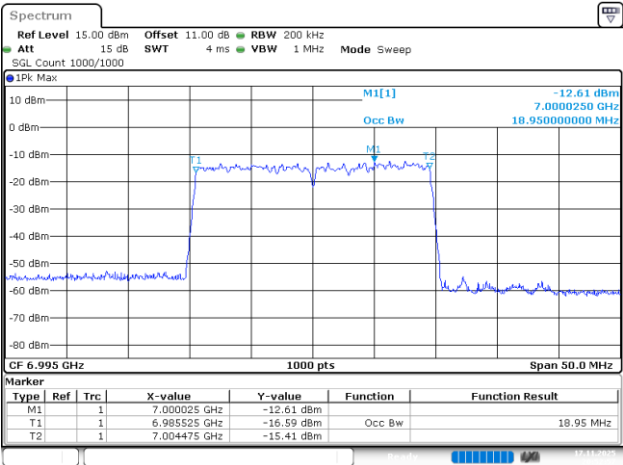
802.11be20_6995MHz_RU_242/61_Chain 2
