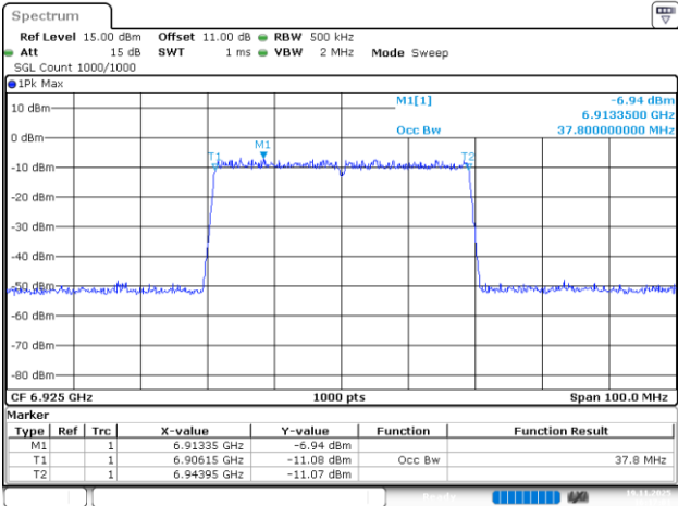
802.11be40_6925MHz_RU_484/65_Chain 2
