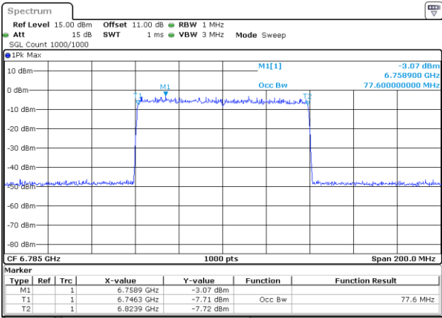
802.11be80_6785MHz_RU_996/67_Chain 1
