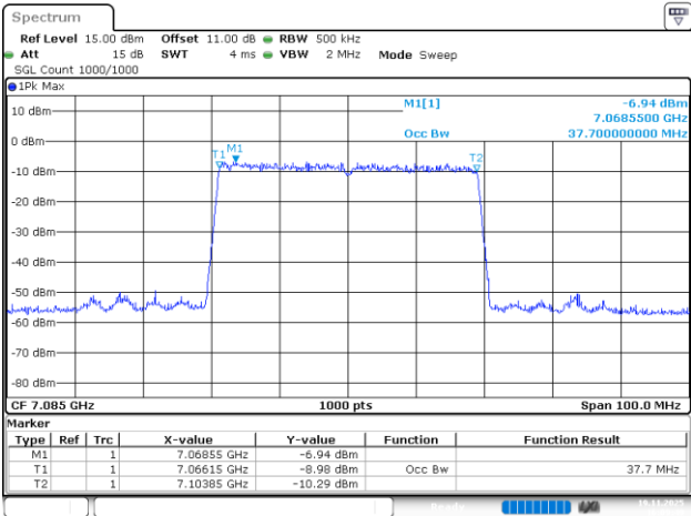
802.11be40_7085MHz_RU_484/65_Chain 1
