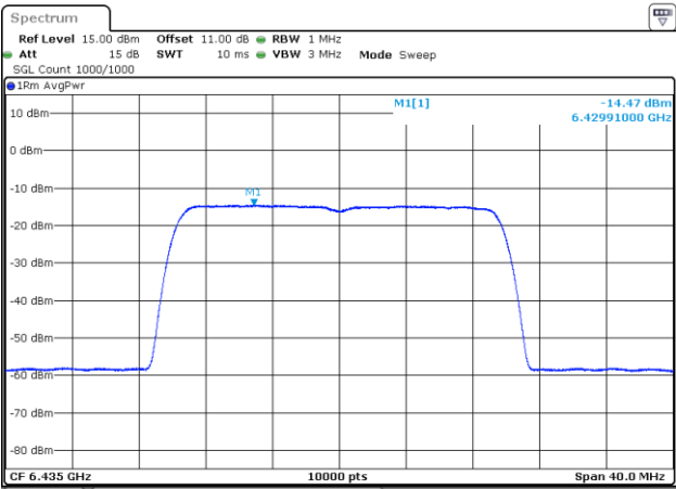
802.11be20_6435MHz_RU_242/61_Chain 2
