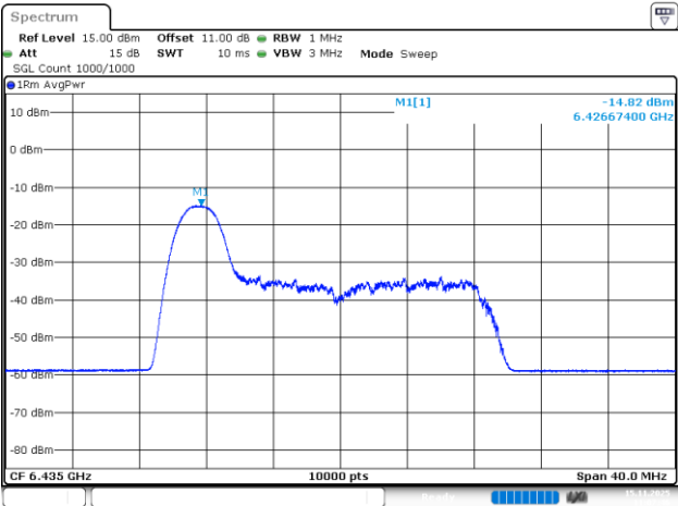
802.11be20_6435MHz_RU_26/0_Chain 2
