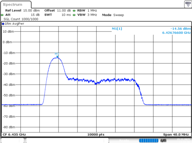
802.11be20_6435MHz_RU_26/0_Chain 3
