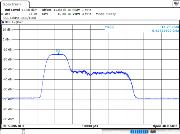
802.11be20_6435MHz_RU_52/37_Chain 3
