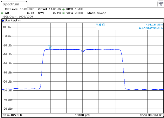
802.11be40_6485MHz_RU_484/65_Chain 1
