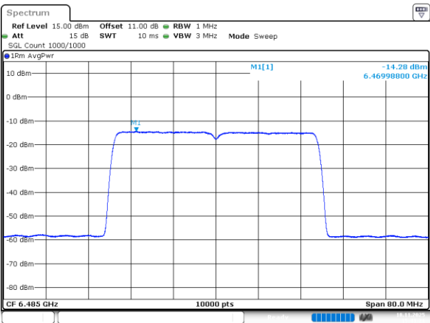
802.11be40_6485MHz_RU_484/65_Chain 0
