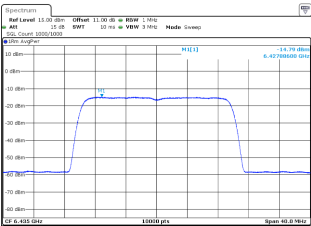
802.11be20_6435MHz_RU_242/61_Chain 3
