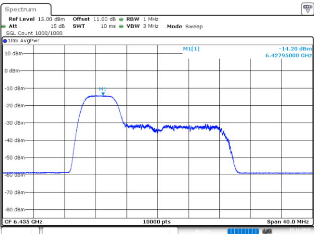
802.11be20_6435MHz_RU_52/37_Chain 1
