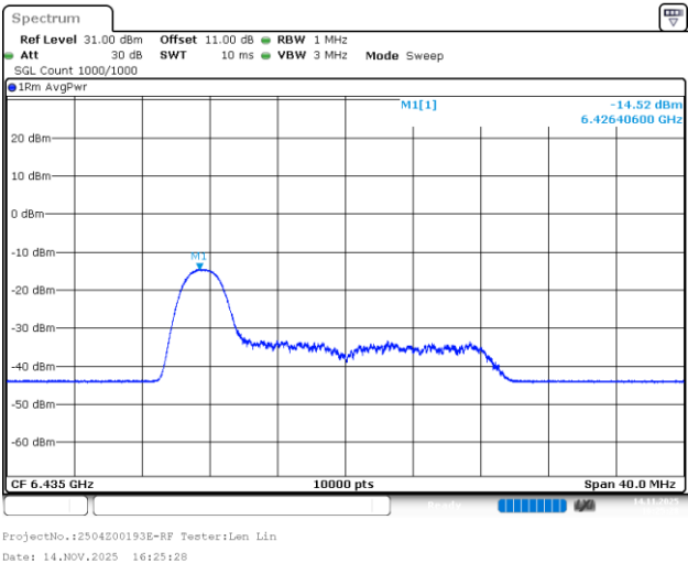
802.11be20_6435MHz_RU_26/0_Chain 1
