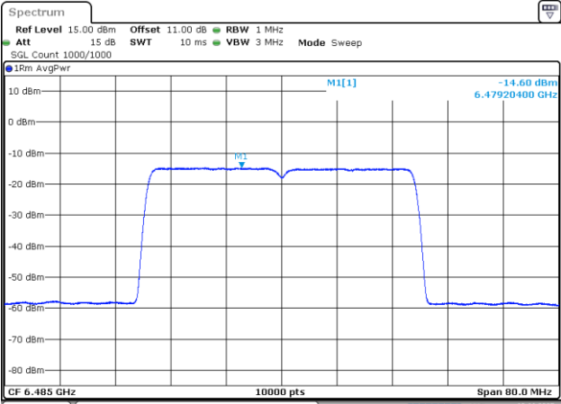
802.11be40_6485MHz_RU_484/65_Chain 2
