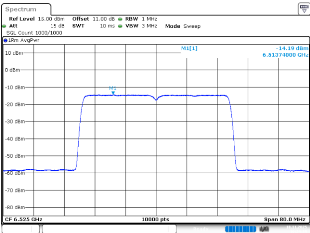
802.11be40_6525MHz_RU_484/65_Chain 1
