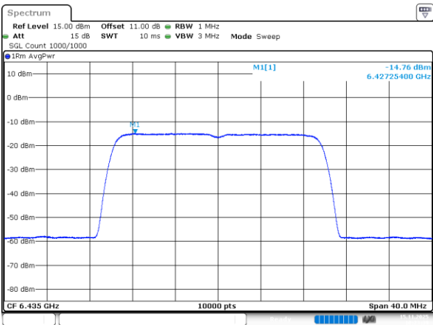
802.11be20_6435MHz_RU_242/61_Chain 1
