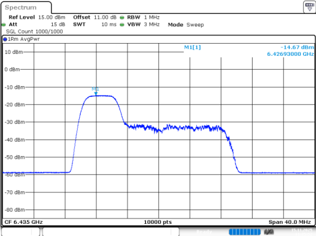
802.11be20_6435MHz_RU_52/37_Chain 0
