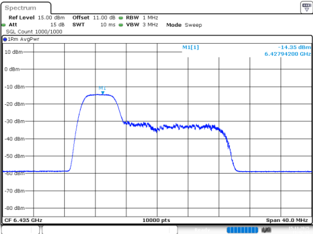
802.11be20_6435MHz_RU_52/37_Chain 2
