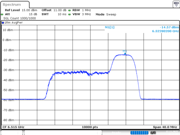
802.11be20_6515MHz_RU_52/40_Chain 2
