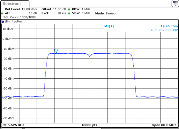
802.11be40_6525MHz_RU_484/65_Chain 2
