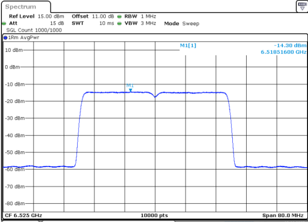
802.11be40_6525MHz_RU_484/65_Chain 3
