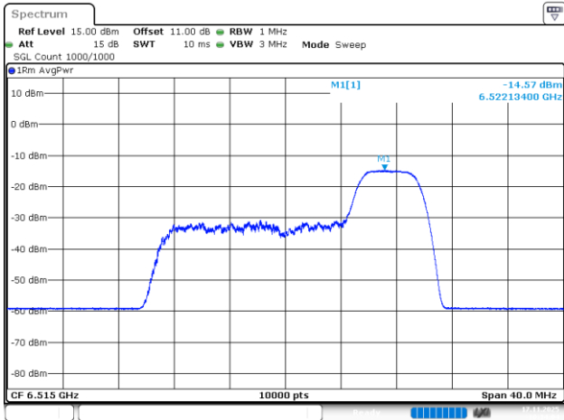
802.11be20_6515MHz_RU_52/40_Chain 3
