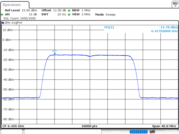
802.11be20_6435MHz_RU_242/61_Chain 0
