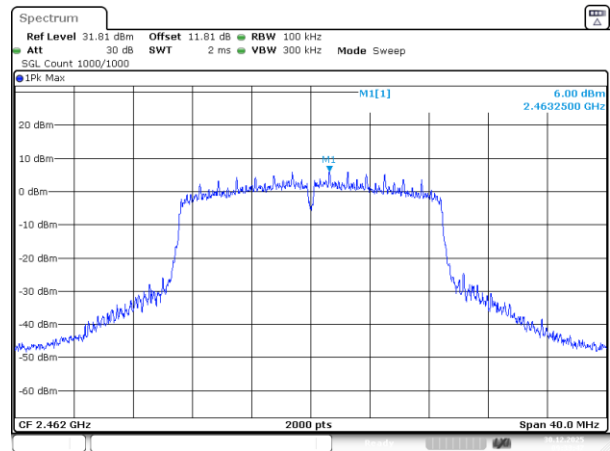
802.11n20_2462MHz_Chain 2
