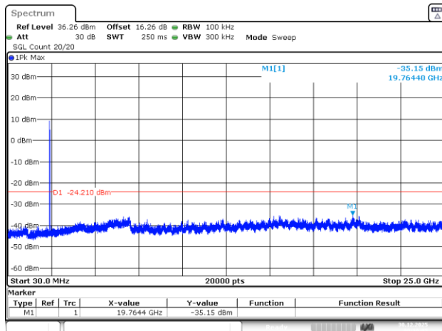
802.11n20_2412MHz_Chain 3
