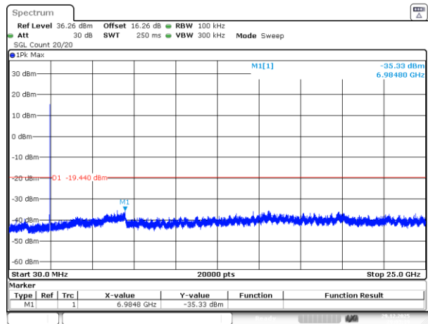
802.11b_2462MHz_Chain 3
