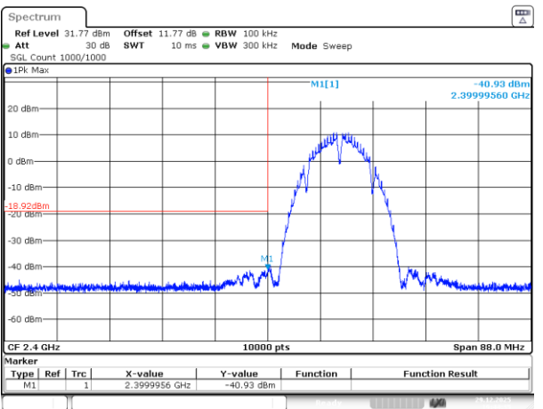
802.11b_2412MHz_Chain 2
