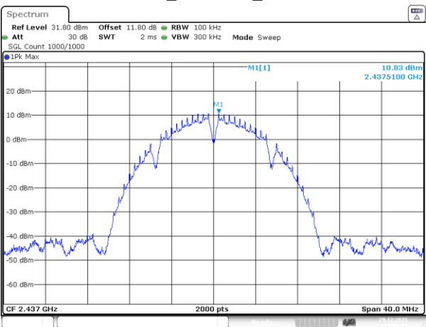
802.11b_2437MHz_Chain 3
