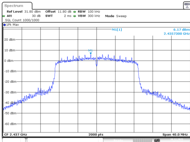
802.11n20_2437MHz_Chain 3
