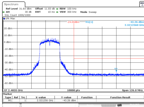
802.11n20_2462MHz_Chain 2
