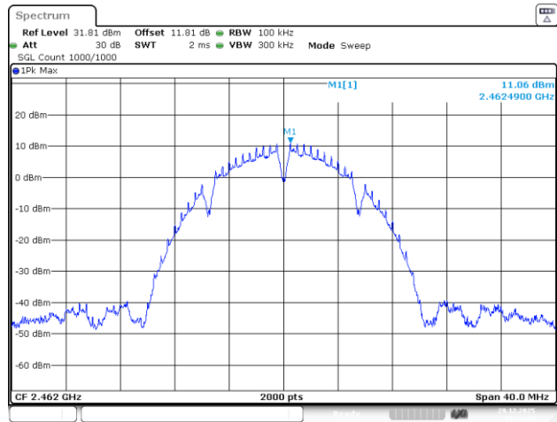
802.11b_2462MHz_Chain 2
