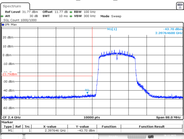
802.11n20_2412MHz_Chain 1
