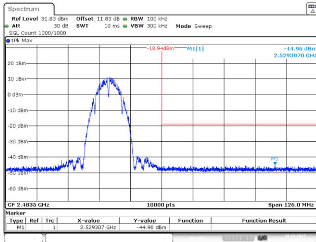
802.11b_2462MHz_Chain 2
