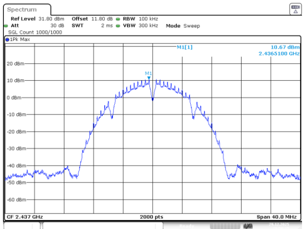
802.11b_2437MHz_Chain 1
