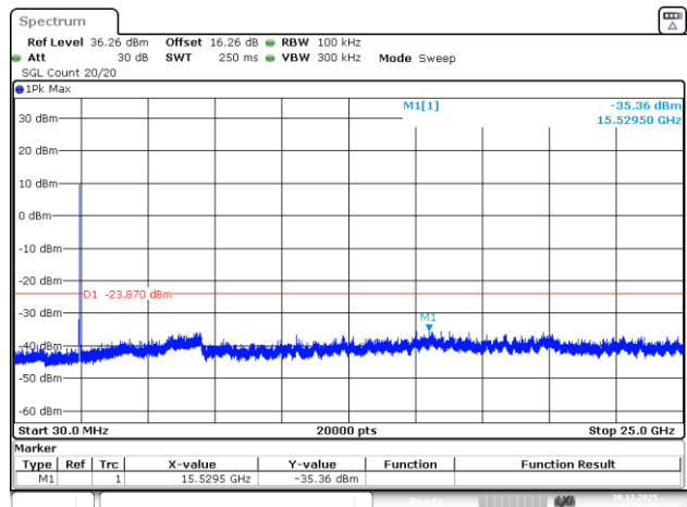
802.11n20_2462MHz_Chain 3
