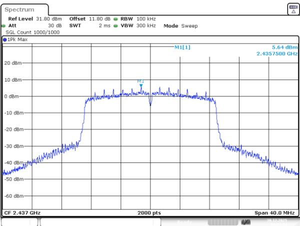
802.11n20_2437MHz_Chain 1
