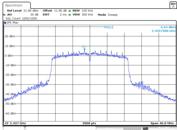
802.11n20_2437MHz_Chain 2
