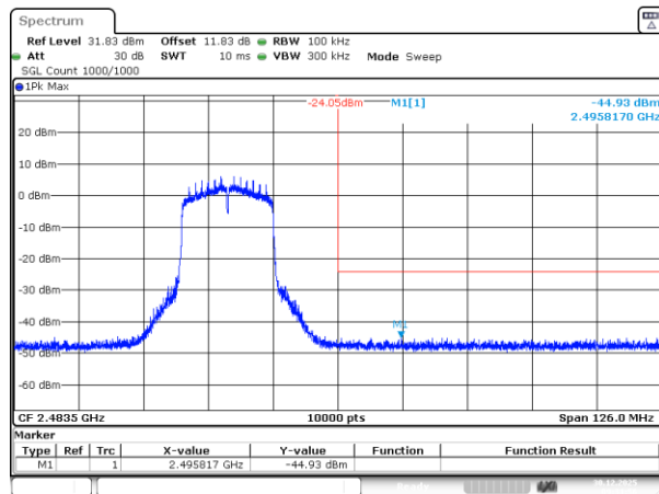
802.11n20_2462MHz_Chain 1
