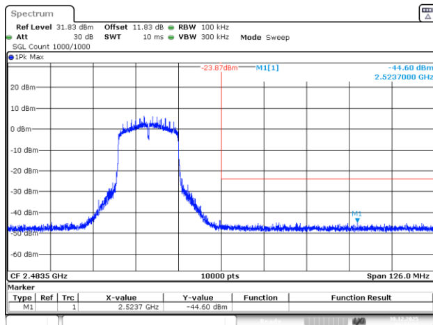
802.11n20_2462MHz_Chain 3
