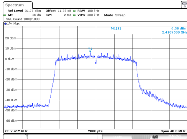
802.11n20_2412MHz_Chain 2
