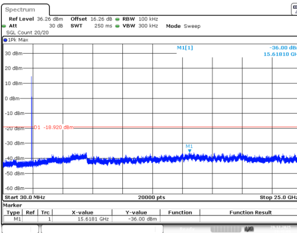
802.11b_2412MHz_Chain 2
