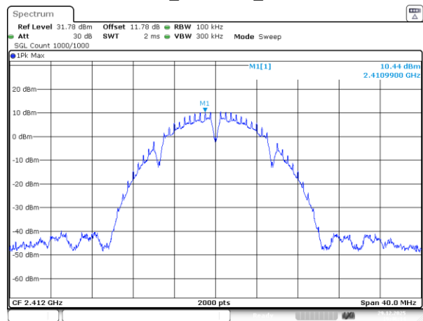
802.11b_2412MHz_Chain 3
