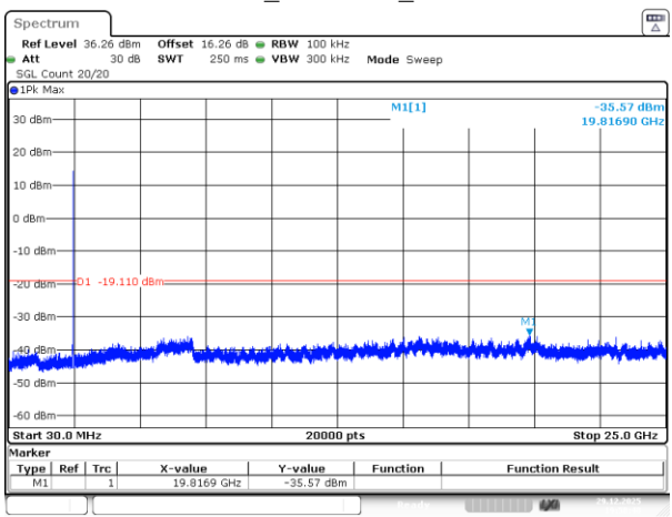
802.11b_2462MHz_Chain 1
