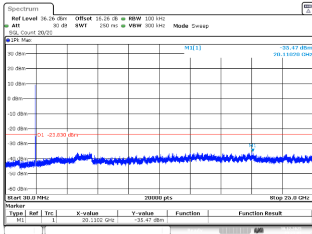
802.11n20_2437MHz_Chain 3
