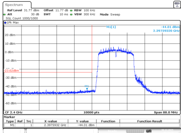
802.11n20_2412MHz_Chain 2
