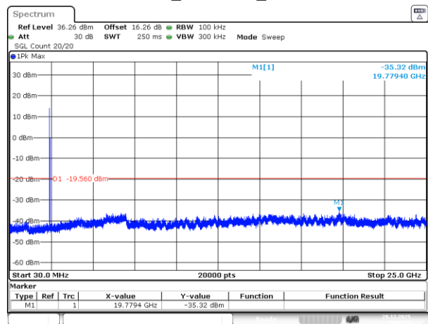
802.11b_2412MHz_Chain 3
