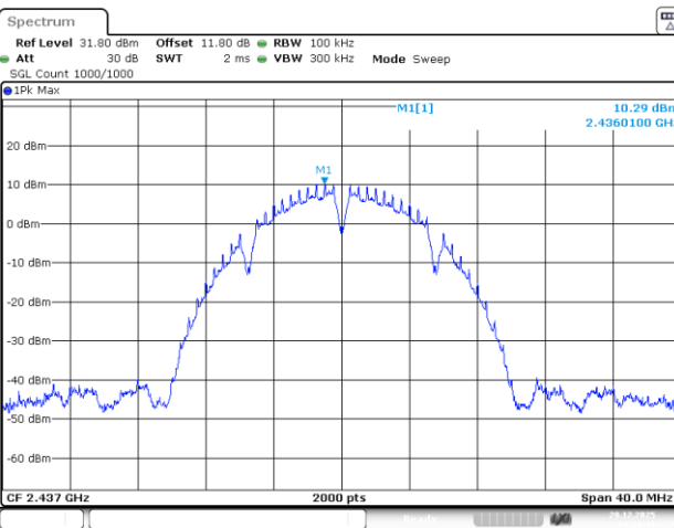
802.11b_2437MHz_Chain 2
