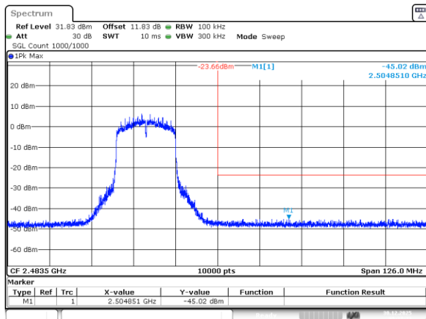
802.11n20_2462MHz_Chain 0
