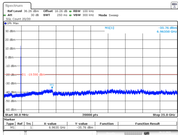
802.11b_2412MHz_Chain 1
