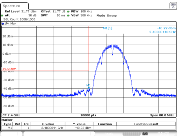
802.11b_2412MHz_Chain 3
