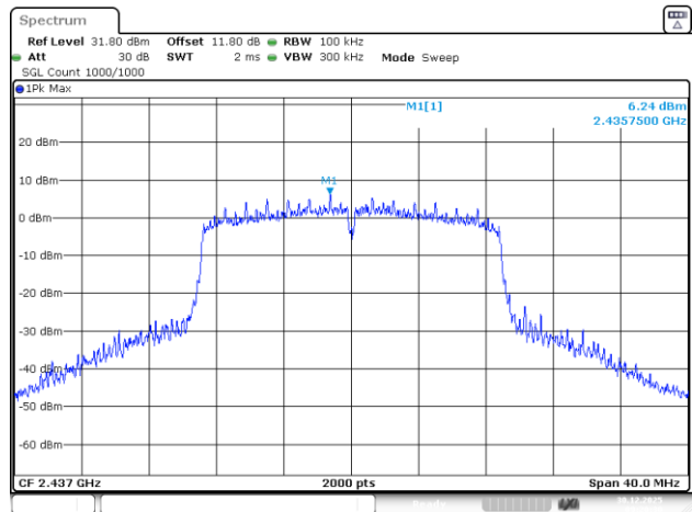
802.11n20_2437MHz_Chain 0
