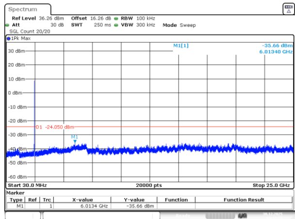
802.11n20_2462MHz_Chain 1
