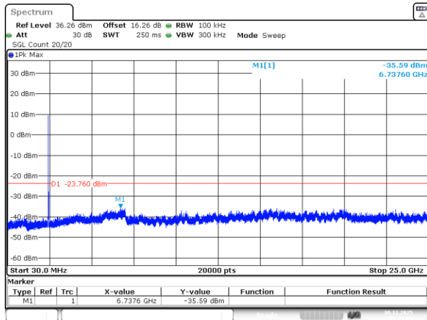
802.11n20_2437MHz_Chain 0
