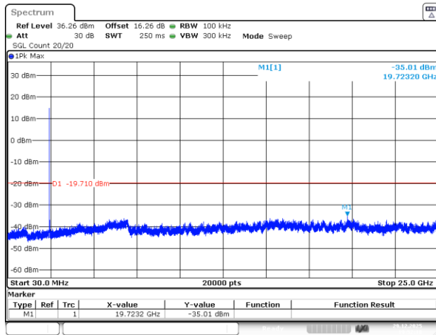
802.11b_2437MHz_Chain 2
