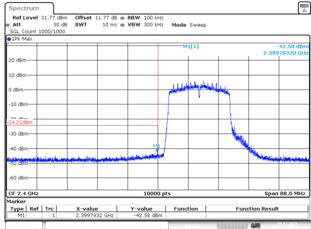
802.11n20_2412MHz_Chain 3
