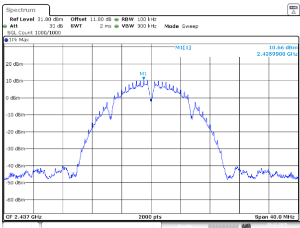
802.11b_2437MHz_Chain 0
