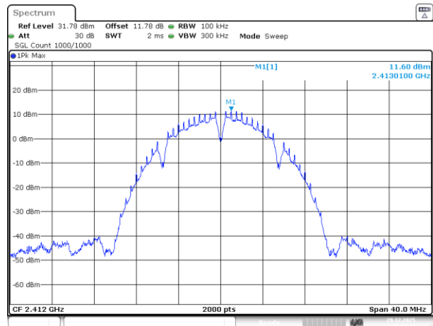
802.11b_2412MHz_Chain 0
