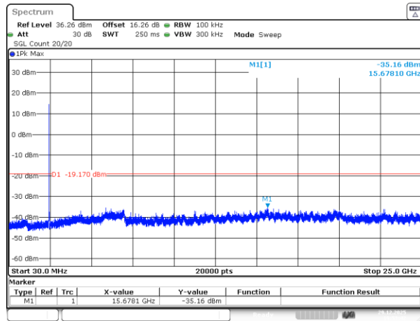
802.11b_2437MHz_Chain 3
