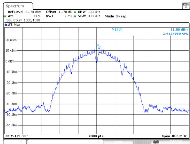
802.11b_2412MHz_Chain 2
