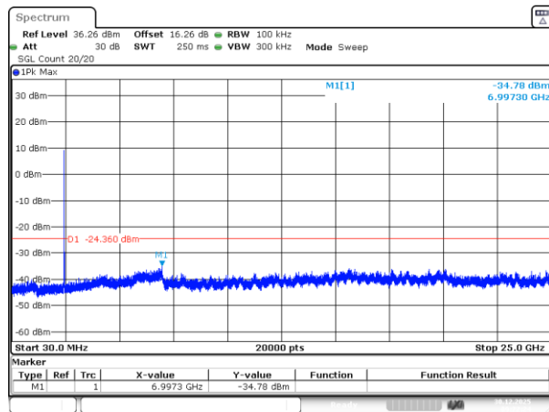
802.11n20_2437MHz_Chain 1
