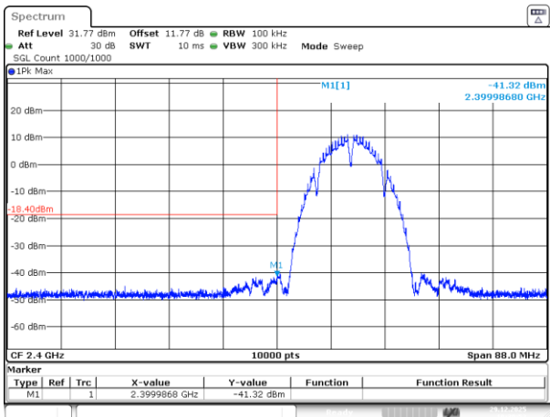
802.11b_2412MHz_Chain 0
