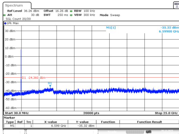
802.11n20_2437MHz_Chain 2
