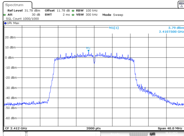
802.11n20_2412MHz_Chain 3
