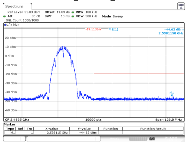
802.11b_2462MHz_Chain 1
