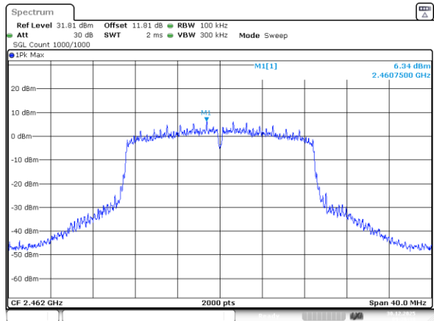
802.11n20_2462MHz_Chain 0
