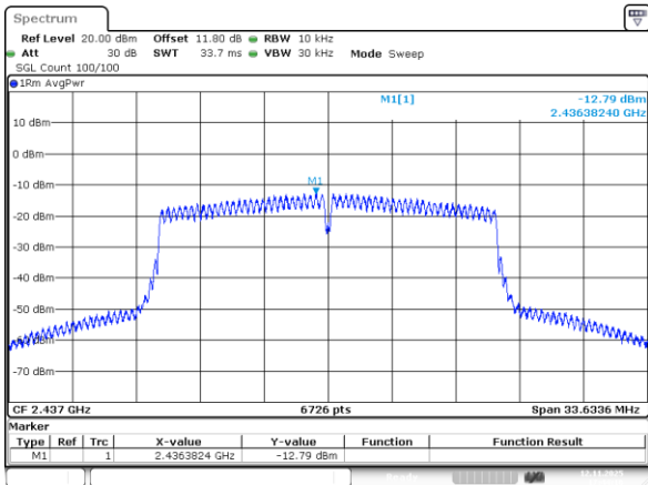
802.11n20_2437MHz_Chain 3
