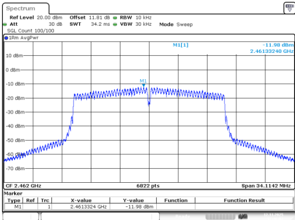
802.11n20_2462MHz_Chain 3
