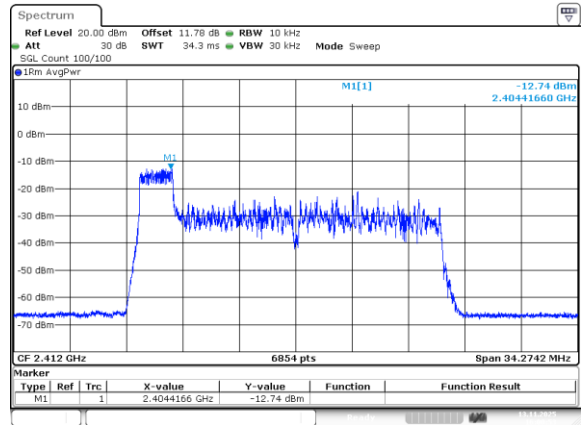
802.11be20_2412MHz_RU_26/0_Chain 0
