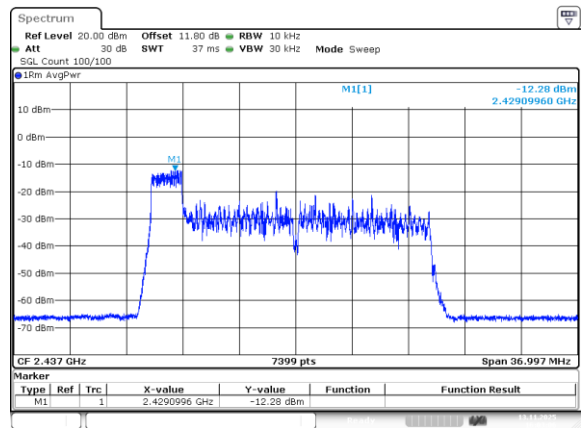
802.11be20_2437MHz_RU_26/0_Chain 1
