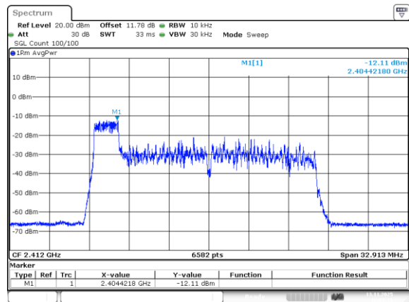
802.11be20_2412MHz_RU_26/0_Chain 1
