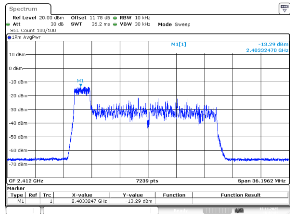
802.11be20_2412MHz_RU_26/0_Chain 3
