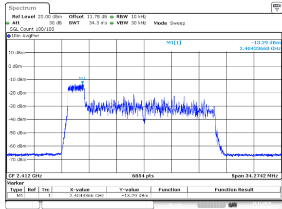
802.11be20_2412MHz_RU_26/0_Chain 2
