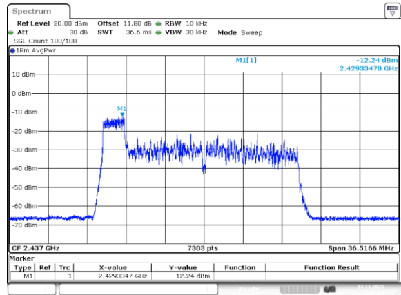
802.11be20_2437MHz_RU_26/0_Chain 2
