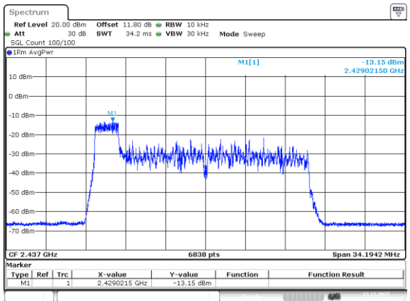
802.11be20_2437MHz_RU_26/0_Chain 3
