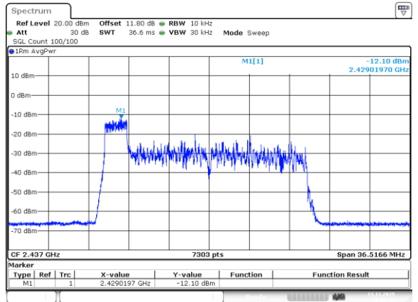
802.11be20_2437MHz_RU_26/0_Chain 0
