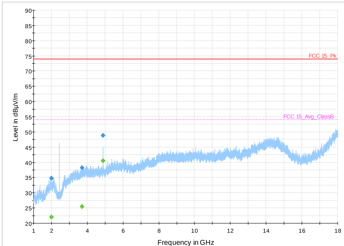
Plot 49. 1-18GHz, 2480MHz, DH5
