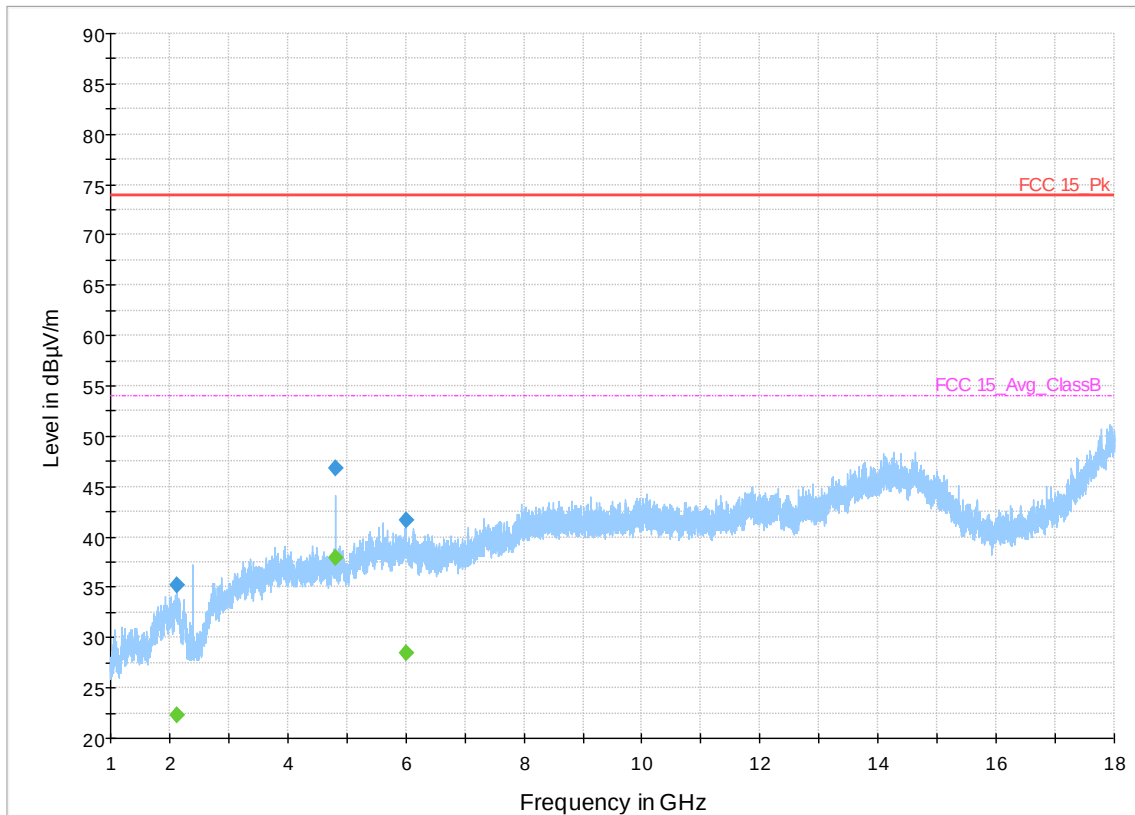
Plot 47. 1-18GHz, 2402MHz, DH5
