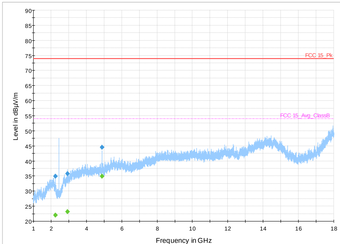
Plot 48. 1-18GHz, 2441MHz, DH5
