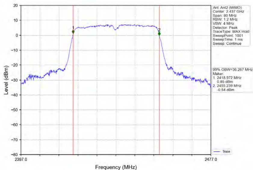
802.11n(HT40)_MCH_2437MHz_Ant2 (MIMO)_NTNV
