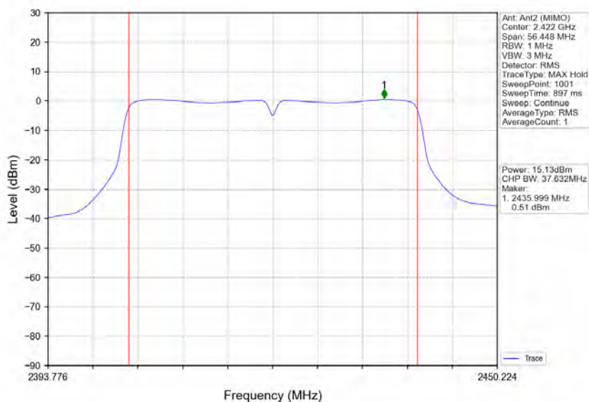
802.11n(HT40)_LCH_2422MHz_Ant2 (MIMO)_NTNV
