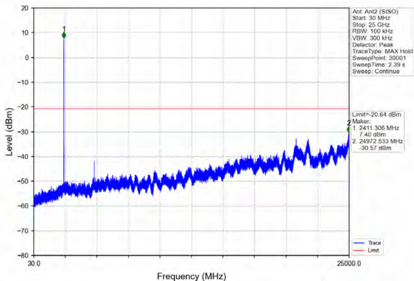
802.11b_LCH_2412MHz_Ant2 (SISO)_NTNV
