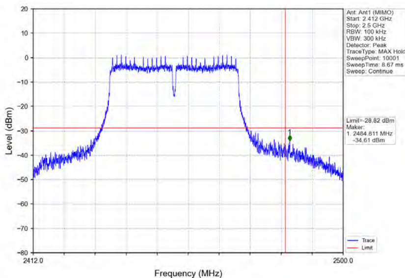
802.11n(HT40)_HCH_2452MHz_Ant1 (MIMO)_NTNV
