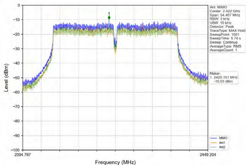
802.11n(HT40)_LCH_2422MHz_MIMO_NTNV
