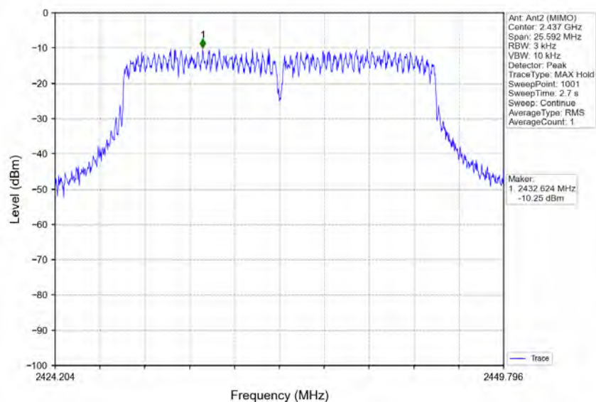
802.11n(HT20)_MCH_2437MHz_MIMO_NTNV
