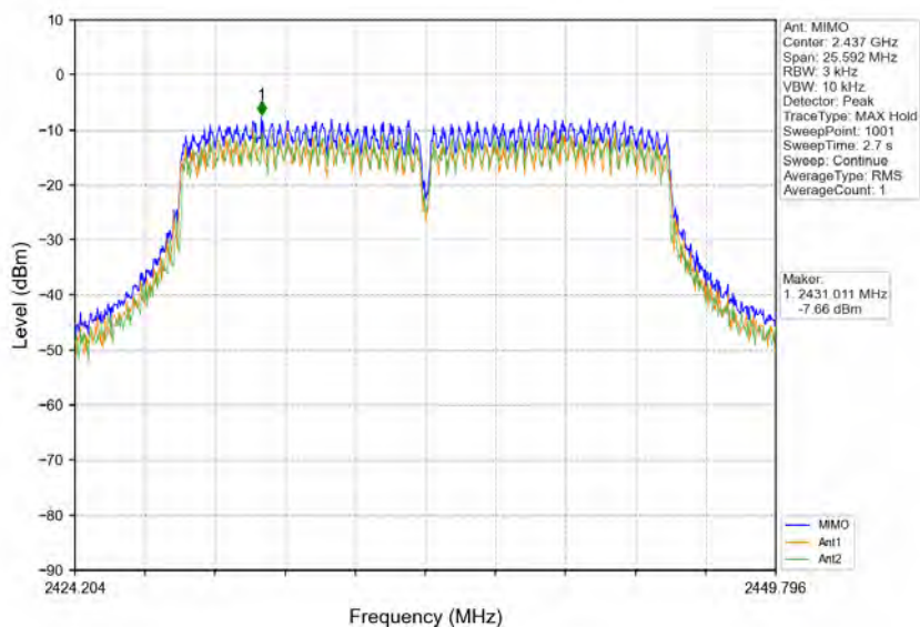
802.11n(HT20)_MCH_2437MHz_MIMO_NTNV
