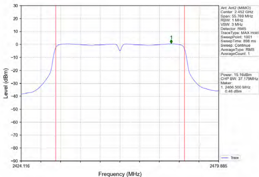
802.11n(HT40)_HCH_2452MHz_Ant2 (MIMO)_NTNV
