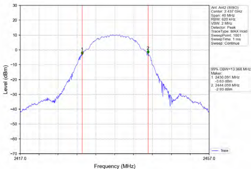
802.11b_MCH_2437MHz_Ant2 (SISO)_NTNV
