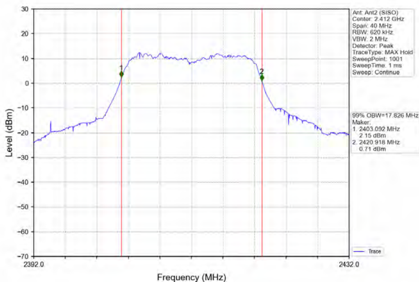
802.11g_LCH_2412MHz_Ant2 (SISO)_NTNV
