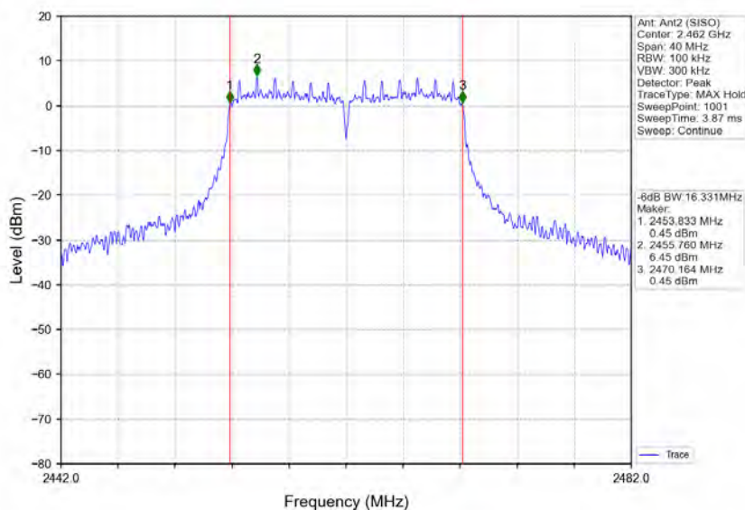
802.11g_HCH_2462MHz_Ant2 (SISO)_NTNV
