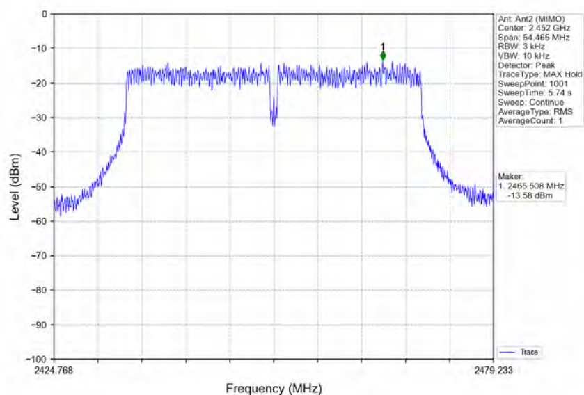
802.11n(HT40)_HCH_2452MHz_MIMO_NTNV
