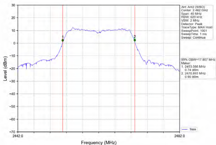
802.11g_HCH_2462MHz_Ant2 (SISO)_NTNV
