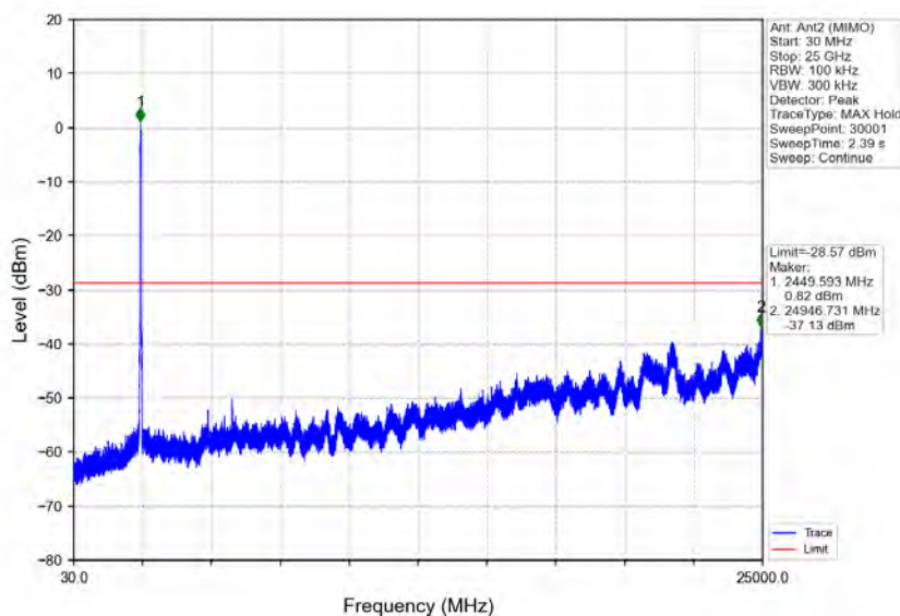
802.11n(HT40)_HCH_2452MHz_Ant2 (MIMO)_NTNV
