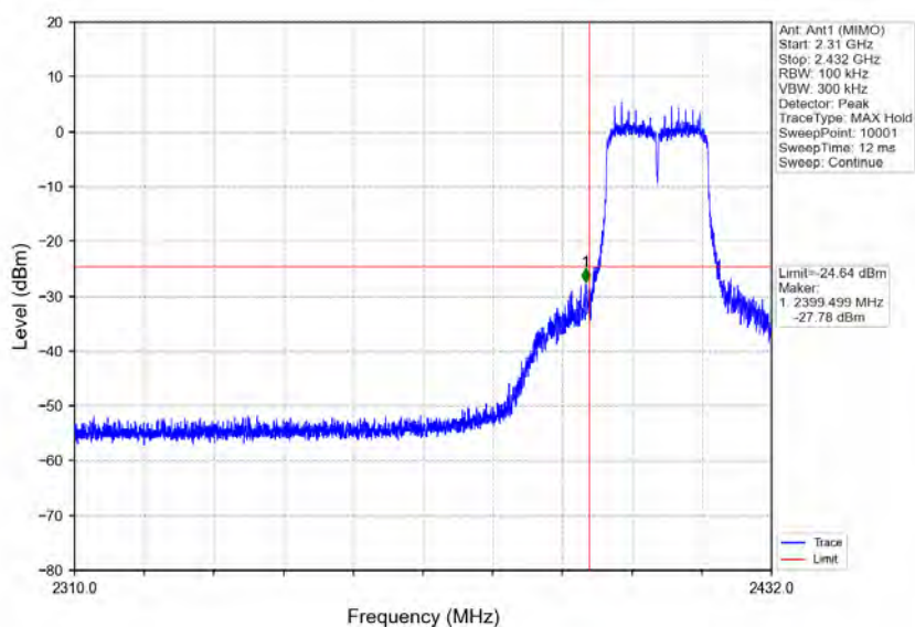
802.11n(HT20)_LCH_2412MHz_Ant1 (MIMO)_NTNV
