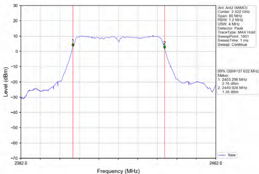
802.11n(HT40)_LCH_2422MHz_Ant2 (MIMO)_NTNV
