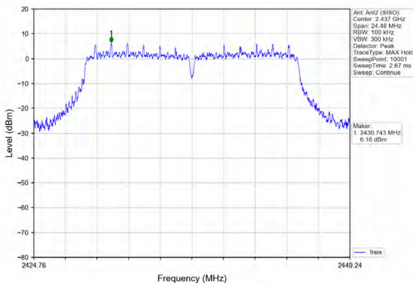
802.11g_MCH_2437MHz_Ant2 (SISO)_NTNV
