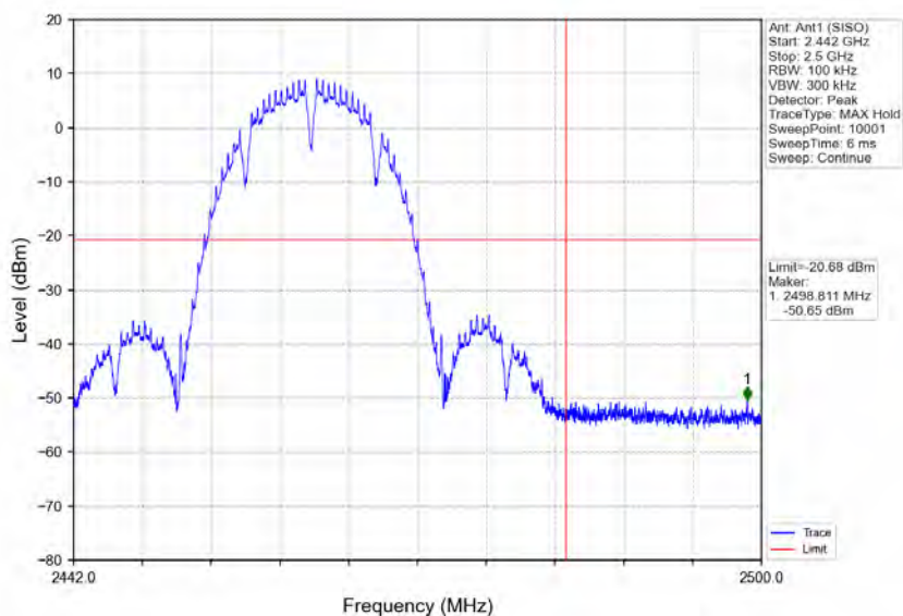
802.11b_HCH_2462MHz_Ant1 (SISO)_NTNV
