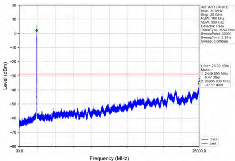
802.11n(HT40)_HCH_2452MHz_Ant1 (MIMO)_NTNV
