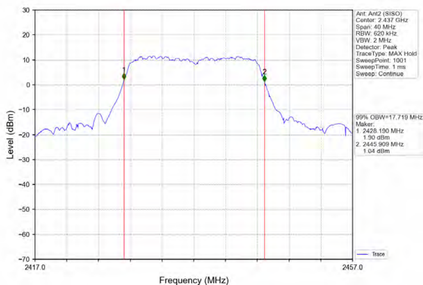
802.11g_MCH_2437MHz_Ant2 (SISO)_NTNV
