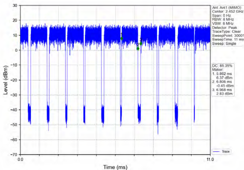
802.11n(HT40)_HCH_2452MHz_Ant1 (MIMO)_NTNV
