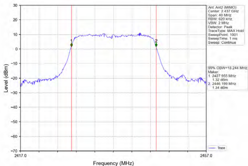
802.11n(HT20)_MCH_2437MHz_Ant2 (MIMO)_NTNV
