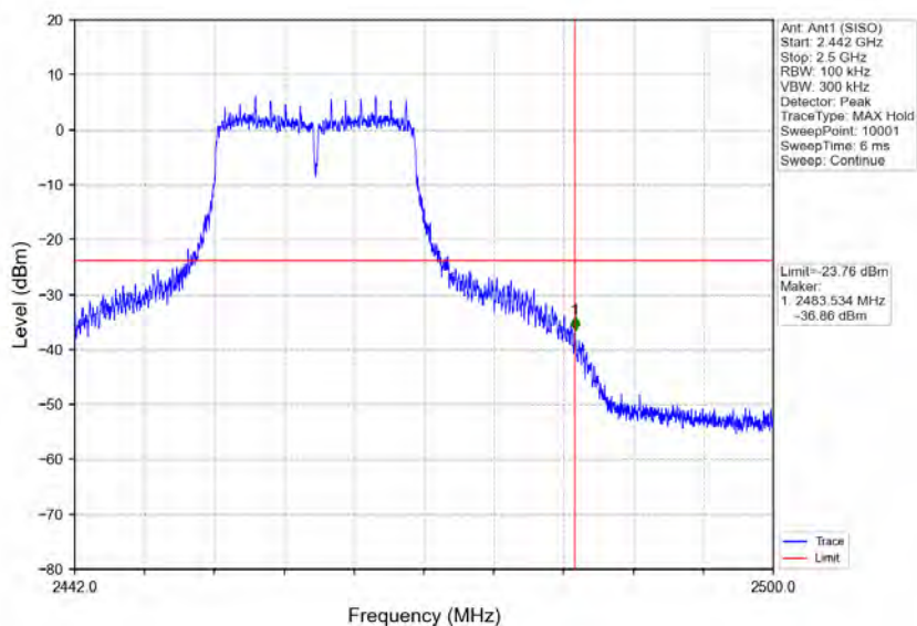
802.11g_HCH_2462MHz_Ant1 (SISO)_NTNV
