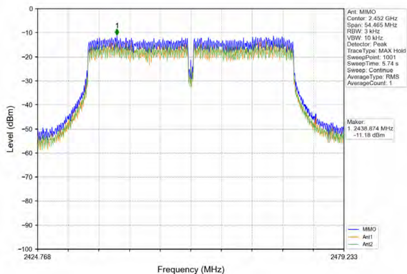
802.11n(HT40)_HCH_2452MHz_MIMO_NTNV
