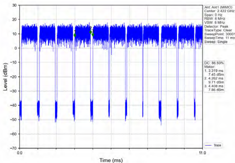
802.11n(HT40)_LCH_2422MHz_Ant1 (MIMO)_NTNV
