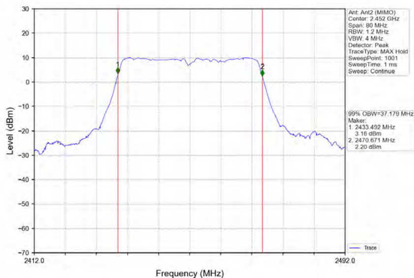
802.11n(HT40)_HCH_2452MHz_Ant2 (MIMO)_NTNV
