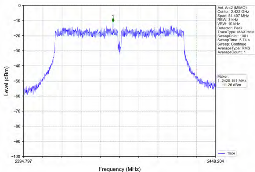
802.11n(HT40)_LCH_2422MHz_MIMO_NTNV
