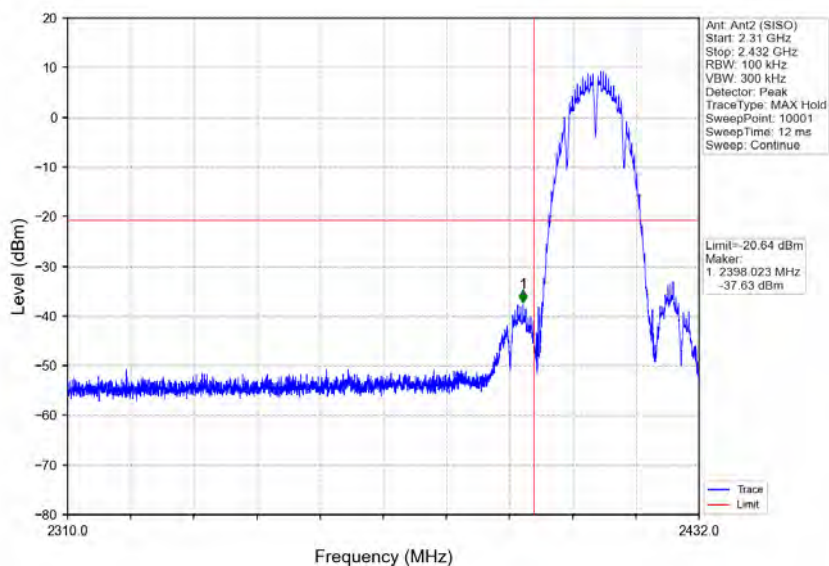
802.11b_LCH_2412MHz_Ant2 (SISO)_NTNV
