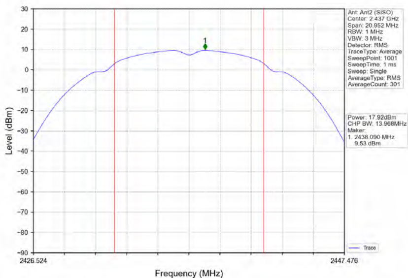
802.11b_MCH_2437MHz_Ant2 (SISO)_NTNV
