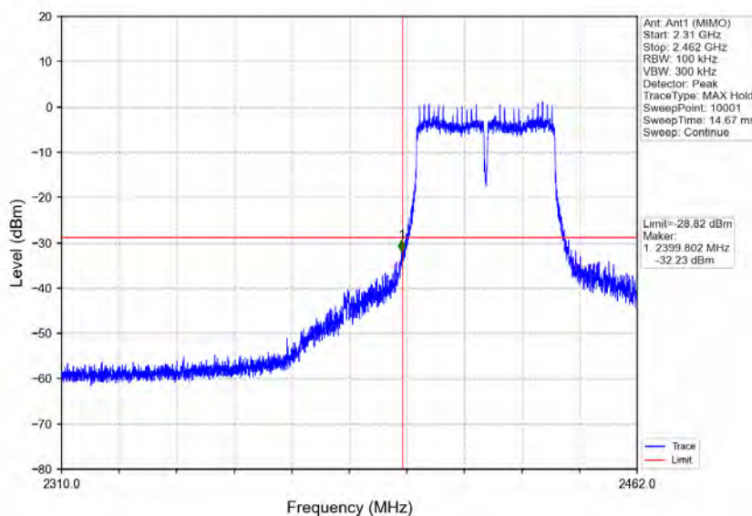
802.11n(HT40)_LCH_2422MHz_Ant1 (MIMO)_NTNV
