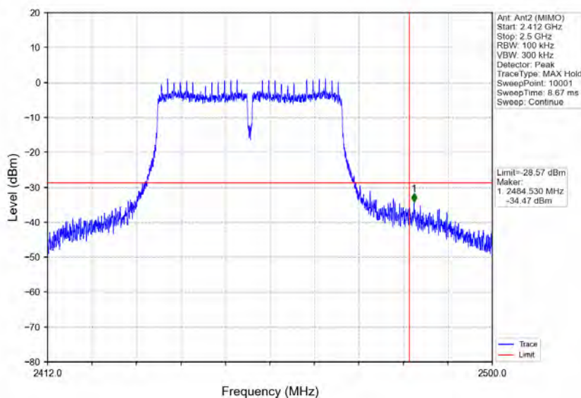
802.11n(HT40)_HCH_2452MHz_Ant2 (MIMO)_NTNV
