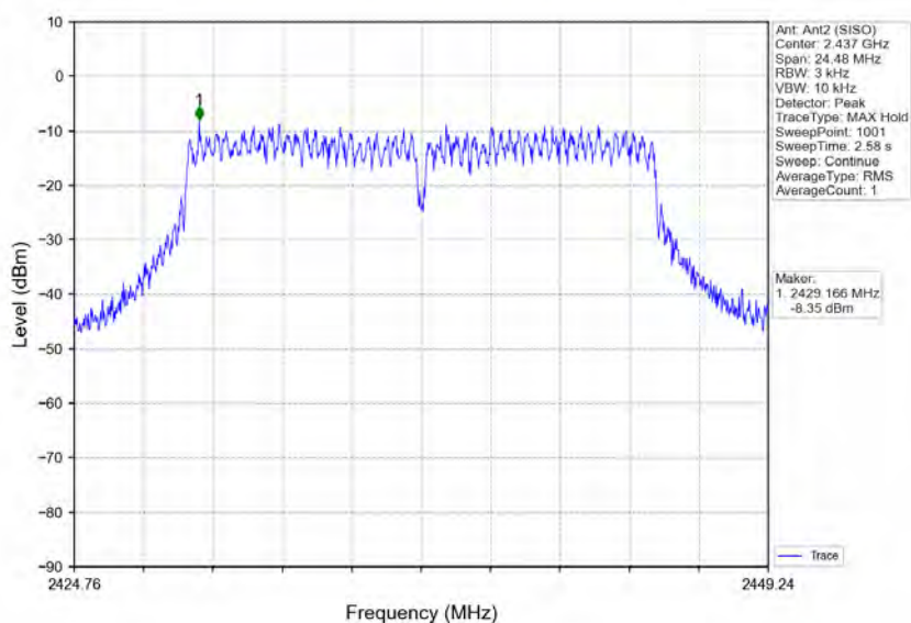
802.11g_MCH_2437MHz_Ant2 (SISO)_NTNV
