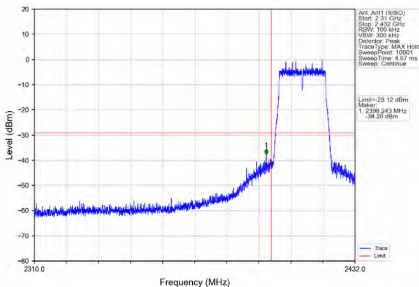
802.11n(HT20)_LCH_2412MHz_Ant1 (SISO) NTNV
