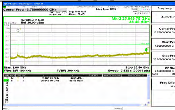
11N20MIMO_Ant2_2412_1000~26500
