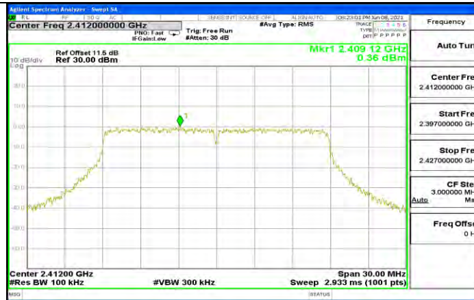
11N20MIMO_Ant2_2412_0~Reference
