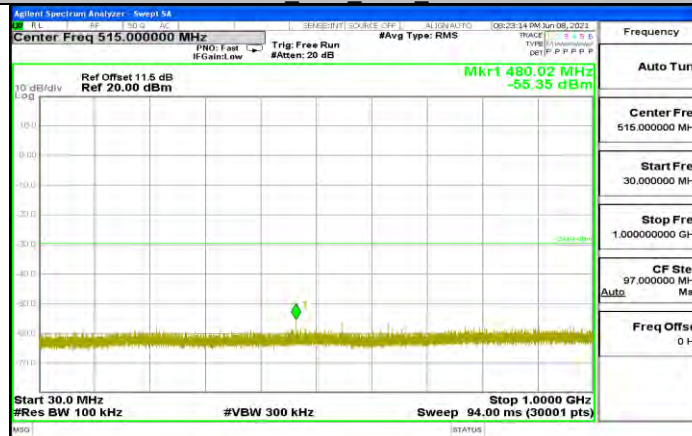
11N20MIMO_Ant2_2412_30~1000
