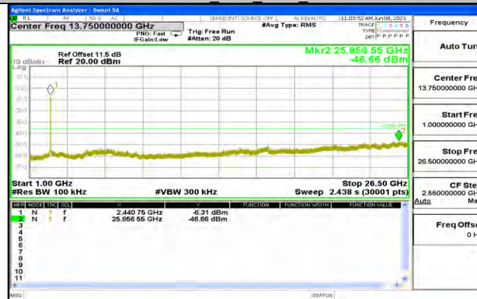
11N40SISO Ant1 2437 1000~26500
