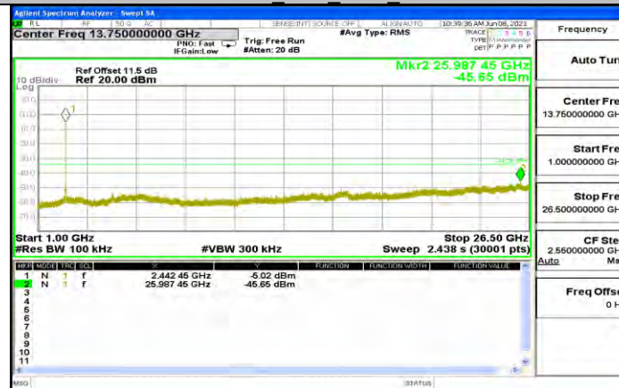
11N20SISO Ant1 2437 1000~26500
