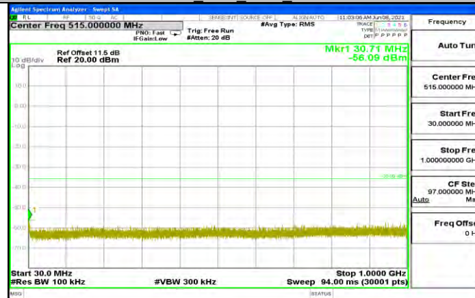
11N40SISO Ant1 2437 30~1000
