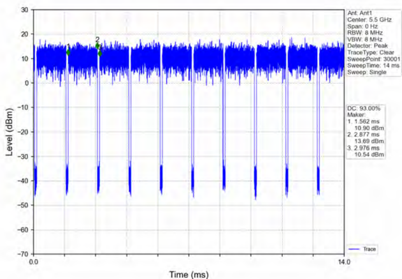
802.11ac(VHT20) LCH 5500MHz Ant1 NTNV
