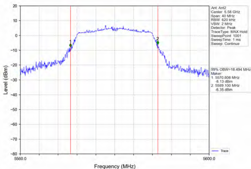
802.11a_MCH_5580MHz_Ant2_NTNV
