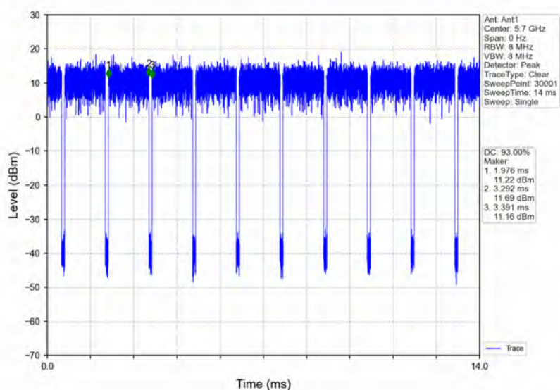
802.11ac(VHT20)_HCH_5700MHz_Ant1_NTNV
