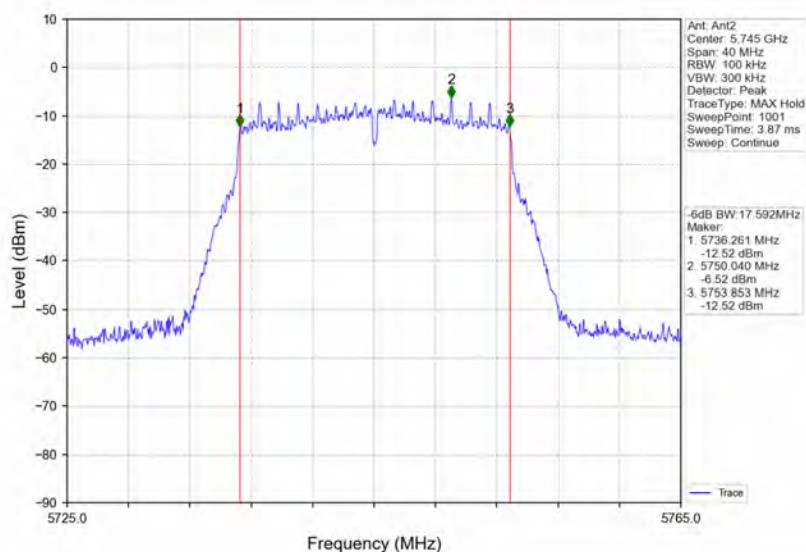
802.11n(HT20) LCH_5745MHz_Ant2_NTNV
