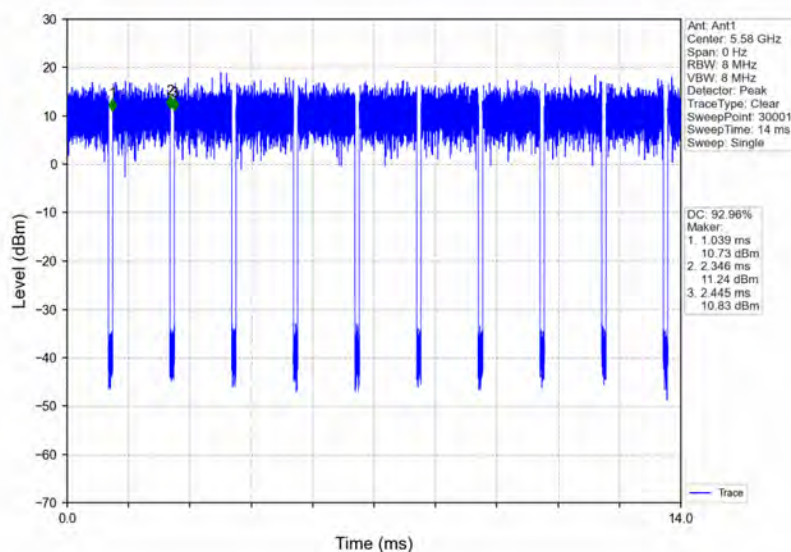
802.11n(HT20) MCH 5580MHz Ant1 NTVN
