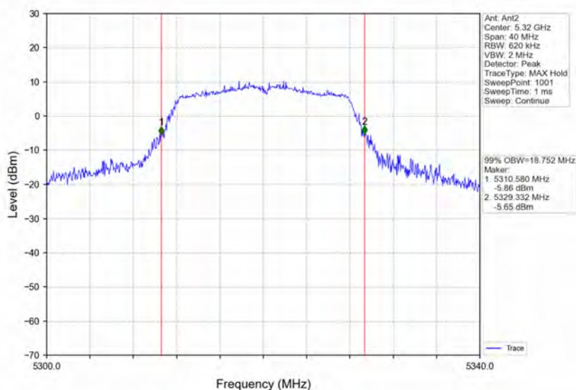
802.11a_HCH_5320MHz_Ant2_NTNV
