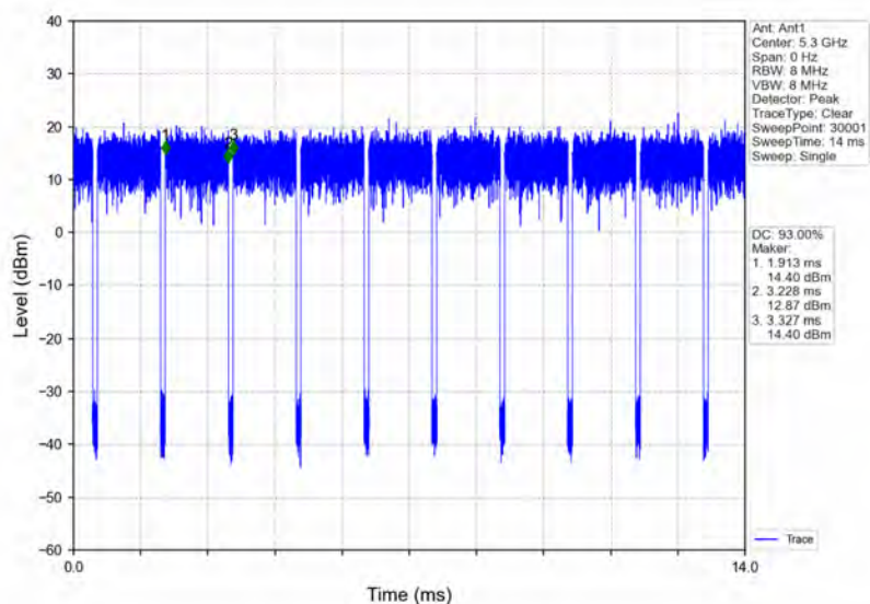
802.11ac(VHT20) MCH 5300MHz Ant1 NTNV
