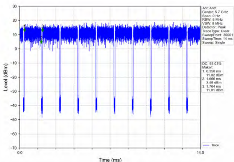
802.11n(HT20) LCH 5745MHz Ant1 NTVN
