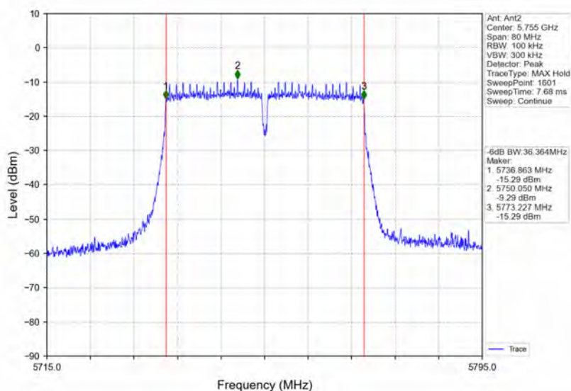
802.11n(HT40) LCH_5755MHz_Ant2_NTNV
