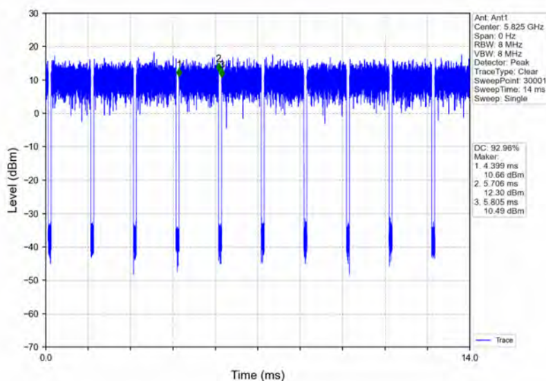
802.11n(HT20) HCH 5825MHz Ant1 NTN
