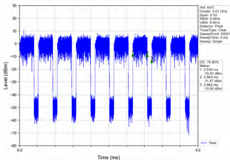
802.11ac(VHT80) HCH 5610MHz Ant1 NTNV
