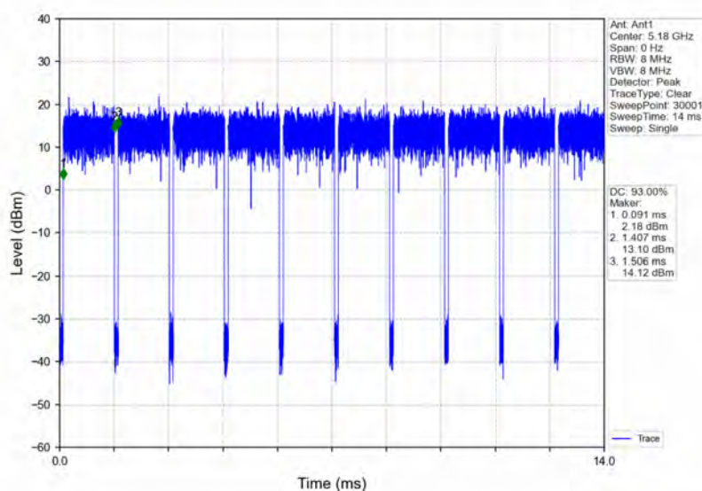
802.11ac(VHT20) LCH 5180MHz Ant1 NTN
