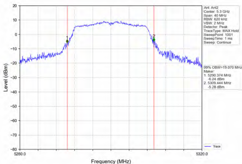
802.11a_MCH_5300MHz_Ant2_NTNV
