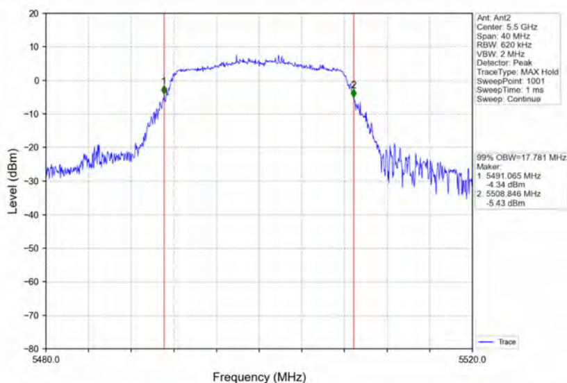
802.11a LCH_5500MHz_Ant2_NTNV
