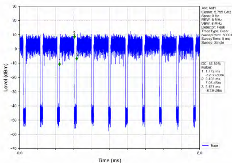
802.11ac(VHT40) HCH 5795MHz Ant1 NTNV
