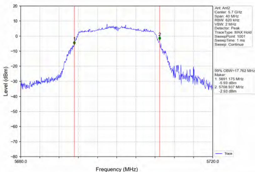
802.11a_HCH_5700MHz_Ant2_NTNV
