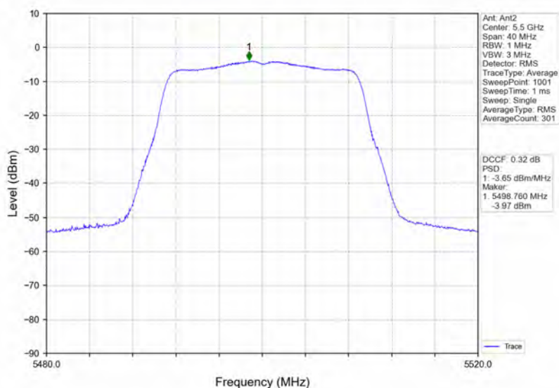
802.11n(HT20) LCH 5500MHz Ant2 NTVN
