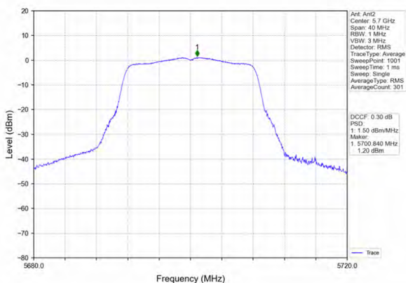
802.11a_HCH_5700MHz_Ant2_NTNV
