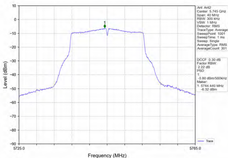
802.11a_LCH_5745MHz_Ant2_NTNV
