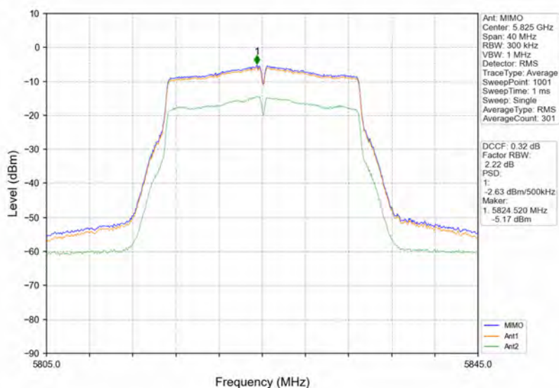
802.11ac(VHT20) HCH 5825MHz MIMO NTNV
