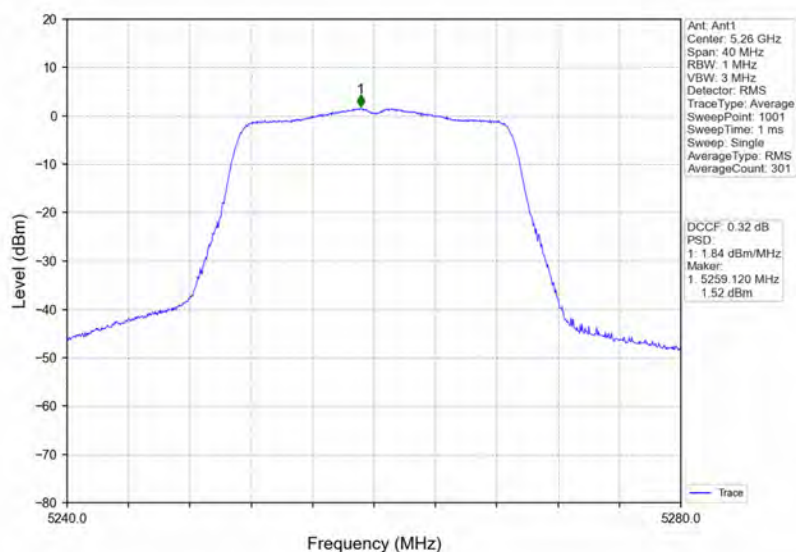
802.11n(HT20) LCH 5260MHz Ant1 NTN
