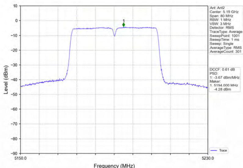
802.11ac(VHT40) LCH 5190MHz MIMO NTN
