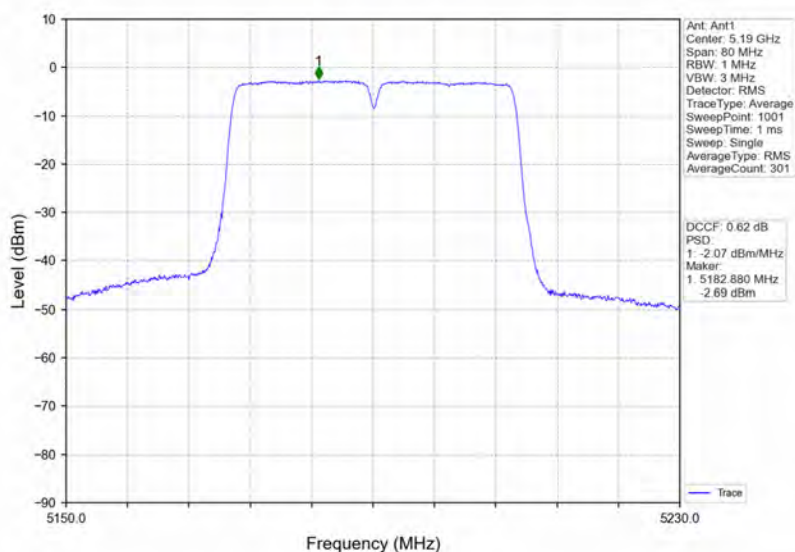
802.11n(HT40) LCH 5190MHz Ant1 NTN
