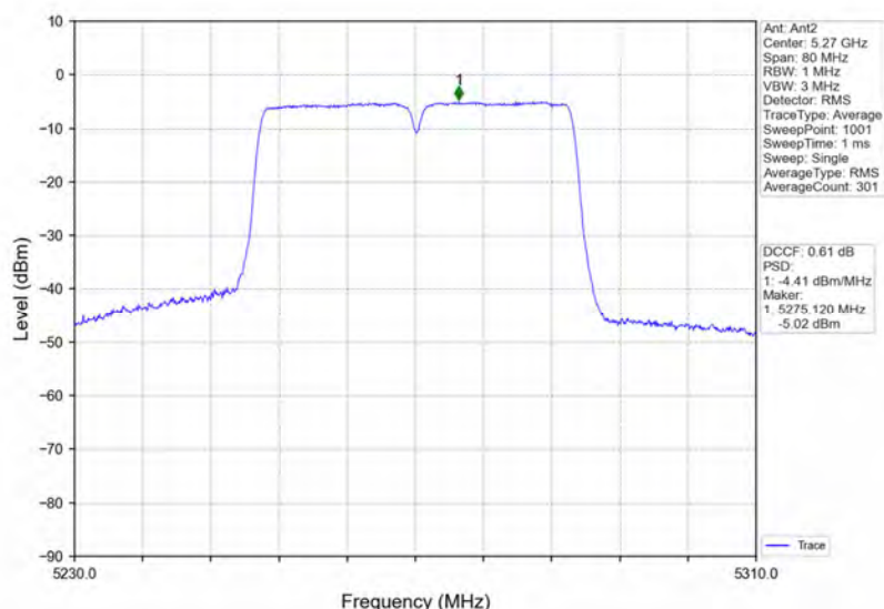
802.11ac(VHT40) LCH 5270MHz MIMO NTN
