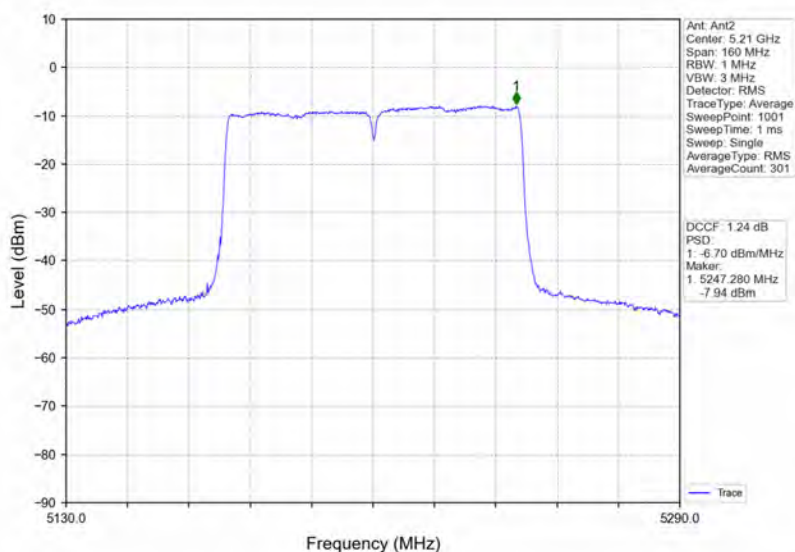
802.11ac(VHT80)_MCH_5210MHz_Ant2_NTNV
