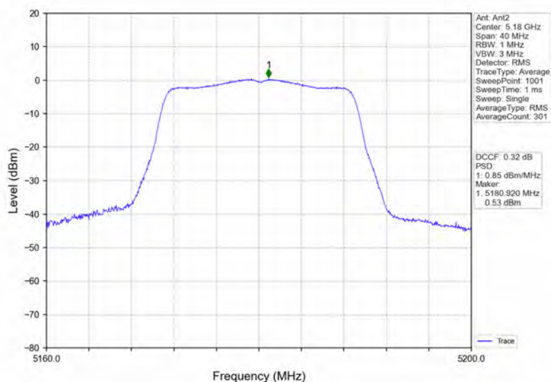
802.11ac(VHT20) LCH 5180MHz Ant2_NTNV
