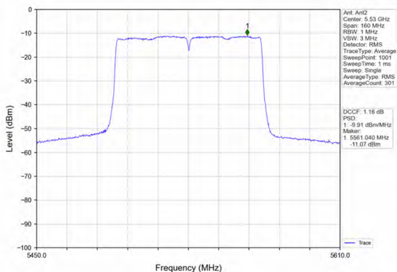
802.11ac(VHT80) LCH 5530MHz Ant2_NTNV
