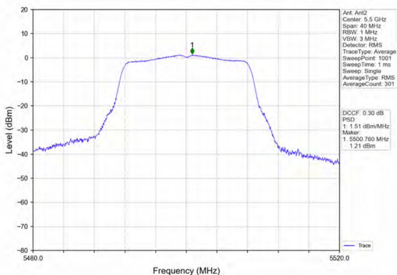
802.11a LCH_5500MHz_Ant2_NTNV
