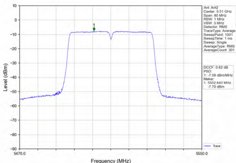
802.11n(HT40) LCH 5510MHz MIMO NTN
