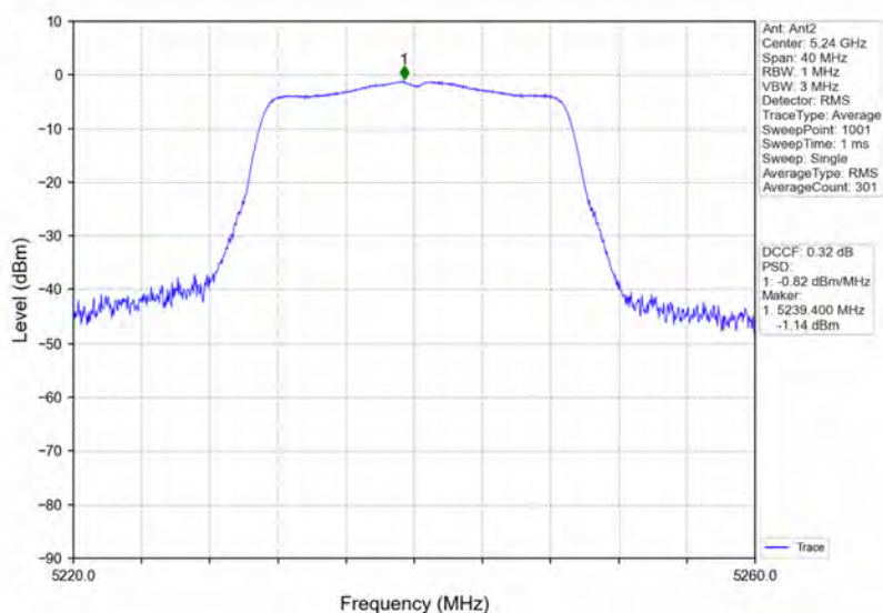
802.11n(HT20) HCH 5240MHz Ant2 NTN
