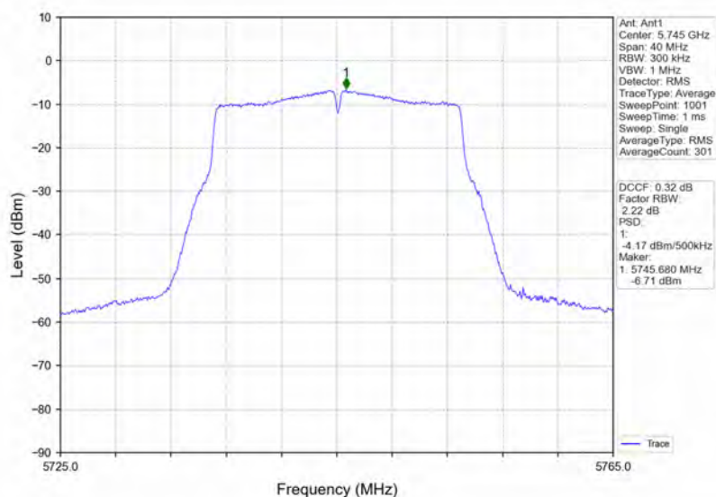
802.11ac(VHT20) LCH 5745MHz Ant1 NTN
