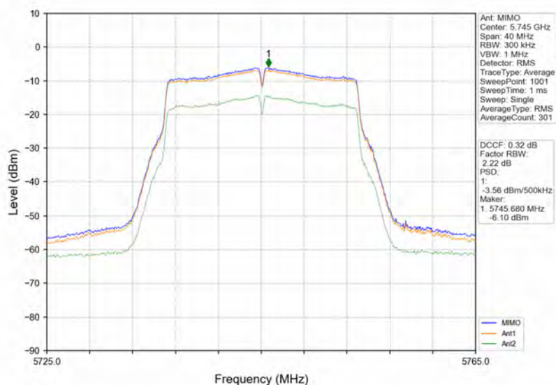
802.11ac(VHT20) LCH 5745MHz MIMO NTN
