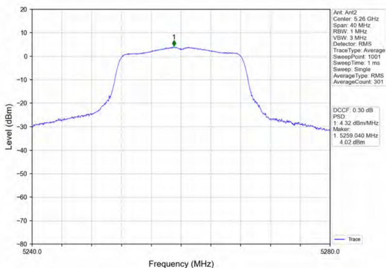
802.11a LCH_5260MHz_Ant2_NTNV
