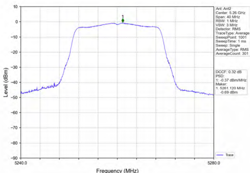
802.11n(HT20) LCH 5260MHz MIMO NTN
