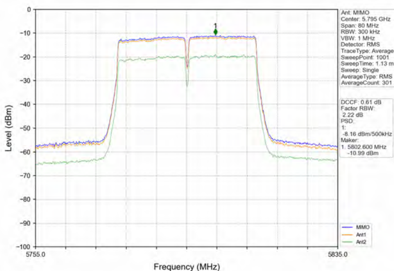
802.11ac(VHT40) HCH 5795MHz MIMO NTNV
