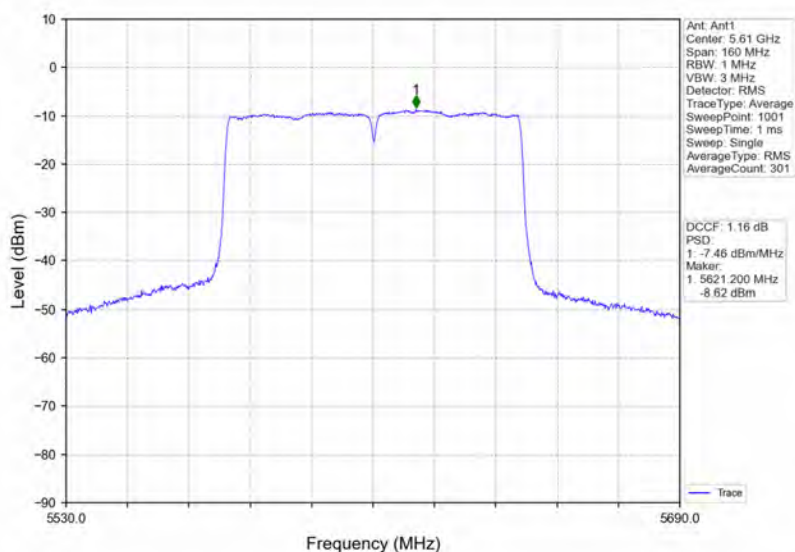
802.11ac(VHT80) HCH 5610MHz Ant1 NTN
