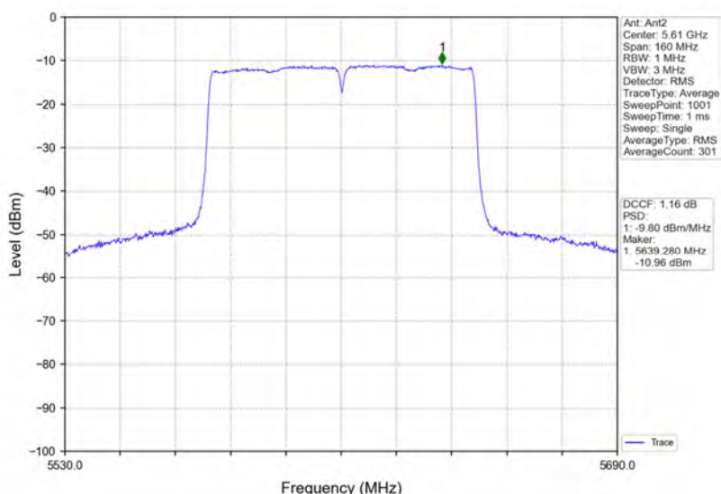
802.11ac(VHT80) HCH 5610MHz MIMO NTNV
