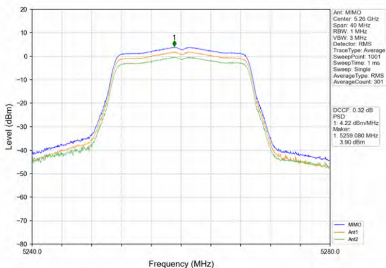
802.11ac(VHT20) LCH 5260MHz MIMO NTN
