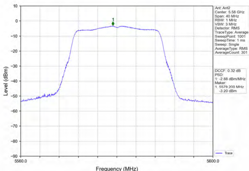
802.11n(HT20) MCH 5580MHz MIMO NTN
