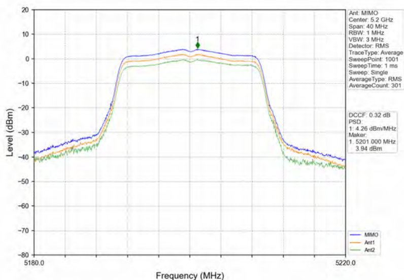
802.11n(HT20) MCH 5200MHz MIMO NTN
