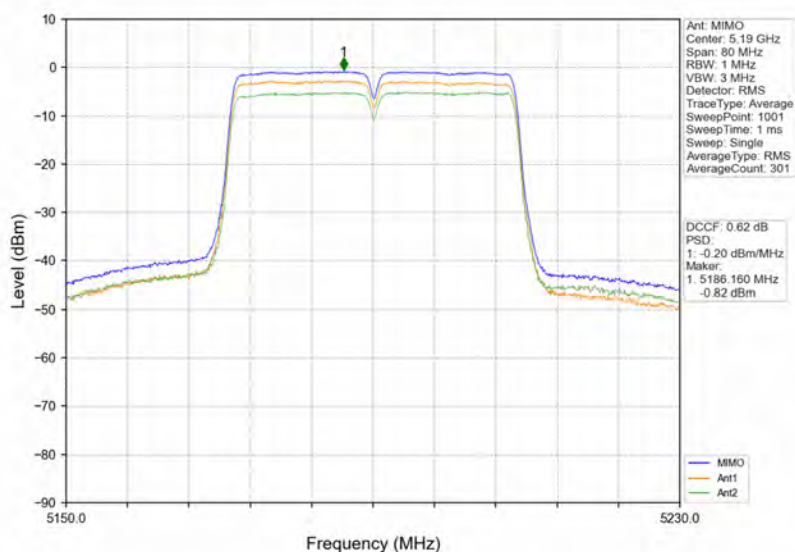
802.11n(HT40) LCH 5190MHz MIMO NTN
