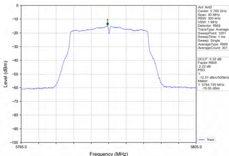
802.11n(HT20) MCH 5785MHz MIMO NTN
