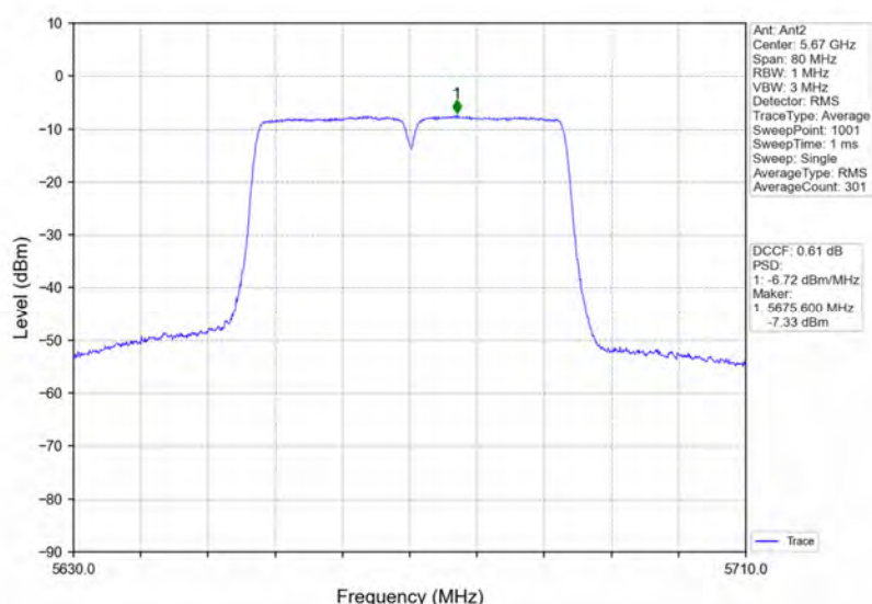
802.11ac(VHT40) HCH 5670MHz MIMO NTNV
