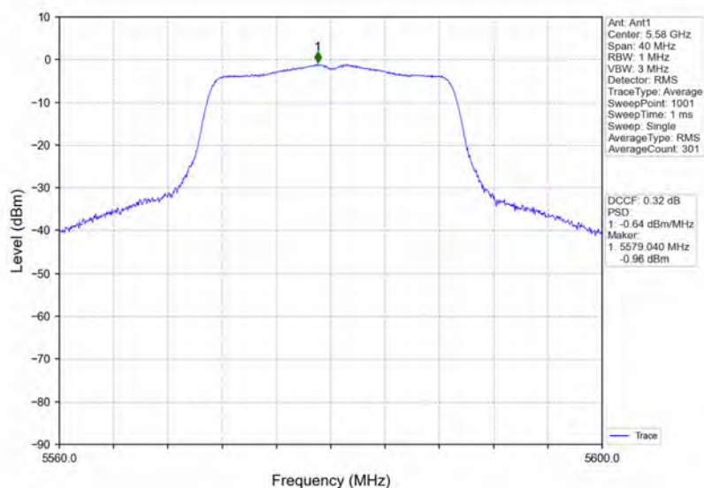
802.11n(HT20) MCH 5580MHz Ant1 NTN
