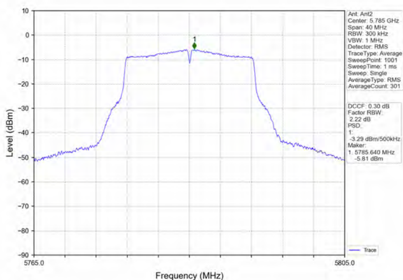
802.11a_MCH_5785MHz_Ant2_NTNV
