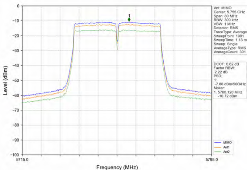
802.11n(HT40) LCH 5755MHz MIMO NTN
