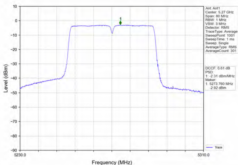
802.11ac(VHT40) LCH 5270MHz Ant1 NTNV
