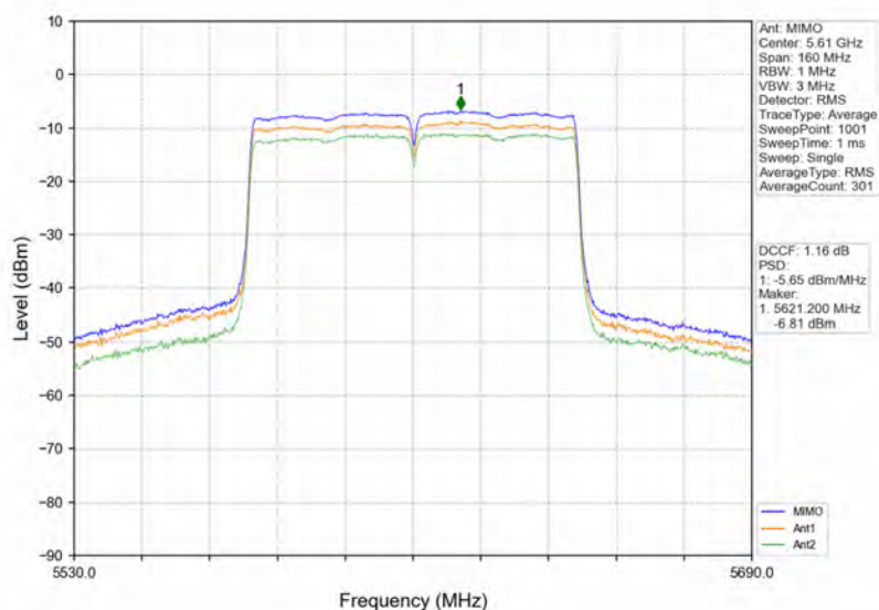
802.11ac(VHT80) HCH 5610MHz MIMO NTNV
