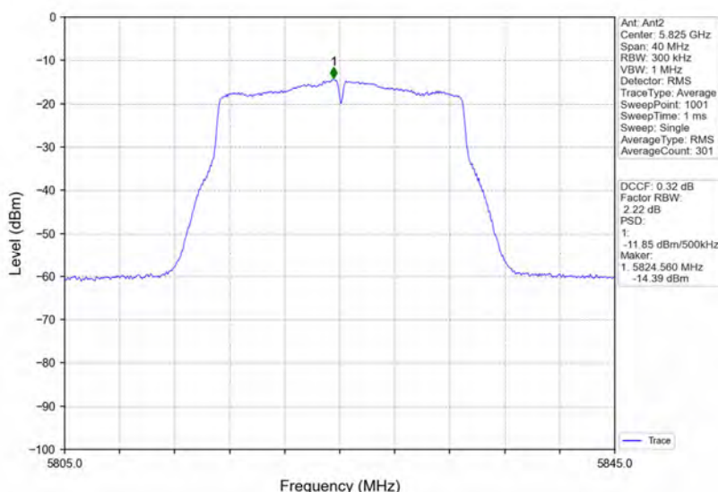
802.11ac(VHT20) HCH 5825MHz MIMO NTNV
