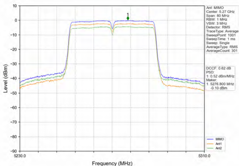
802.11n(HT40) LCH 5270MHz MIMO NTN
