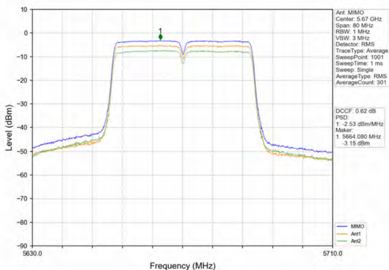
802.11n(HT40) HCH 5670MHz MIMO NTN
