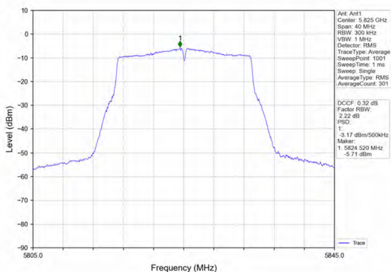
802.11ac(VHT20) HCH 5825MHz Ant1 NTNV
