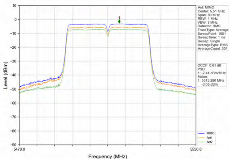
802.11ac(VHT40) LCH 5510MHz MIMO NTN
