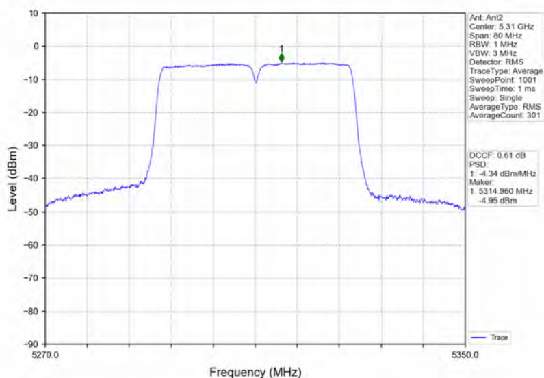
802.11ac(VHT40) HCH 5310MHz Ant2 NTNV
