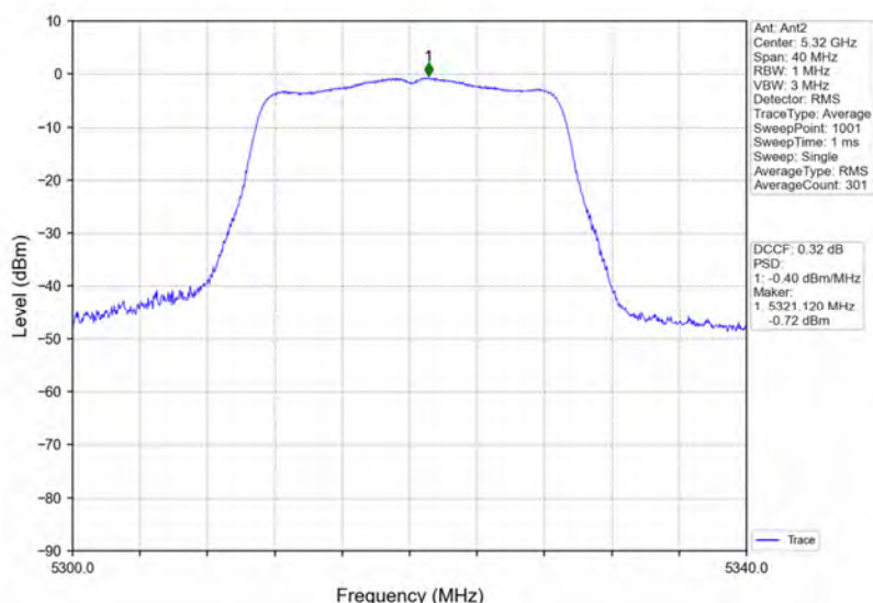
802.11n(HT20) HCH 5320MHz MIMO NTN
