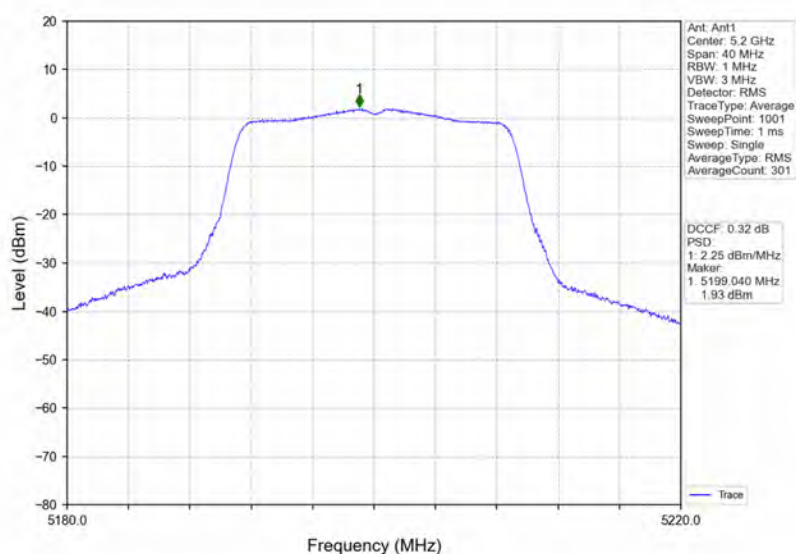
802.11ac(VHT20) MCH 5200MHz Ant1 NTN
