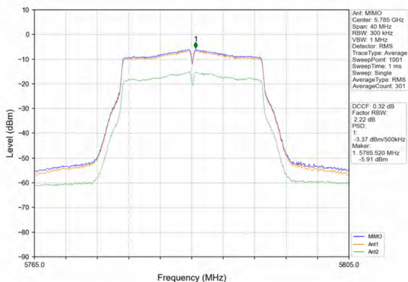
802.11n(HT20) MCH 5785MHz MIMO NTN
