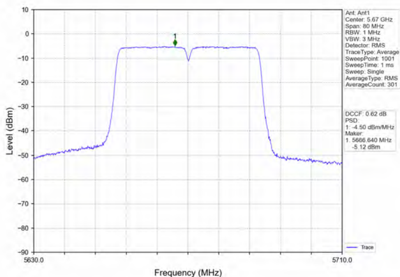
802.11n(HT40) HCH 5670MHz Ant1 NTN
