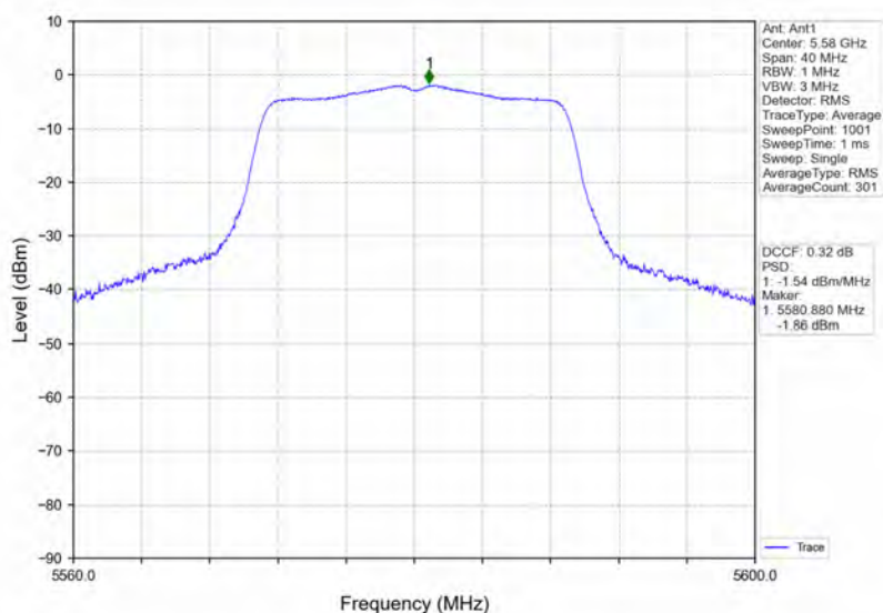
802.11ac(VHT20) MCH 5580MHz Ant1 NTN
