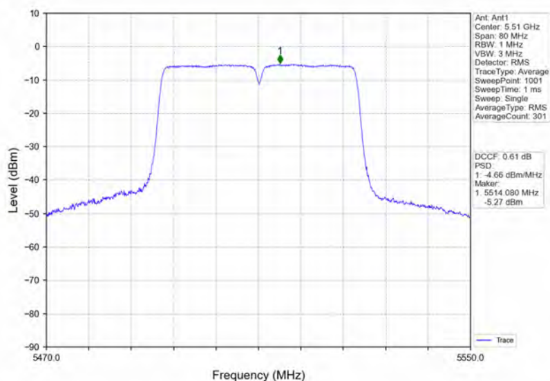
802.11ac(VHT40) LCH 5510MHz Ant1 NTNV
