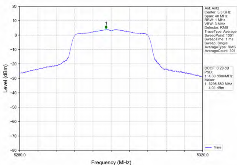
802.11a_MCH_5300MHz_Ant2_NTNV
