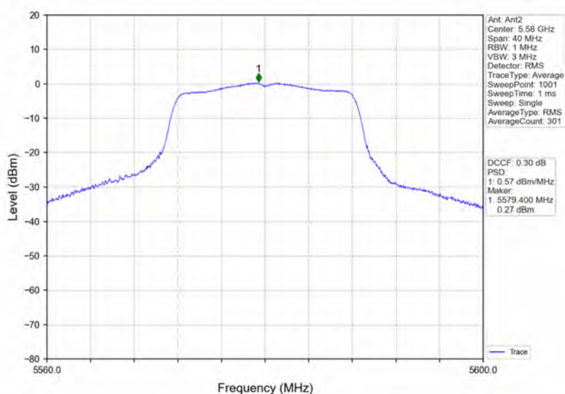
802.11a_MCH_5580MHz_Ant2_NTNV
