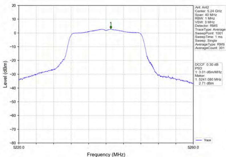
802.11a_HCH_5240MHz_Ant2_NTNV
