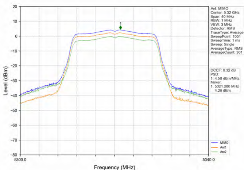
802.11ac(VHT20) HCH 5320MHz MIMO NTNV
