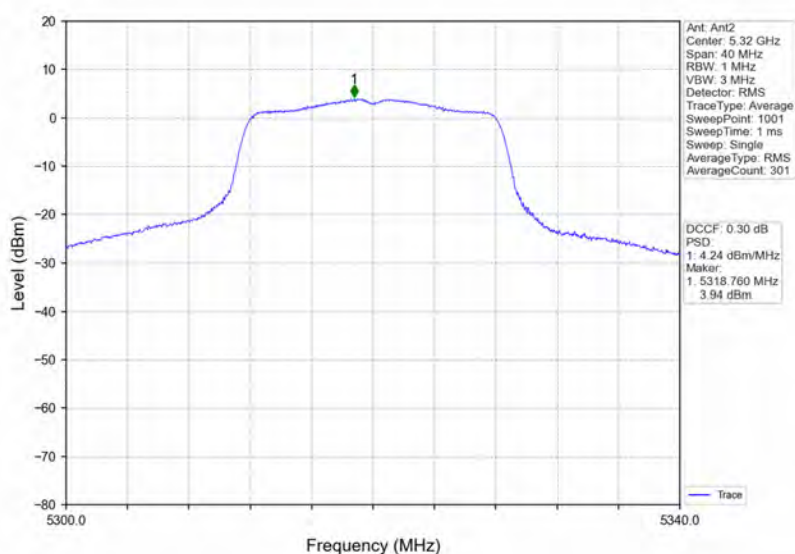
802.11a_HCH_5320MHz_Ant2_NTNV
