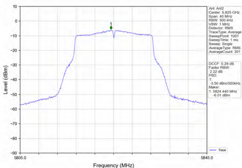
802.11a_HCH_5825MHz_Ant2_NTNV
