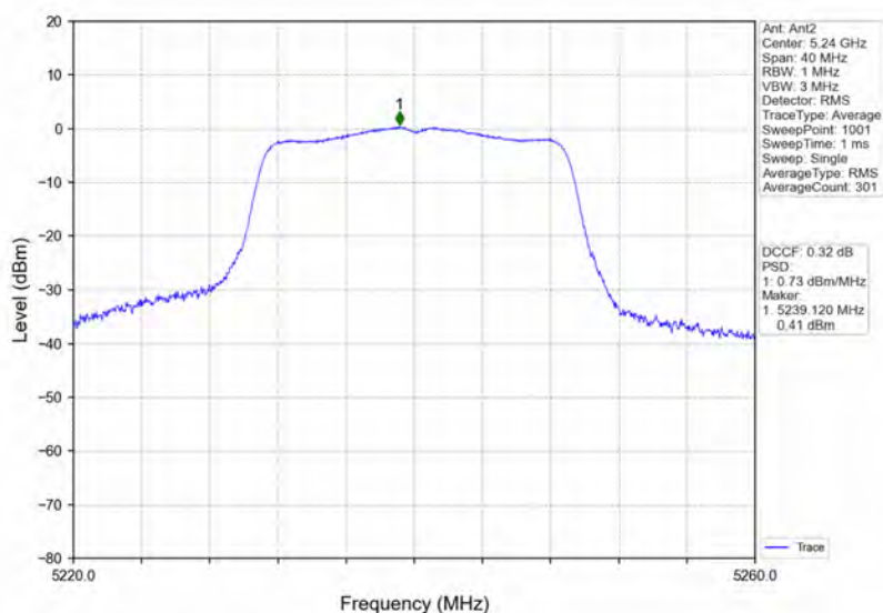
802.11ac(VHT20) HCH 5240MHz Ant2 NTNV
