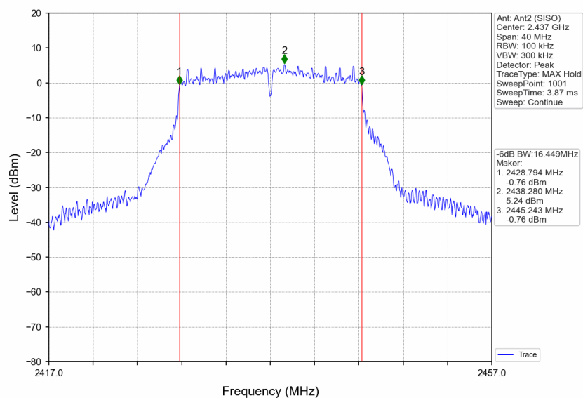
802.11g_MCH_2437MHz_Ant2 (SISO)_NTNV
