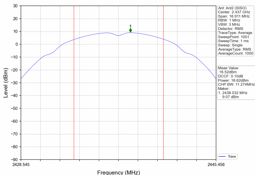
802.11b_MCH_2437MHz_Ant2 (SISO)_NTNV
