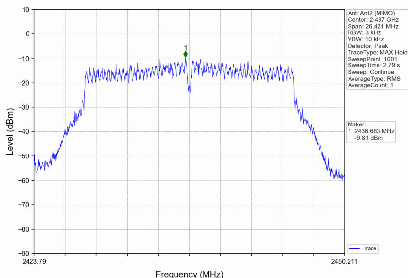
802.11n(HT20)_MCH_2437MHz_MIMO_NTNV
