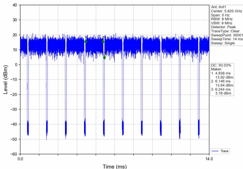
802.11n(HT20)_HCH_5825MHz_Ant1_NTNV
