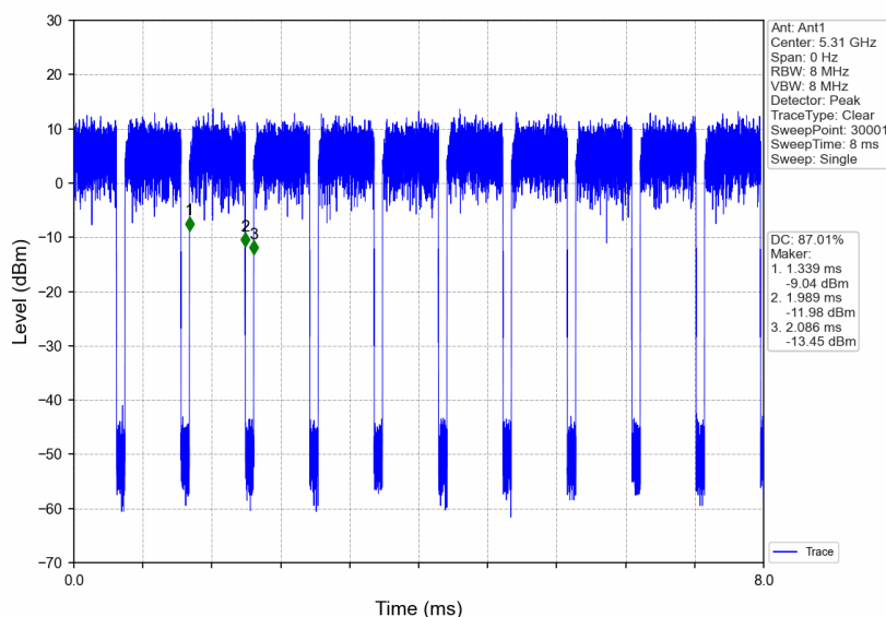
802.11n(HT40)_HCH_5310MHz_Ant1_NTNV
