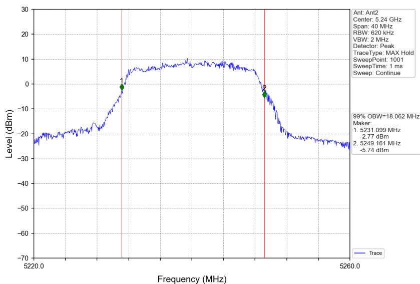
802.11a_HCH_5240MHz_Ant2_NTNV
