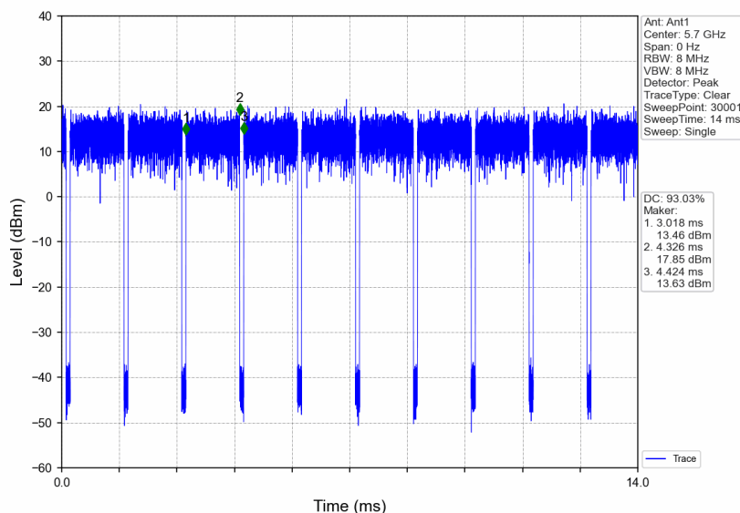
802.11n(HT20)_LCH_5745MHz_Ant1_NTNV
