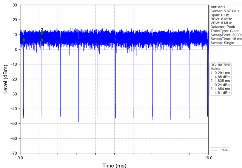
802.11ac(VHT40) HCH 5670MHz Ant1 NTV
