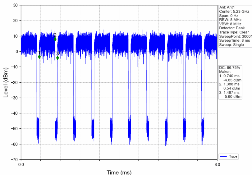
802.11n(HT40)_HCH_5230MHz_Ant1_NTNV
