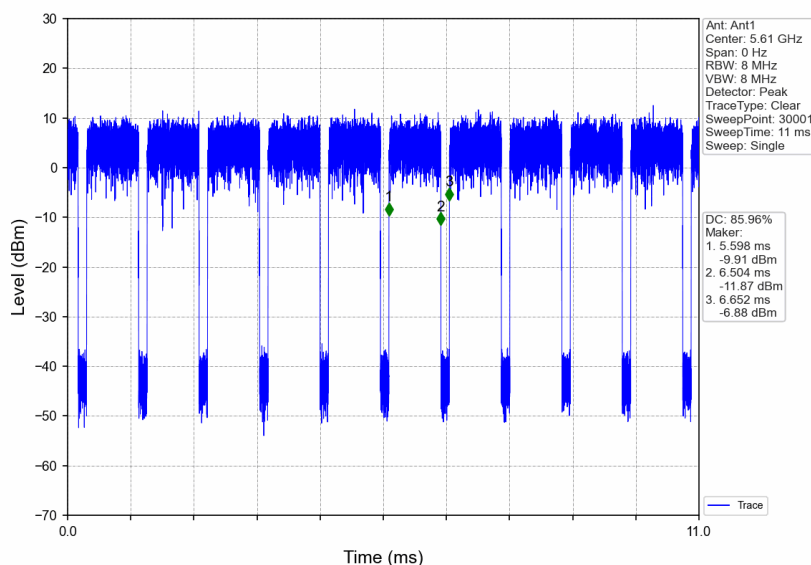
802.11ac(VHT80)_HCH_5610MHz_Ant1_NTNV
