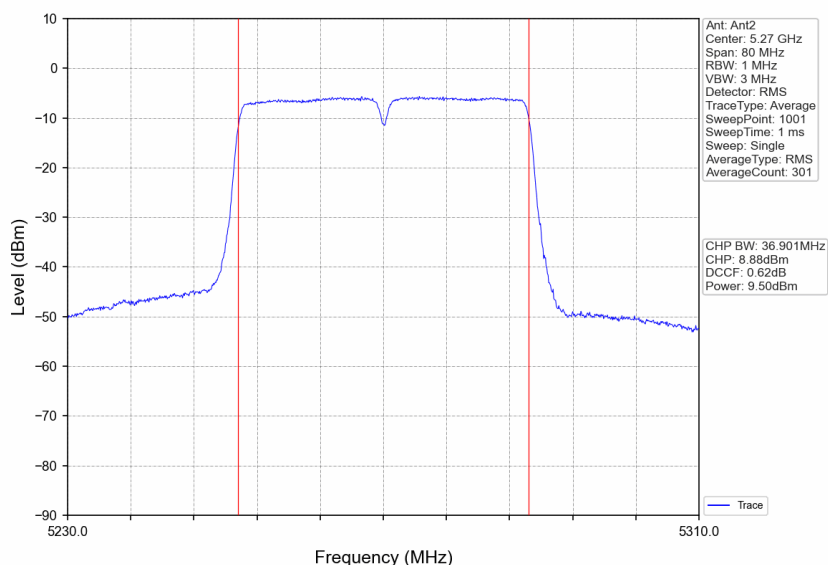
802.11n(HT40)_LCH_5270MHz_Ant2_NTNV
