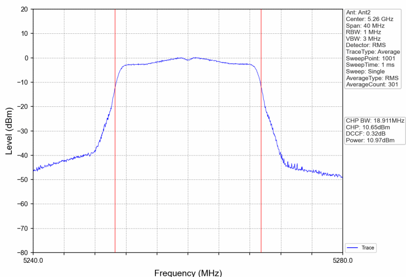
802.11n(HT20)_LCH_5260MHz_Ant2_NTNV
