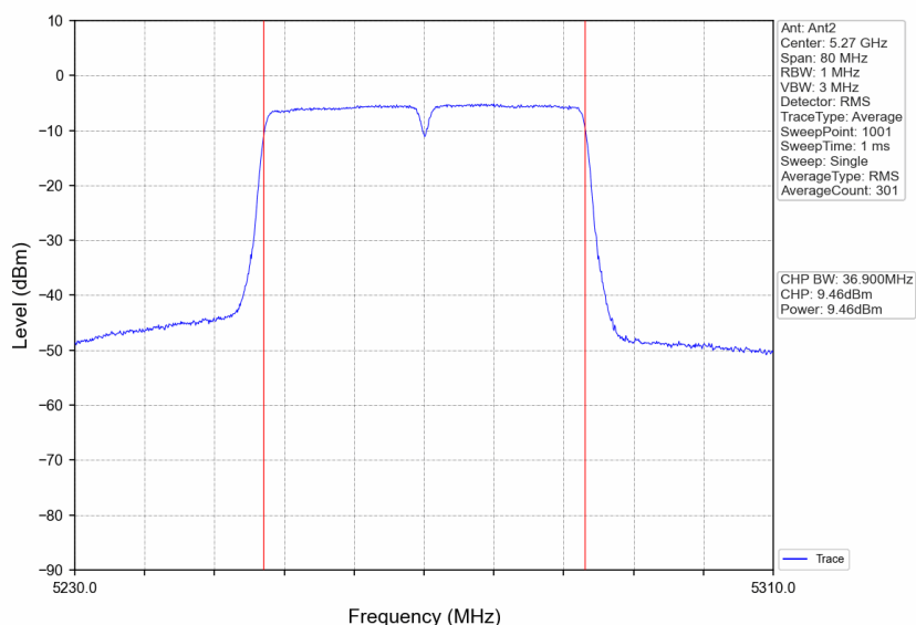
802.11ac(VHT40)_LCH_5270MHz_Ant2_NTNV
