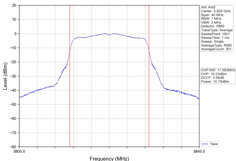
802.11a_HCH_5825MHz_Ant2_NTNV
