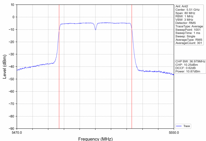
802.11n(HT40)_LCH_5510MHz_Ant2_NTNV
