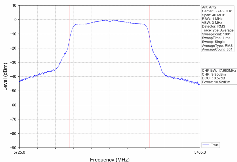
802.11a_LCH_5745MHz_Ant2_NTNV
