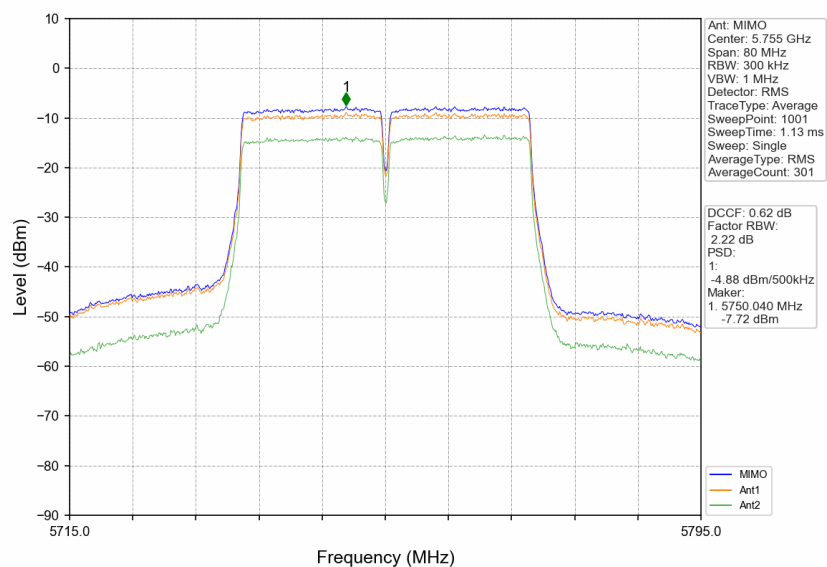
802.11n(HT40)_LCH_5755MHz_MIMO_NTNV
