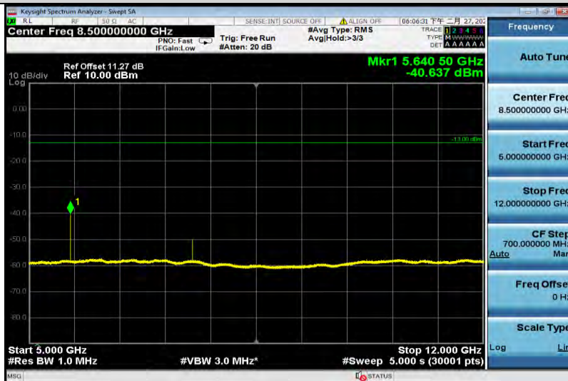
GPRS1900-661-5000~12000
