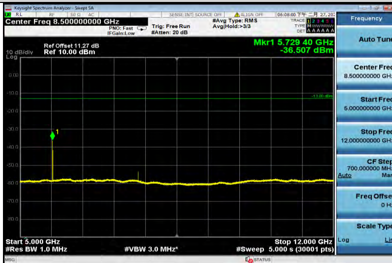
GPRS1900-810-5000~12000
