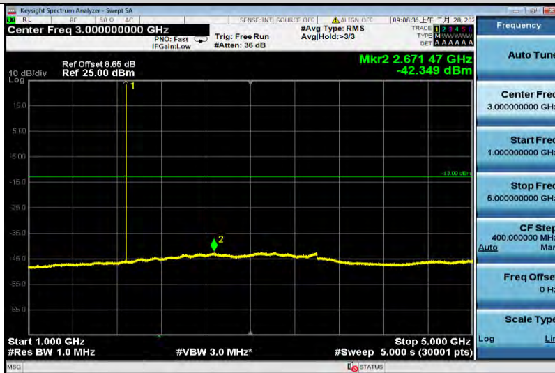
EGPRS1900-661-1000~5000
