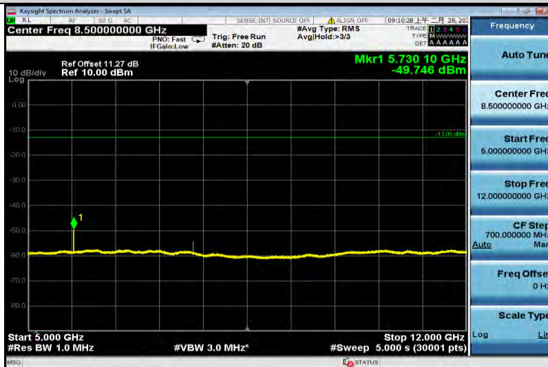
EGPRS1900-810-5000~12000
