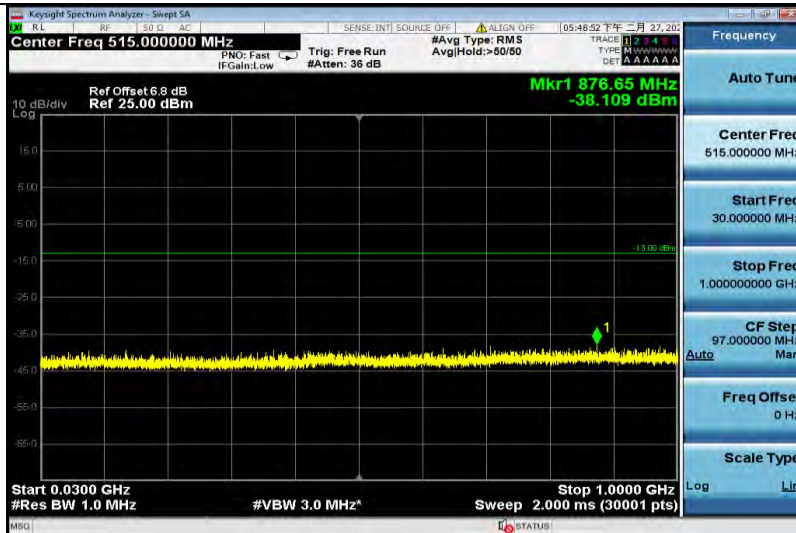
GSM1900-810-30~1000
