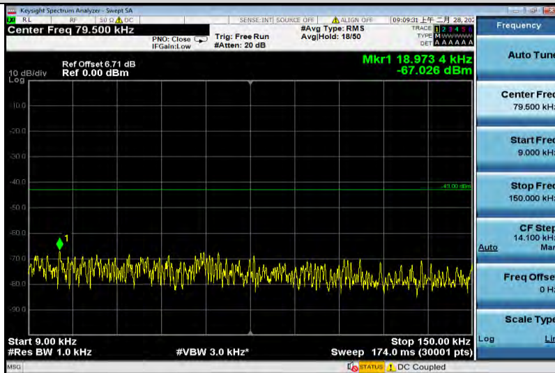
EGPRS1900-810-0.009~0.15
