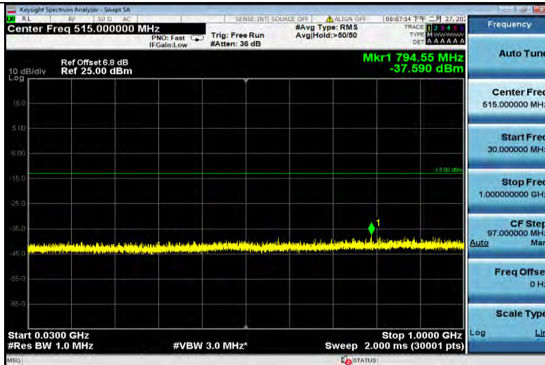
GPRS1900-810-30~1000
