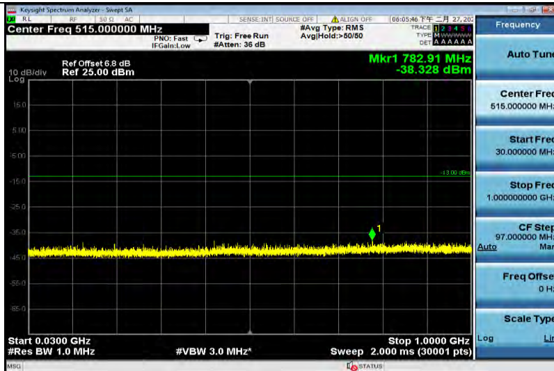
GPRS1900-661-30~1000
