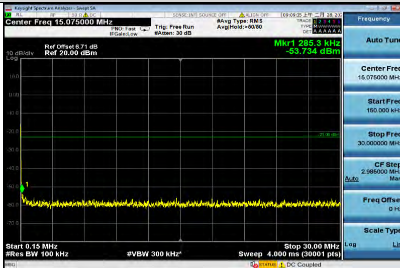
EGPRS1900-810-0.15~30
