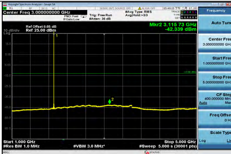
GSM1900-810-1000~5000
