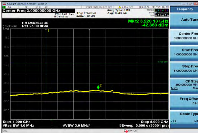
EGPRS1900-810-1000~5000
