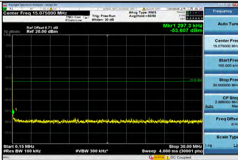
EGPRS1900-661-0.15~30
