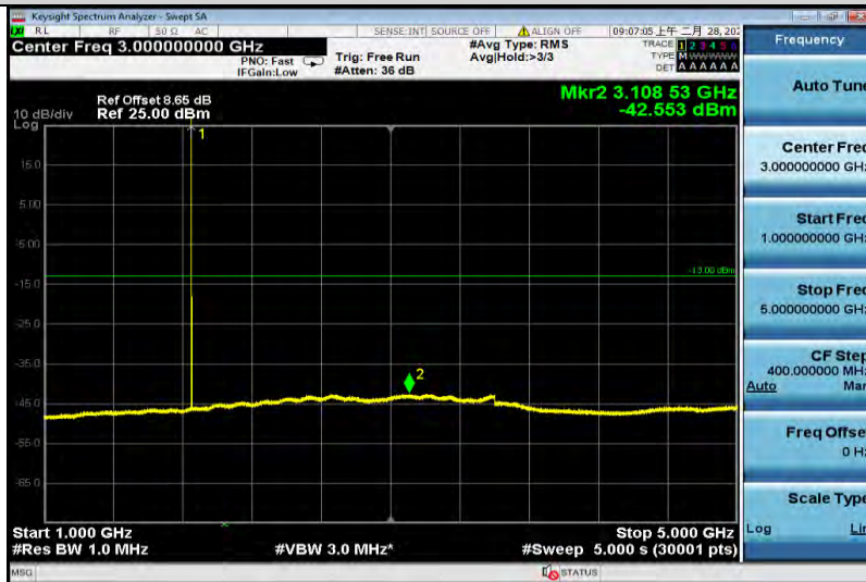
EGPRS1900-512-1000~5000
