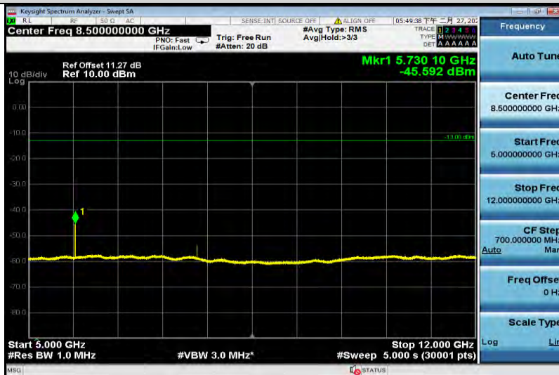
GSM1900-810-5000~12000
