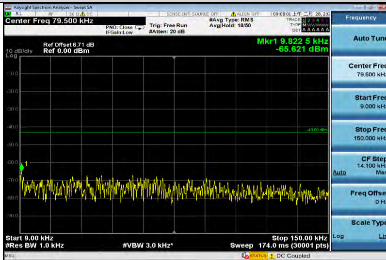
EGPRS1900-661-0.009~0.15
