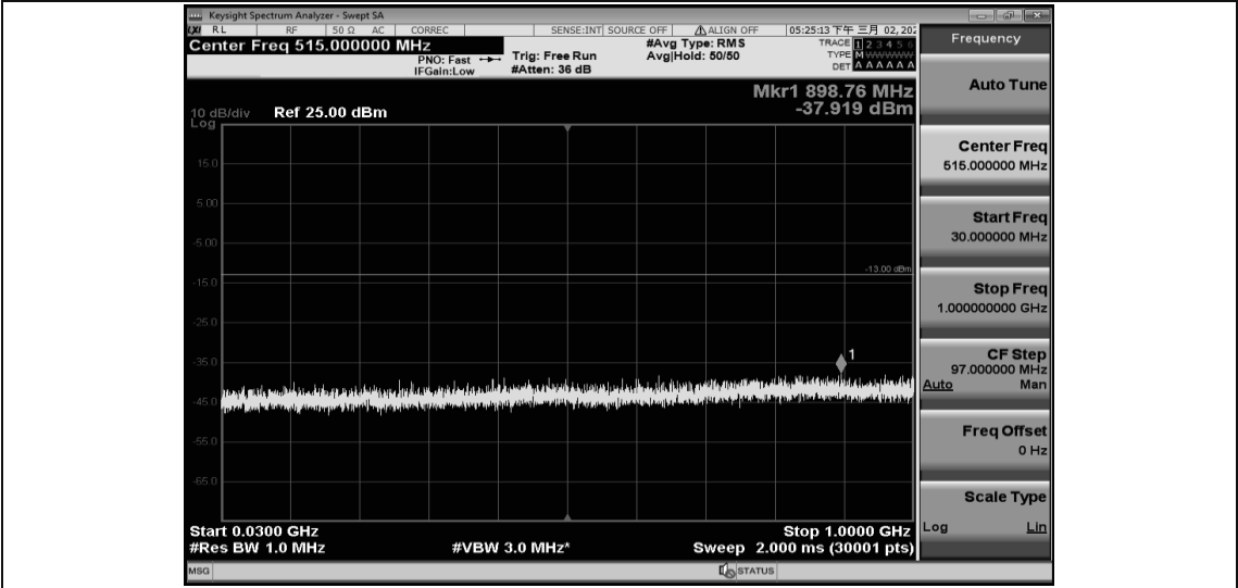
Band25-3MHz-16QAM-26055-1RB#0-Range2:1000~5000MHz
