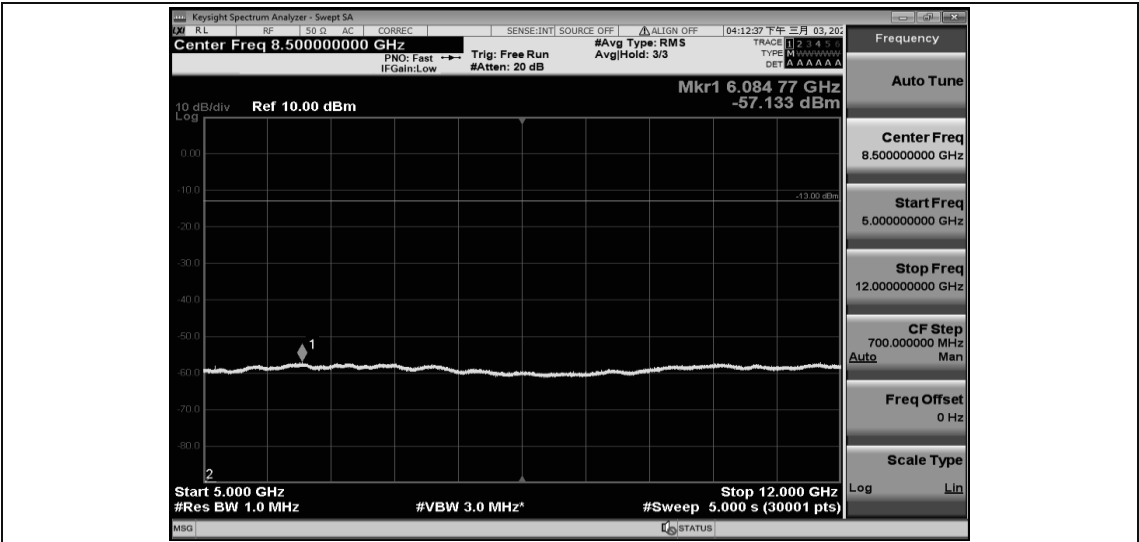
Band66-10MHz-QPSK-132022-1RB#0-Range4:12000~26500MHz
