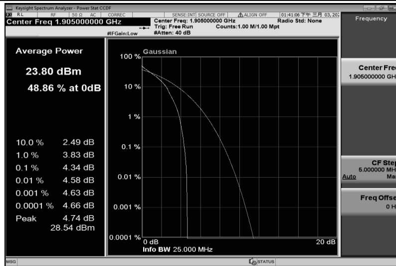
Band25-20MHz-QPSK-26590-100RB#0
