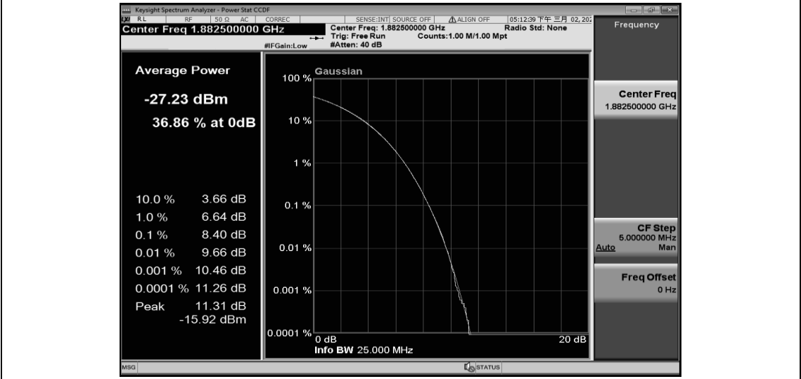
Band25-1.4MHz-QPSK-26365-6RB#0
