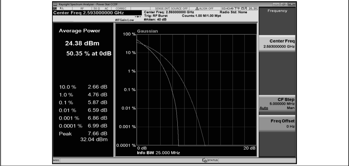
Band41-20MHz-QPSK-41490-1RB#0
