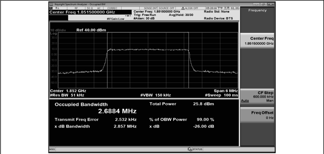
Band25-3MHz-QPSK-26365-15RB#0-2.6896
