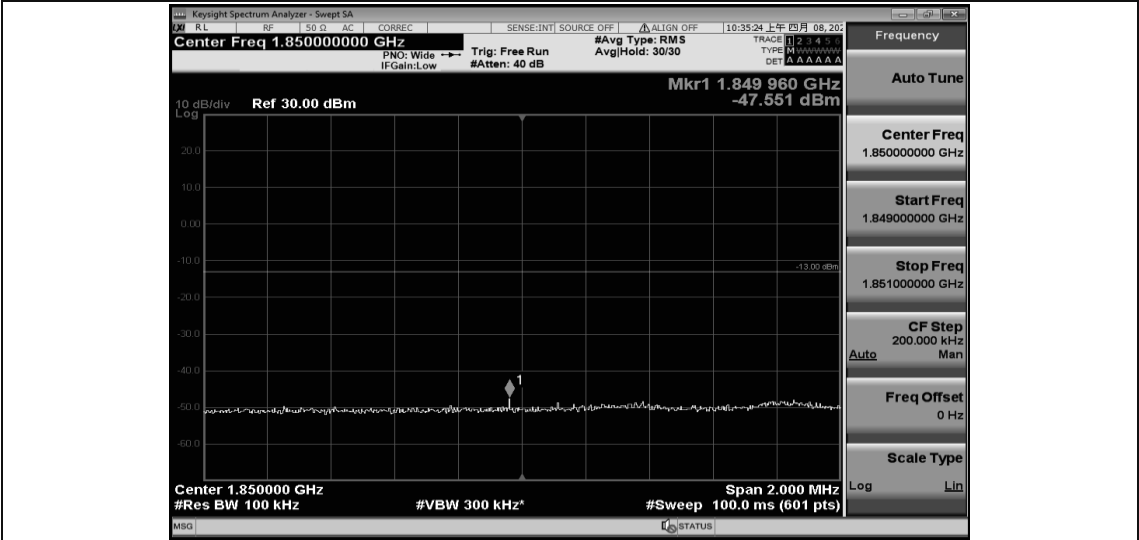
Band2-5MHz-16QAM-18625-1RB#0
