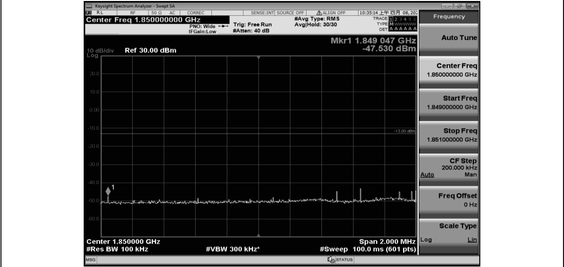
Band2-5MHz-QPSK-18625-25RB#0
