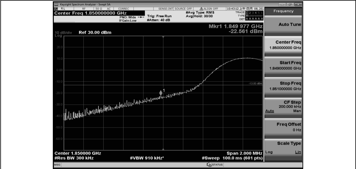
Band2-15MHz-QPSK-18675-1RB#74
