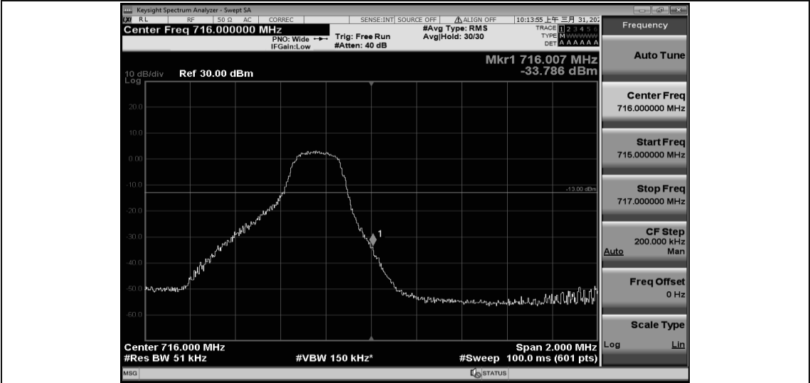
Band12-3MHz-QPSK-23165-15RB#0
