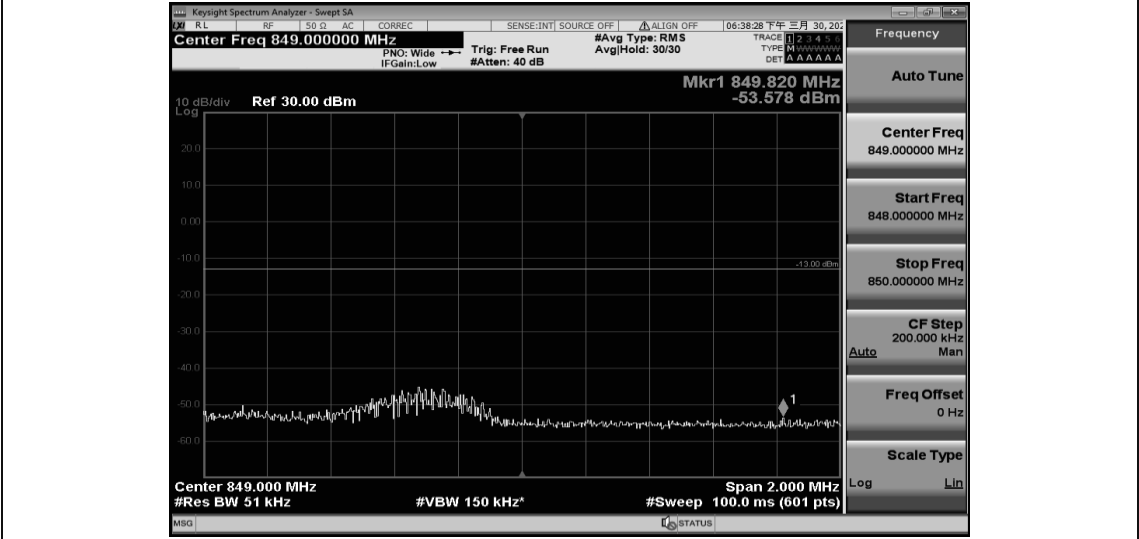
Band5-3MHz-QPSK-20635-15RB#0
