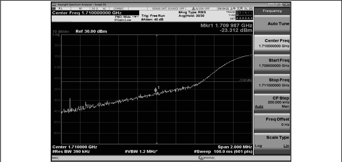
Band66-20MHz-QPSK-132072-1RB#99
