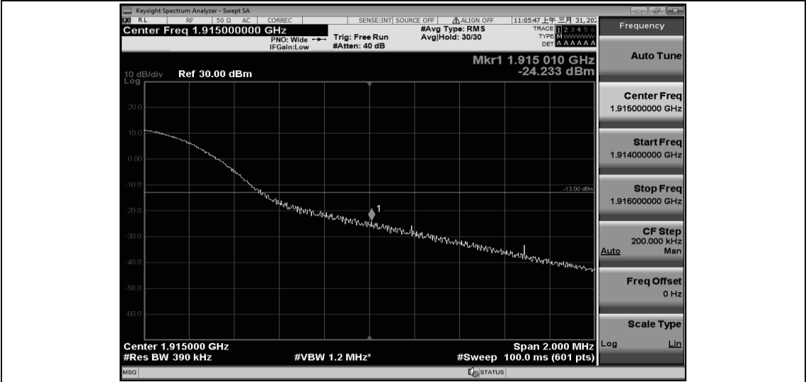
Band25-20MHz-QPSK-26590-1RB#0
