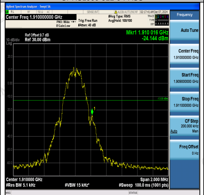
GPRS1900-810-0-PASS
