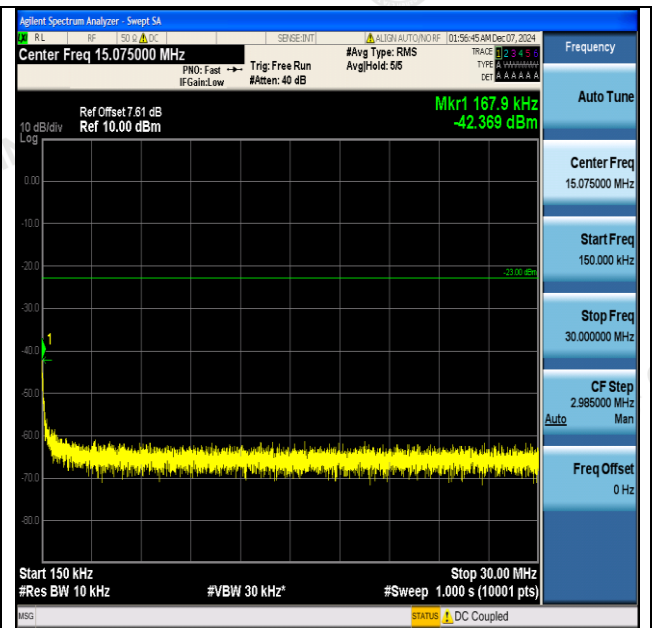
GPRS850-128-5-0.15~30MHz-PASS
