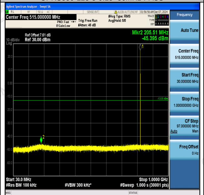
GPRS850-128-5-30~1000MHz-PASS
