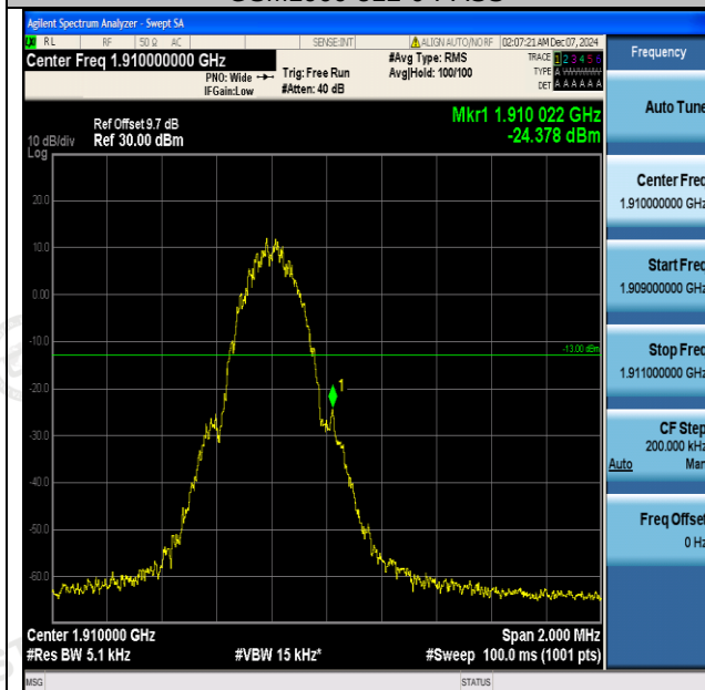
GSM1900-810-0-PASS
