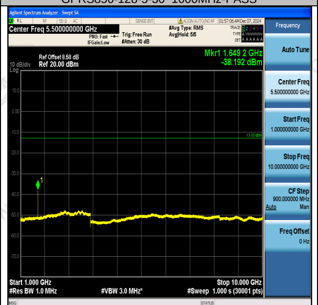
GPRS850-128-5-1000~10000MHz-PASS
