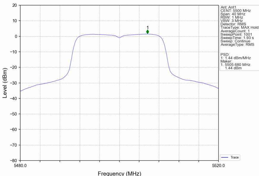
802.11n(HT20)_LCH_5500MHz_Ant1_NTNV
